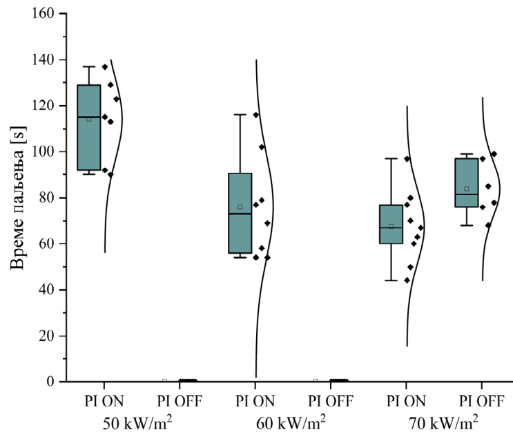
Слика 4.2. Време паљења узорака за различите топлотне флуксеве и типове паљења
