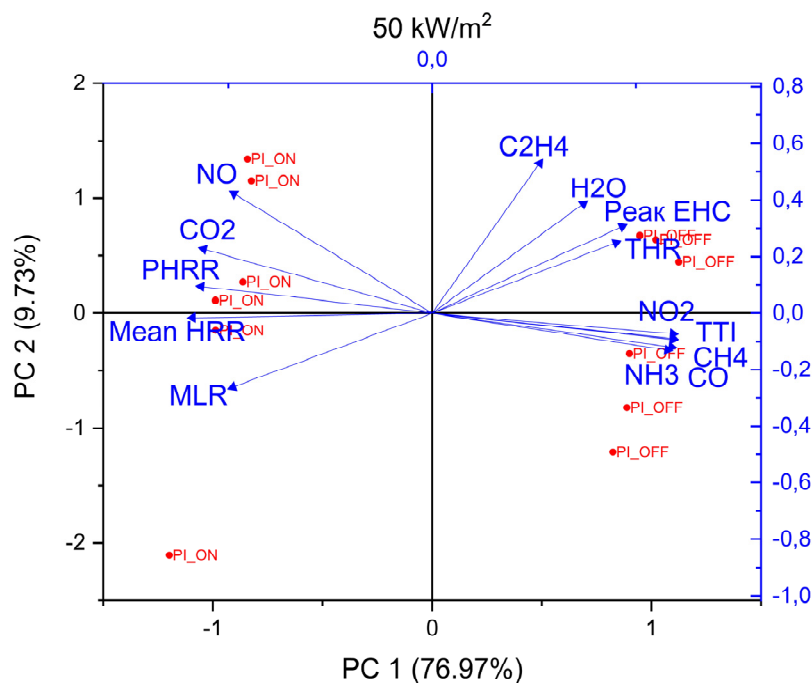
Слика 4.8. Биplot приказ корелације параметара запаљивости и продуката сагоревања у зависности од типа паљења на топлотном флукусу од 50 kW/m 2
