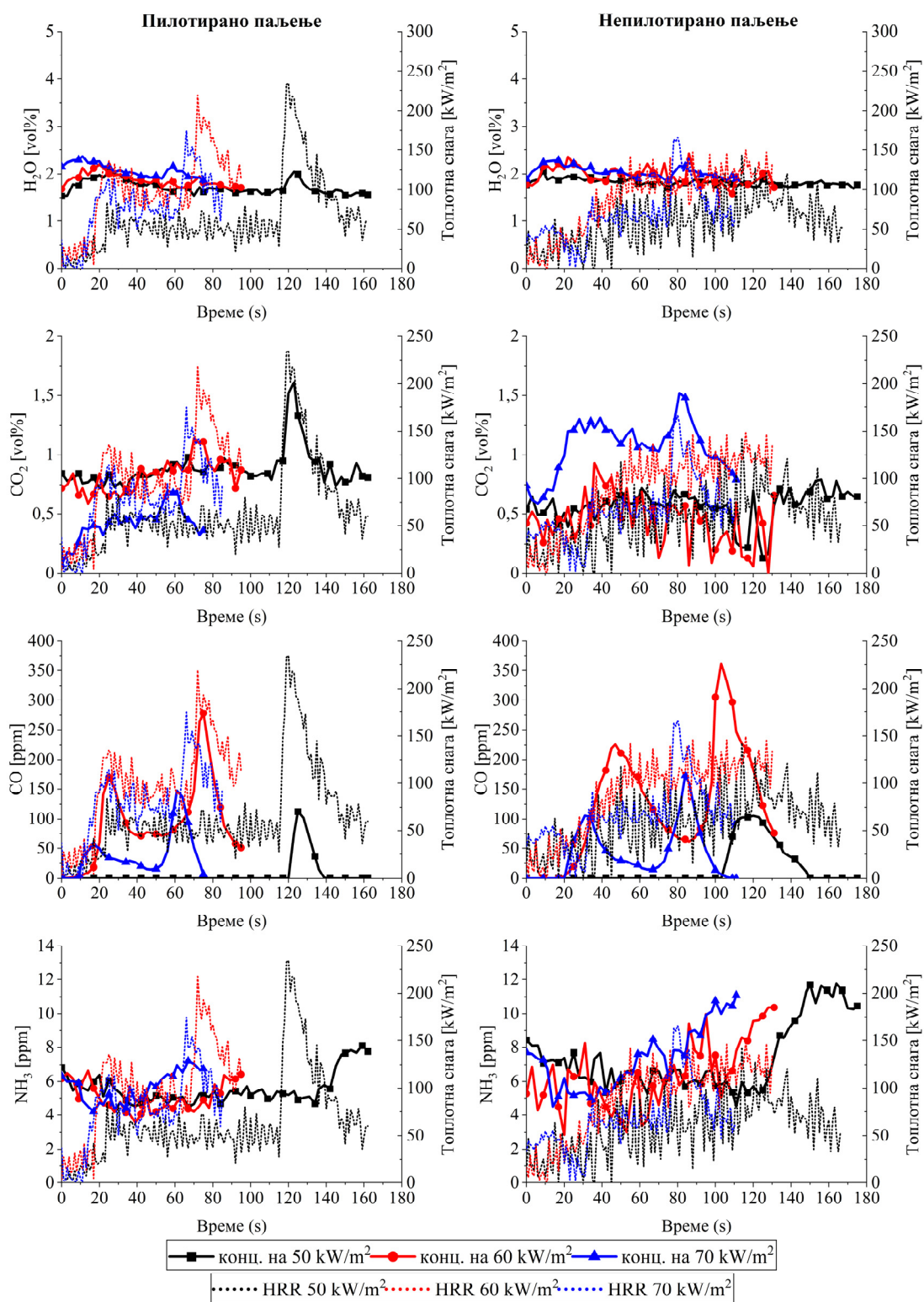
Слика 4.7. Концентрације доминантних продуката сагоревања у функцији времена, за различите типове паљења, при излагању топлотним флукевима од 50, 60 и 70\text{ kW/m}^2
