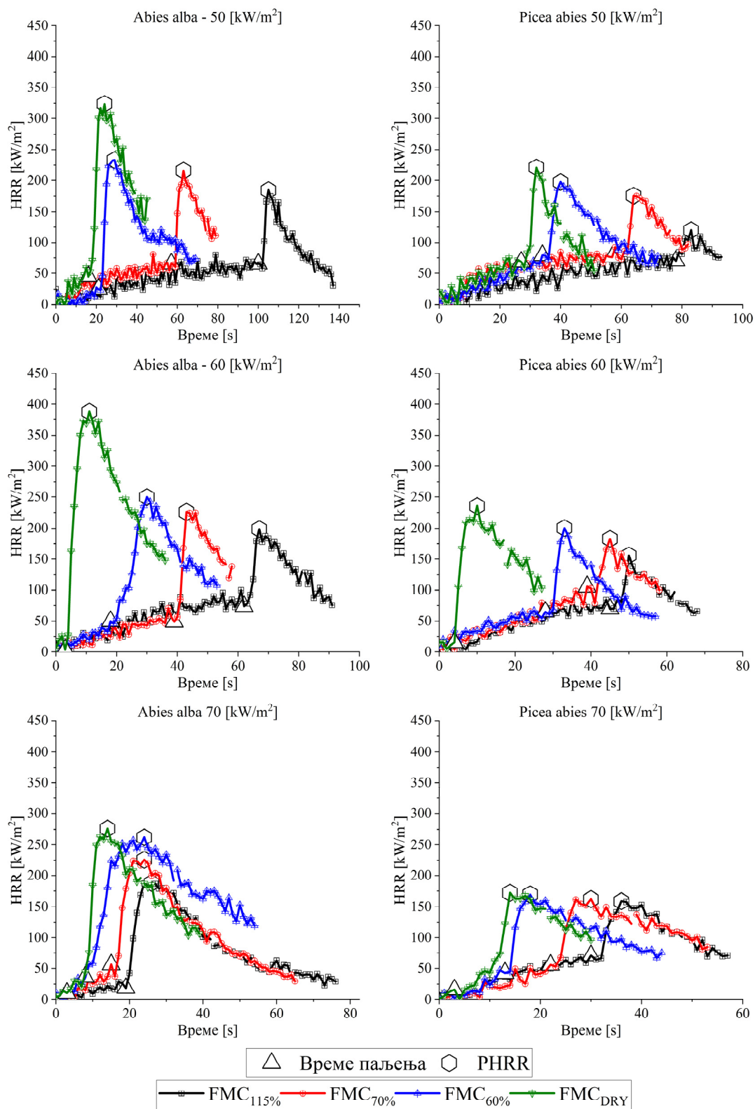
Слика 3.5. Графикон развоја топлотне снаге за различите вредности садржаја воде и топлотних флукса за анализиране четинарске врсте
