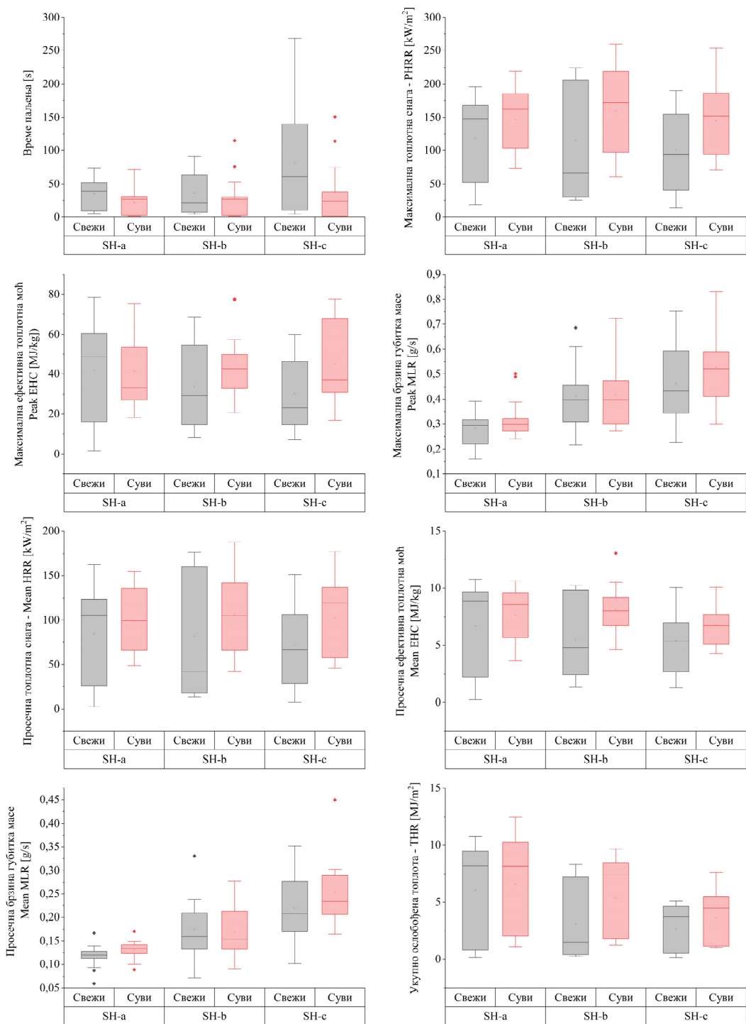
Слика 6.2. Средње вредност параметара запаљивости по типу носача узорка и нивоа влажности узорка
