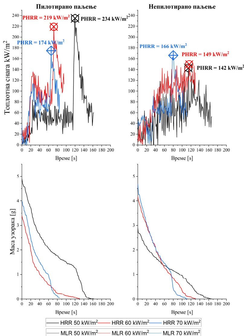
Слика 4.3. Графички приказ развоја топлотне снаге ( HRR ) и брзине губитка масе за пилотирано и непилотирано паљење при излагању топлотном флуксу од 50, 60 и 70 kW/m 2
