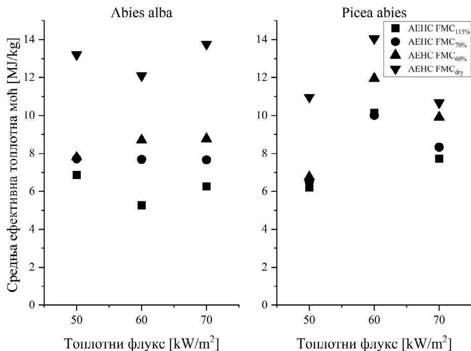
Слика 3.7. Средња ефективна топлотна моћ за различите вредности садржаја влаге и топлотних флуксева за анализирани четиначне врсте
