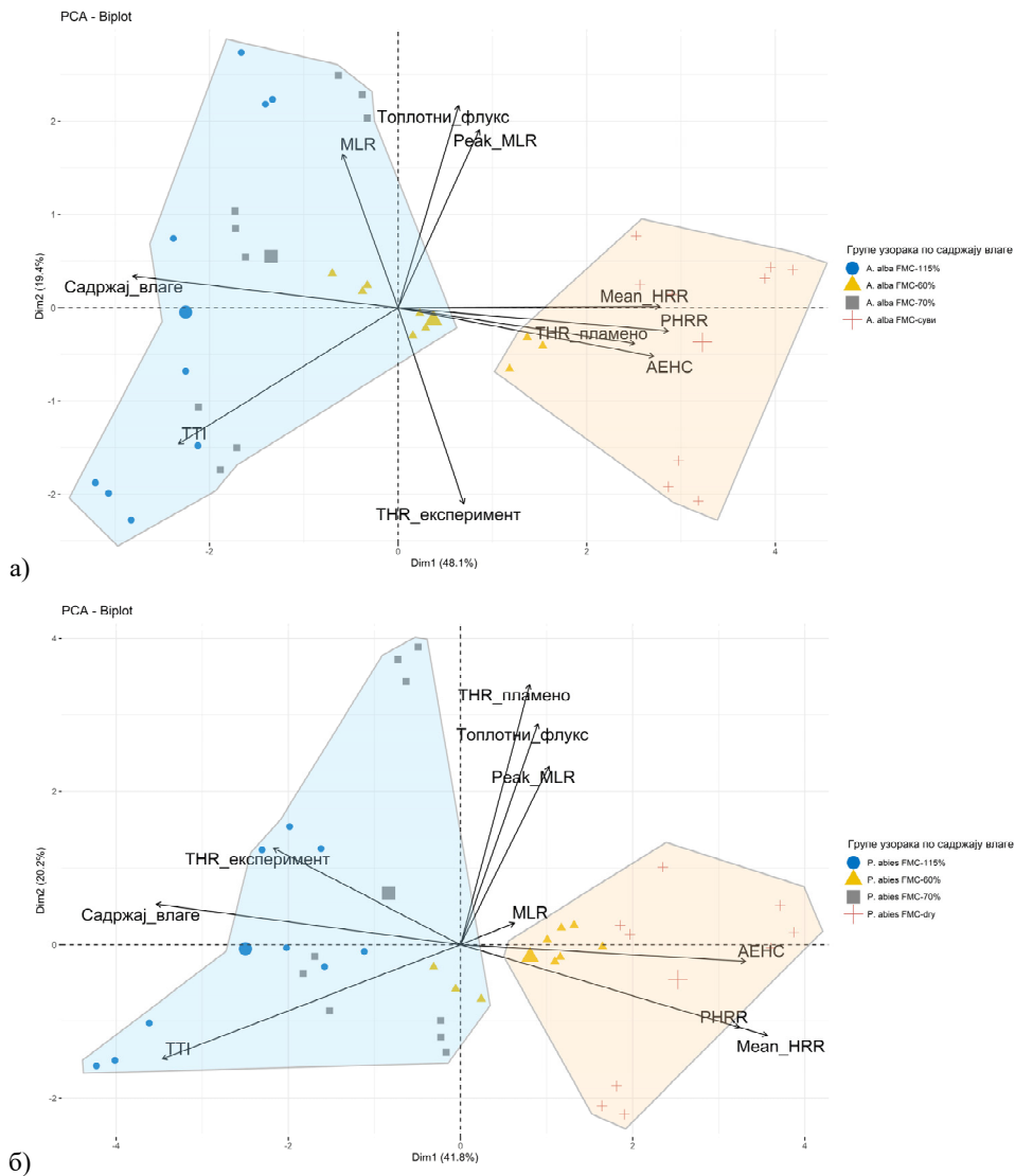
Слика 3.10. Биplot PCA анализе за параметре запаљивости у односу на различите топлотне флуksеве и садржај влага за узорке (а) A. alba и (б) P. abies
