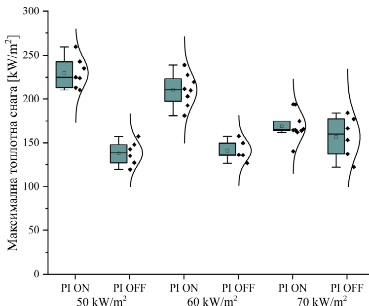
Слика 4.4. Максимальна топлотна снага за различите нивое топлотног флуksа и типа паљења
