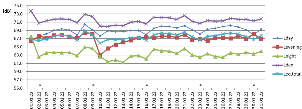
Sl. 2 Promene dnevnih vrednosti indikatora buke u toku januara 2022. za NMT-2
