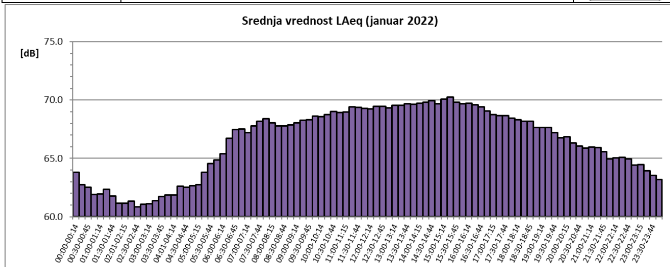
Sl. 6 Promene usrednjenih petnaestominutnih vrednosti ekvivalentnog nivoa buke u toku januara 2022. za NMT-2
