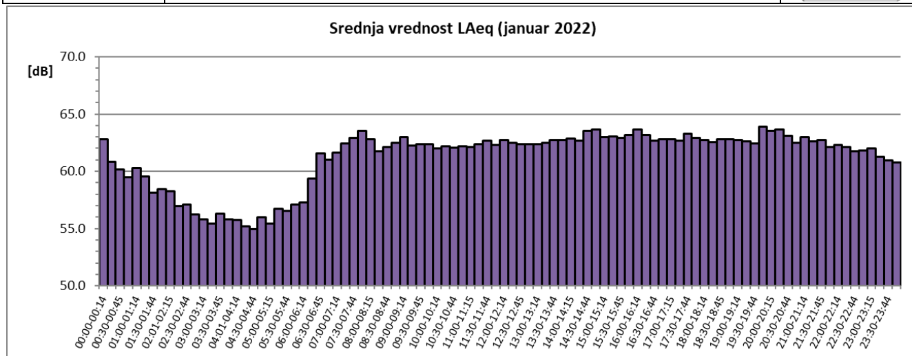
Sl. 5 Promene usrednjenih petnaestominutnih vrednosti ekvivalentnog nivoa buke u toku januara 2022. za NMT-1
