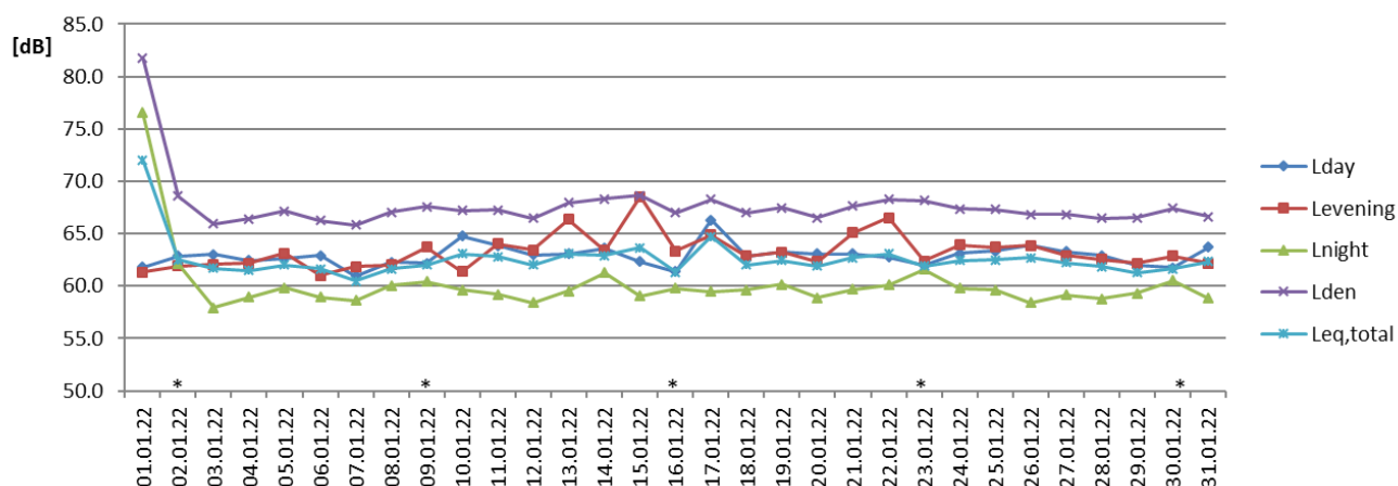
Sl. 1 Promene dnevnih vrednosti indikatora buke u toku januara 2022. za NMT-1
