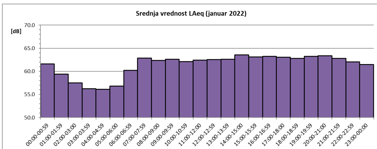
Sl. 3 Promene usrednjenih časovnih vrednosti ekvivalentnog nivoa buke u toku januara 2022. za NMT-1
