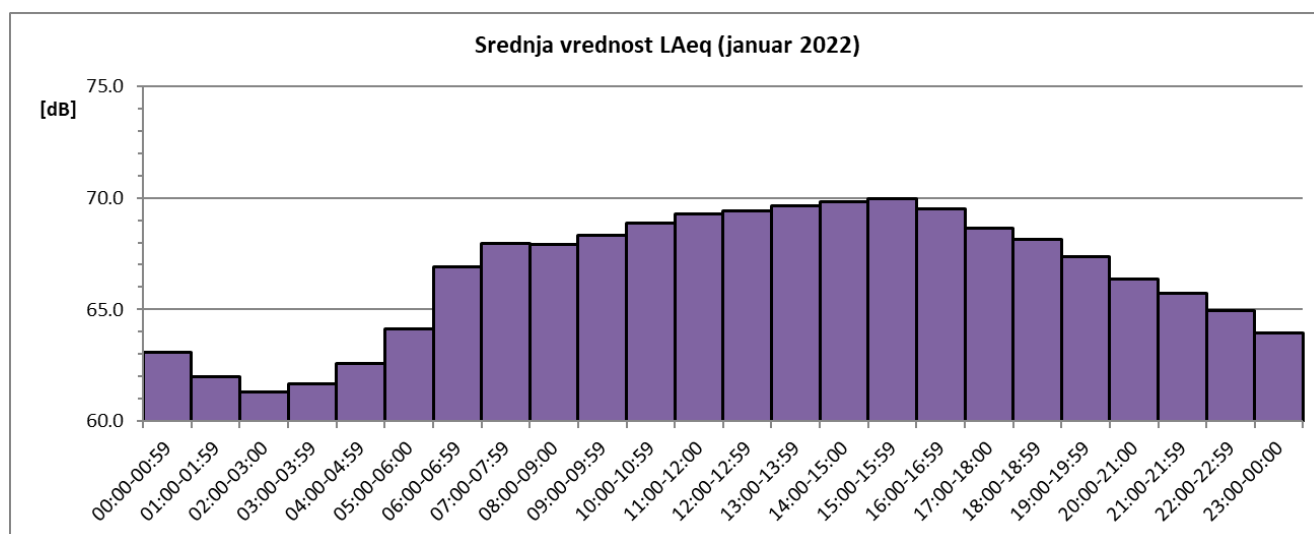
Sl. 4 Promene usrednjenih časovnih vrednosti ekvivalentnog nivoa buke u toku januara 2022. za NMT-2
