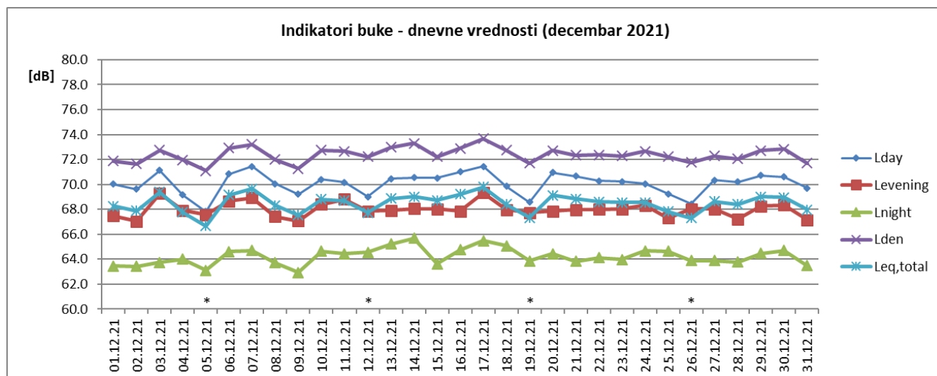
Sl. 2 Promene dnevnih vrednosti indikatora buke u toku decembra 2021. za NMT-2
