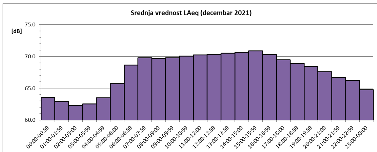
Sl. 4 Promene usrednjenih časovnih vrednosti ekvivalentnog nivoa buke u toku decembra 2021. za NMT-2
