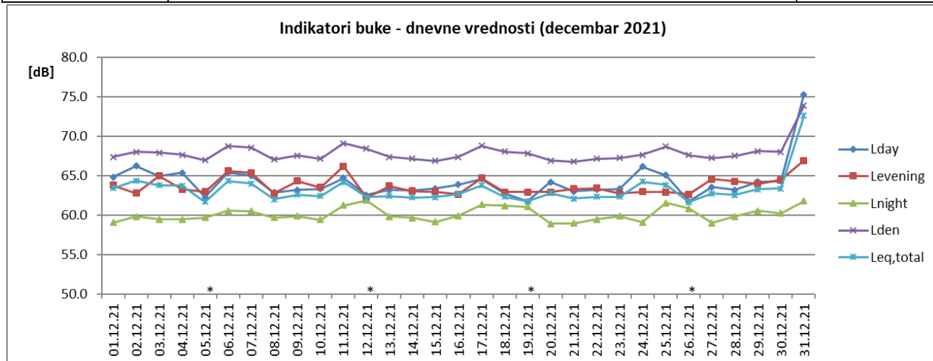
Sl. 1 Promene dnevnih vrednosti indikatora buke u toku decembra 2021. za NMT-1
