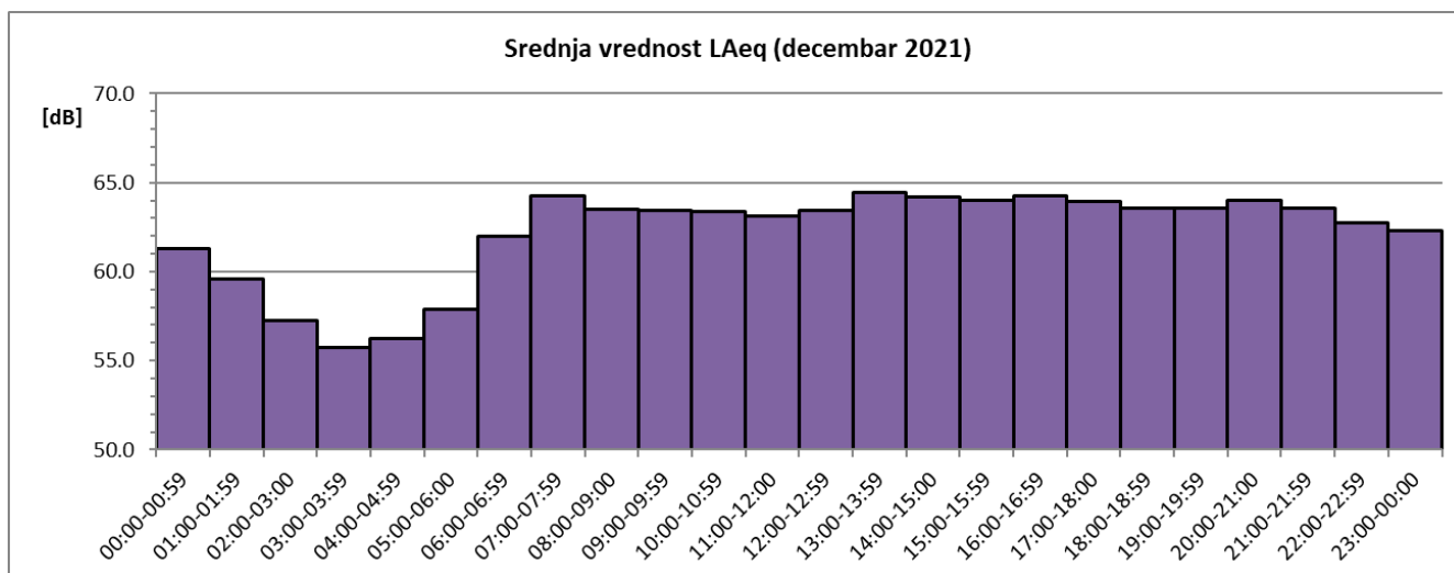
Sl. 3 Promene usrednjenih časovnih vrednosti ekvivalentnog nivoa buke u toku decembra 2021. za NMT-1
