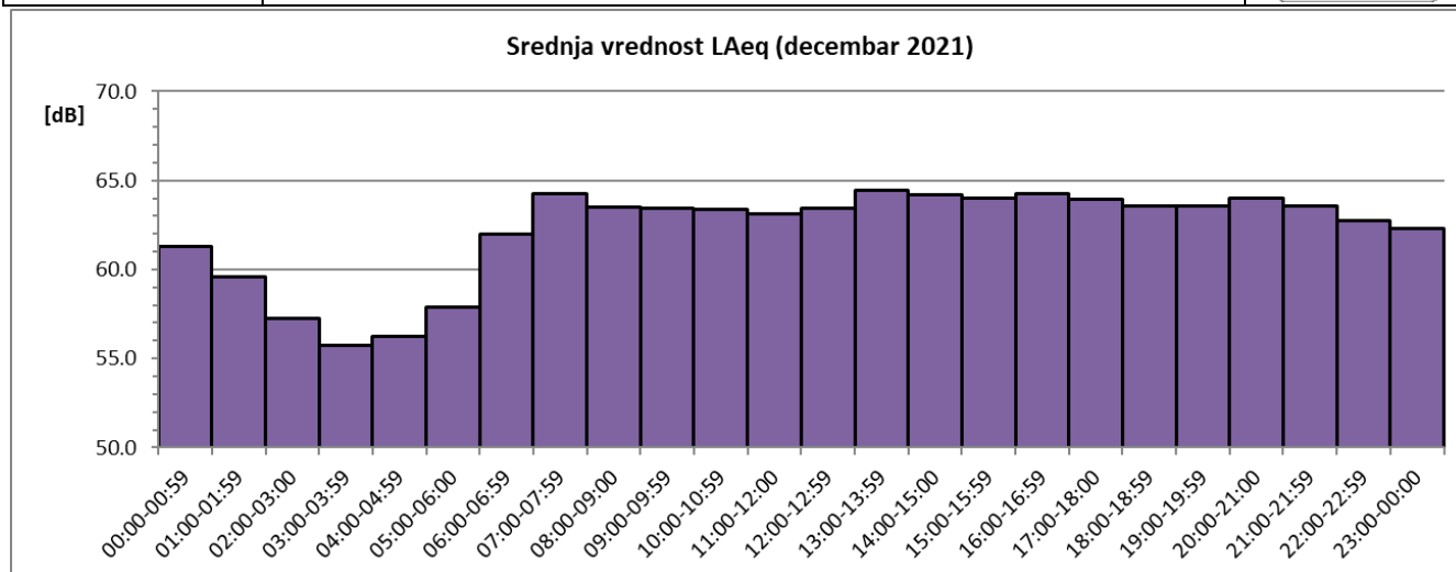
Sl. 5 Promene usrednjenih petnaestominutnih vrednosti ekvivalentnog nivoa buke u toku decembra 2021. za NMT-1
