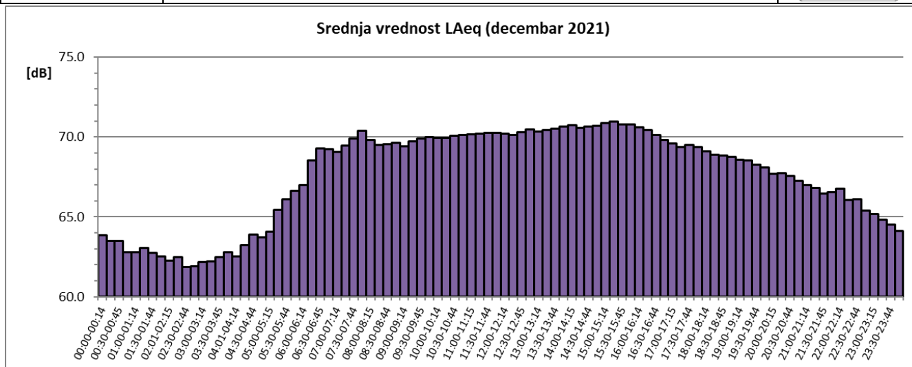
Sl. 6 Promene usrednjenih petnaestominutnih vrednosti ekvivalentnog nivoa buke u toku decembra 2021. za NMT-2
