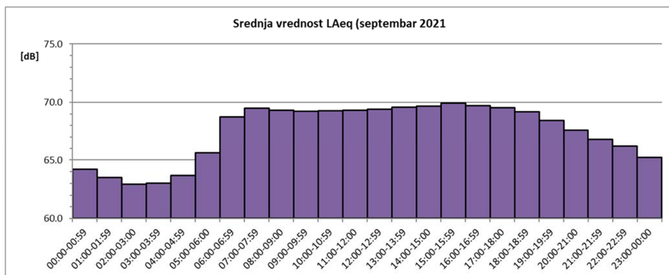
Sl. 4 Promene usrednjenih časovnih vrednosti ekvivalentnog nivoa buke u toku septembra 2021. za NMT-2
