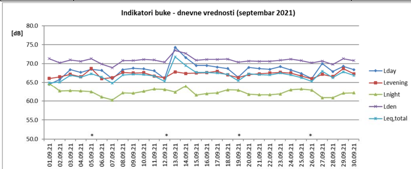
Sl. 1 Promene dnevnih vrednosti indikatora buke u toku septembra 2021. za NMT-1
