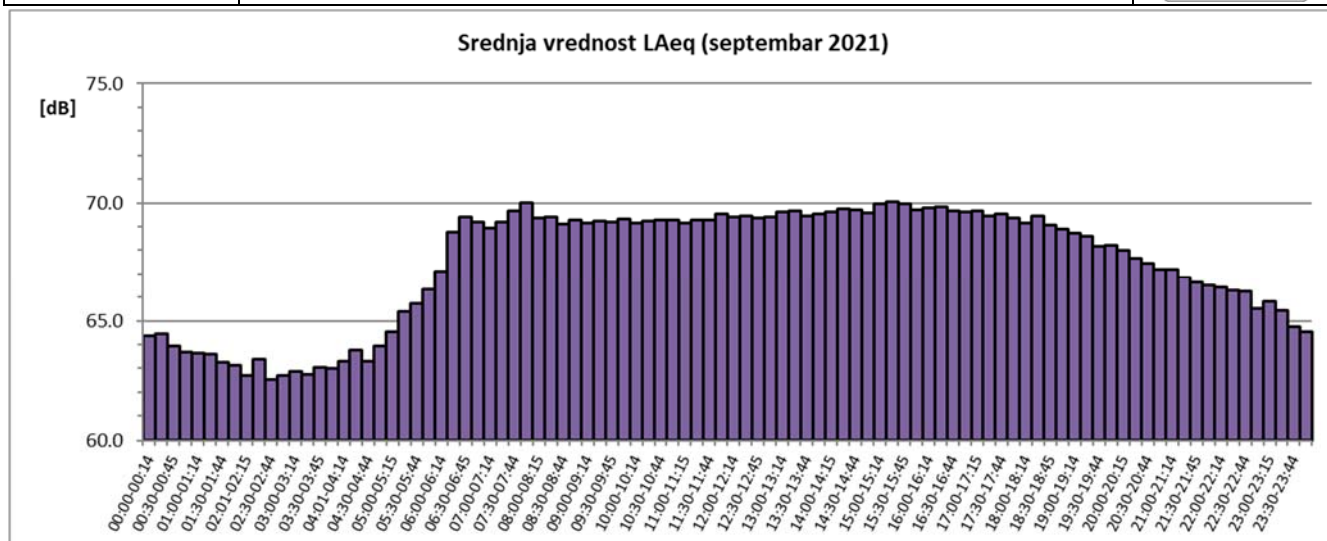
Sl. 6 Promene usrednjenih petnaestominutnih vrednosti ekvivalentnog nivoa buke u toku septembra 2021. za NMT-2
