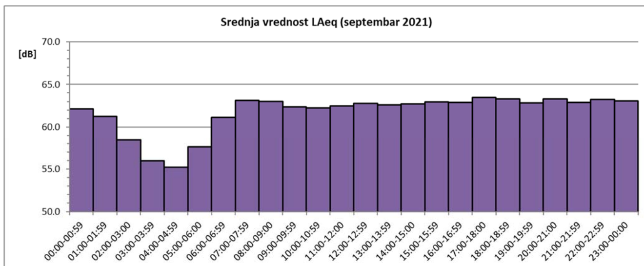
Sl. 3 Promene usrednjenih časovnih vrednosti ekvivalentnog nivoa buke u toku septembra 2021. za NMT-1
