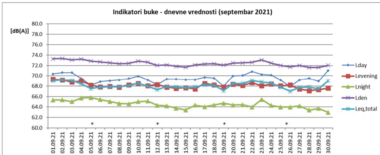
Sl. 2 Promene dnevnih vrednosti indikatora buke u toku septembra 2021. za NMT-2
