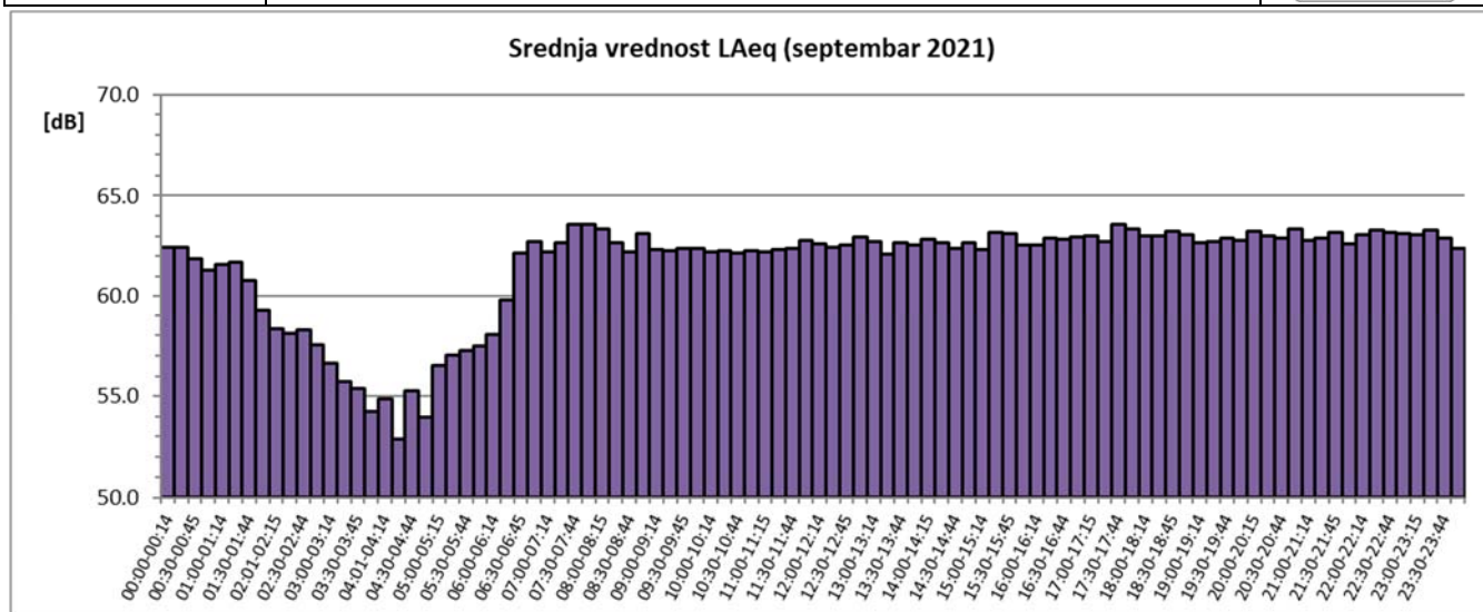
Sl. 5 Promene usrednjenih petnaestominutnih vrednosti ekvivalentnog nivoa buke u toku septembra 2021. za NMT-1
