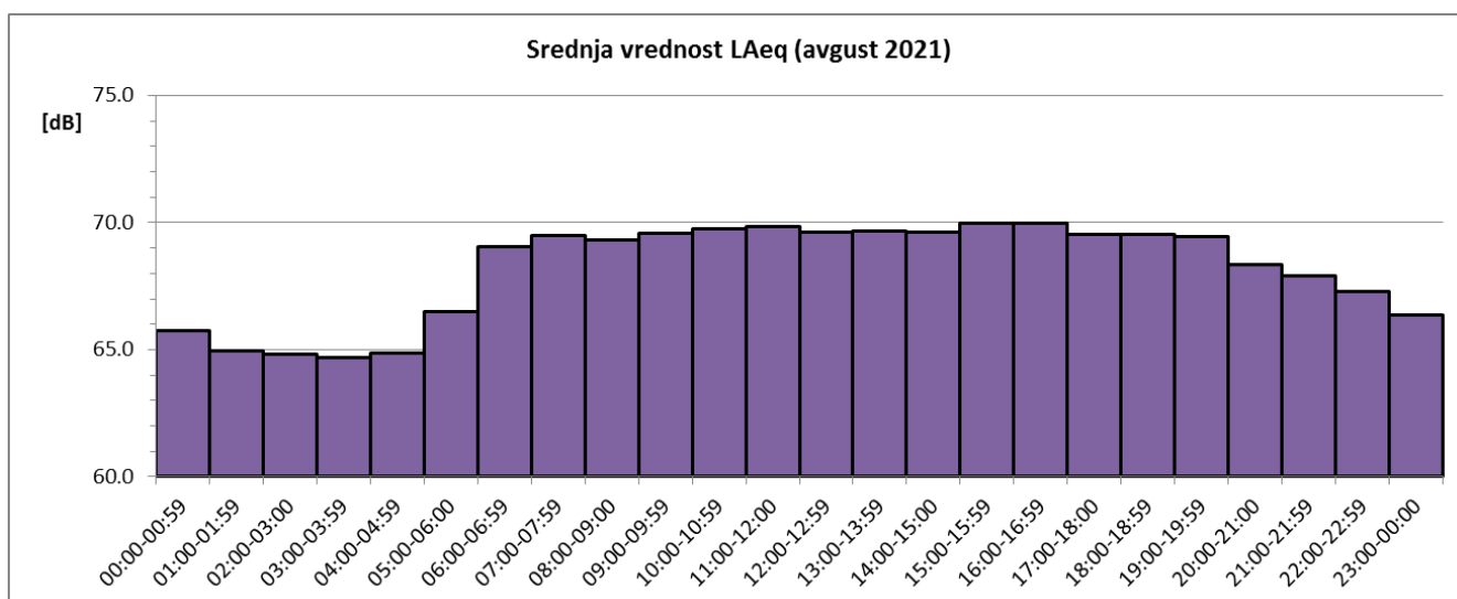
Sl. 4 Promene usrednjenih časovnih vrednosti ekvivalentnog nivoa buke u toku avgusta 2021. za NMT-2
