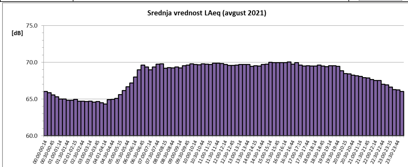
Sl. 6 Promene usrednjenih petnaestominutnih vrednosti ekvivalentnog nivoa buke u toku avgusta 2021. za NMT-2
