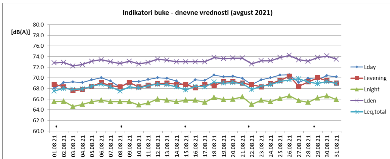
Sl. 2 Promene dnevnih vrednosti indikatora buke u toku avgusta 2021. za NMT-2
