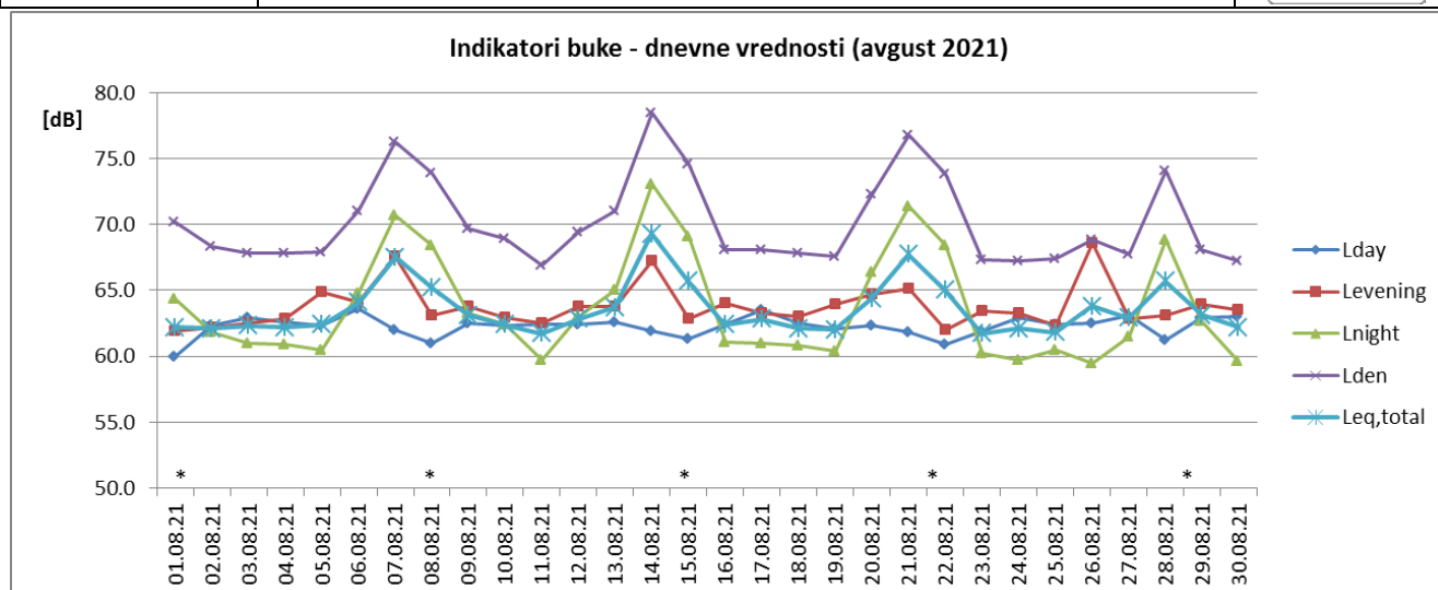
Sl. 1 Promene dnevnih vrednosti indikatora buke u toku avgusta 2021. za NMT-1
