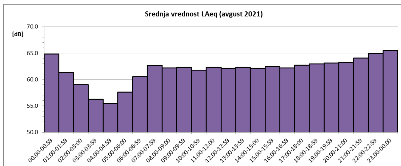
Sl. 3 Promene usrednjenih časovnih vrednosti ekvivalentnog nivoa buke u toku avgusta 2021. za NMT-1
