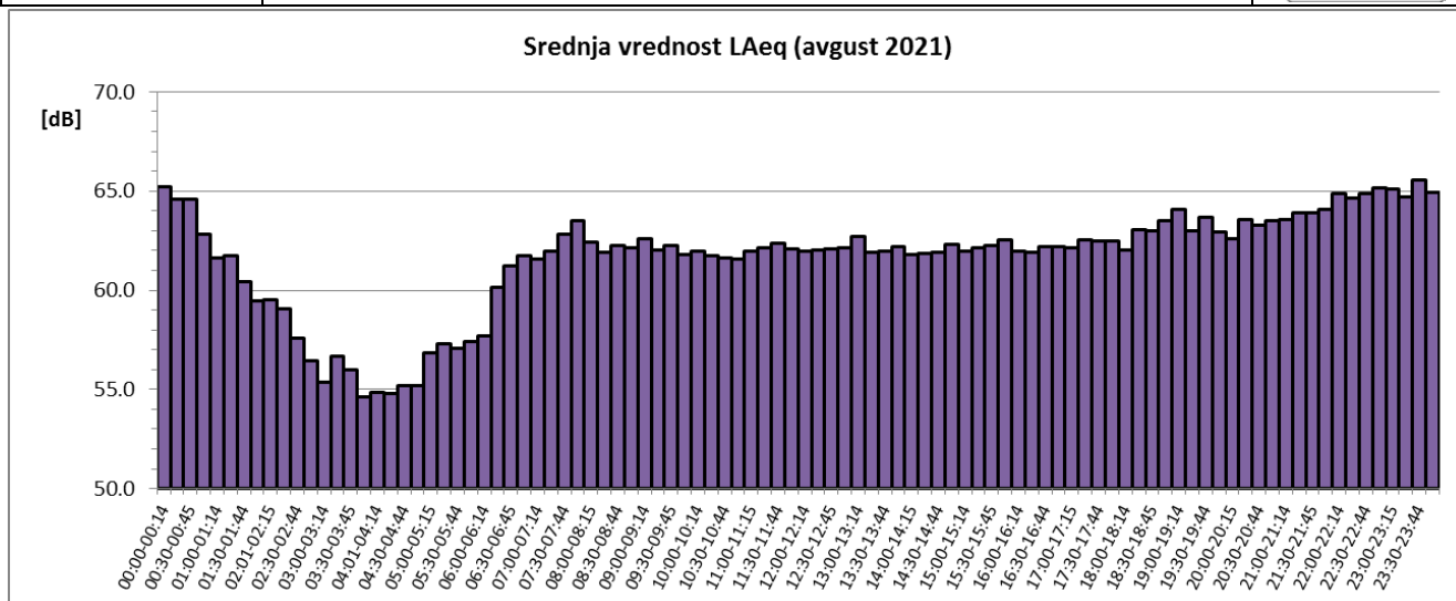
Sl. 5 Promene usrednjenih petnaestominutnih vrednosti ekvivalentnog nivoa buke u toku avgusta 2021. za NMT-1
