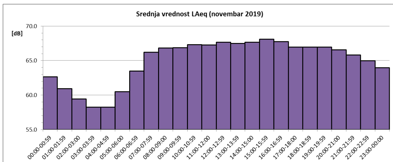
Sl. 3 Promene usrednjenih časovnih vrednosti ekvivalentnog nivoa buke u toku nobembra 2019 za NMT-1
