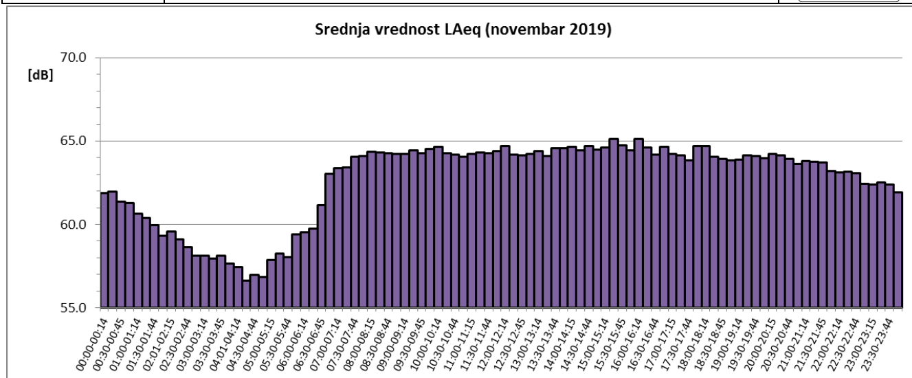
Sl. 6 Promene usrednjenih petnaestominutnih vrednosti ekvivalentnog nivoa buke u toku novembra 2019 za NMT-2
