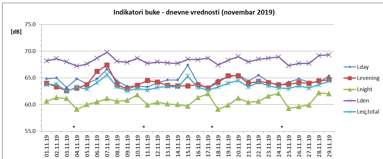
Sl. 2 Promene dnevnih vrednosti indikatora buke u toku novembra 2019 za NMT-2
