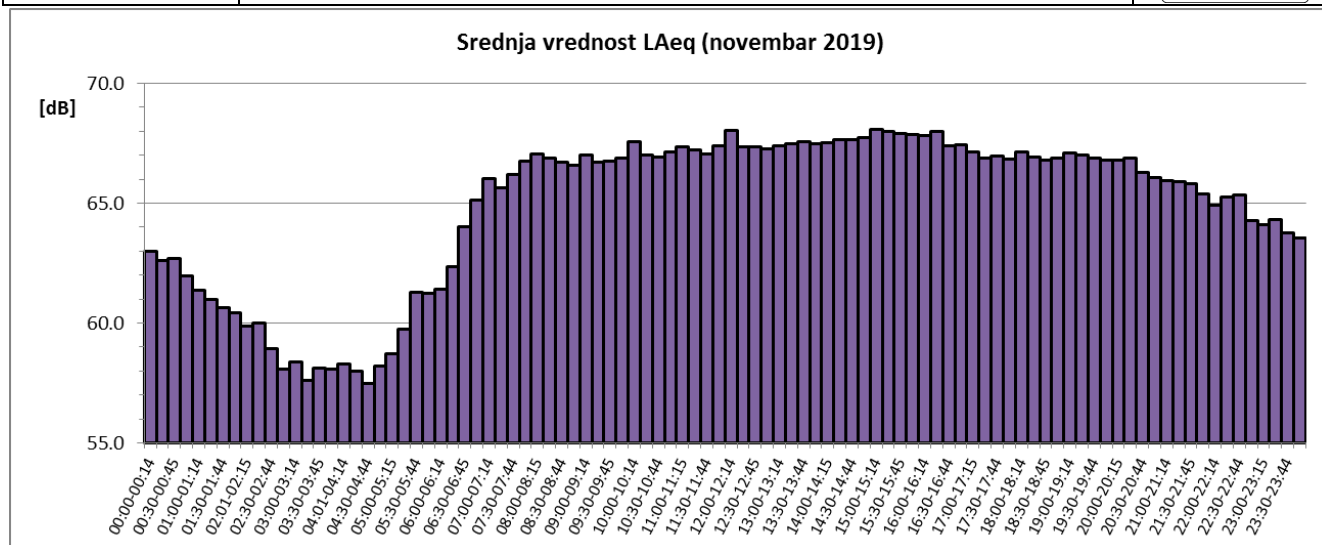
Sl. 5 Promene usrednjenih petnaestominutnih vrednosti ekvivalentnog nivoa buke u toku novembra 2019 za NMT-1
