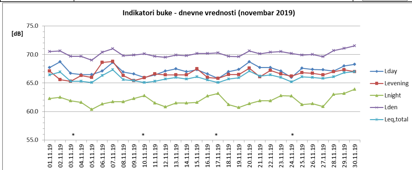
Sl. 1 Promene dnevnih vrednosti indikatora buke u toku novembra 2019 za NMT-1
