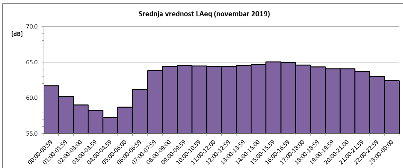
Sl. 4 Promene usrednjenih časovnih vrednosti ekvivalentnog nivoa buke u toku novembra 2019 za NMT-2
