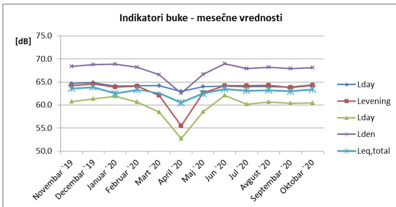
Sl. 2 Promene mesečnih vrednosti indikatora buke u toku 2019/2020 za NMT-2
