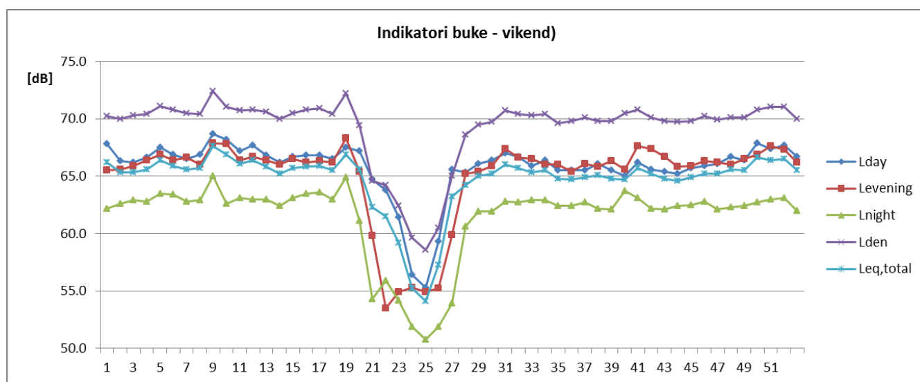
Sl. 7 Promene vikend vrednosti indikatora buke u toku 2019/2020 za NMT-1
