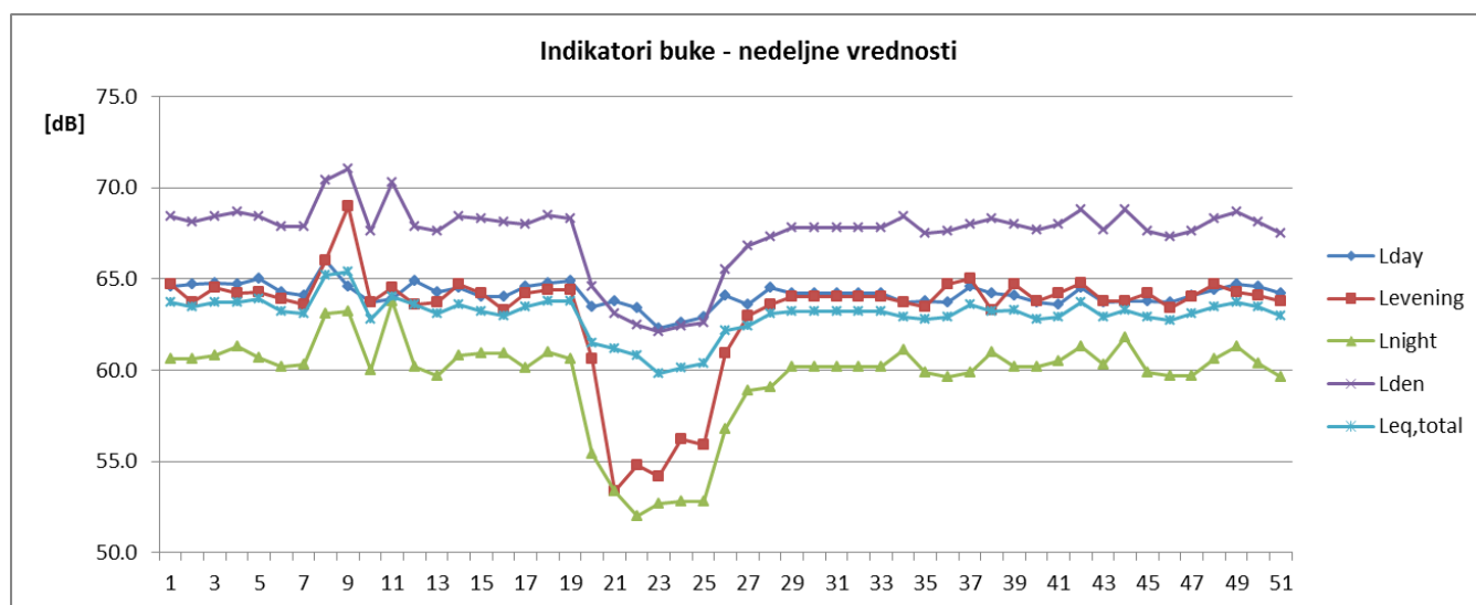
Sl. 4 Promene nedeljnih vrednosti indikatora buke u toku 2019/2020 za NMT-2
