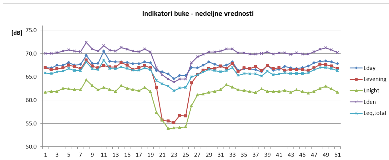
Sl. 3 Promene nedeljnih vrednosti indikatora buke u toku 2019-2020 za NMT-1
