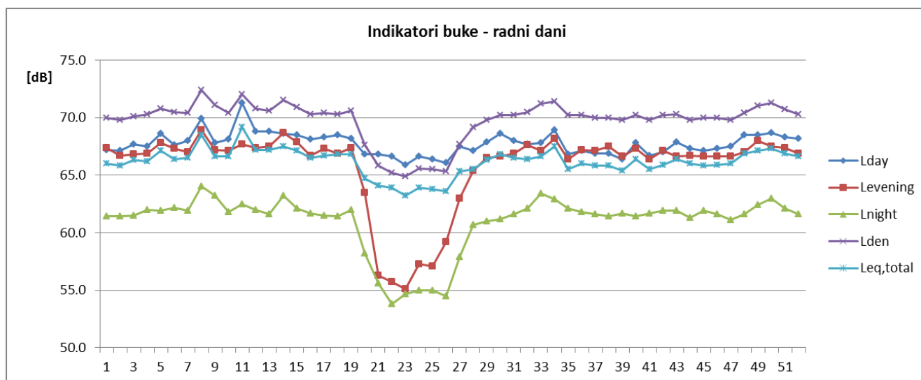
Sl. 5 Promene petodnevних (radni dani) vrednosti indikatora buke u toku 2019/2020 za NMT-1
