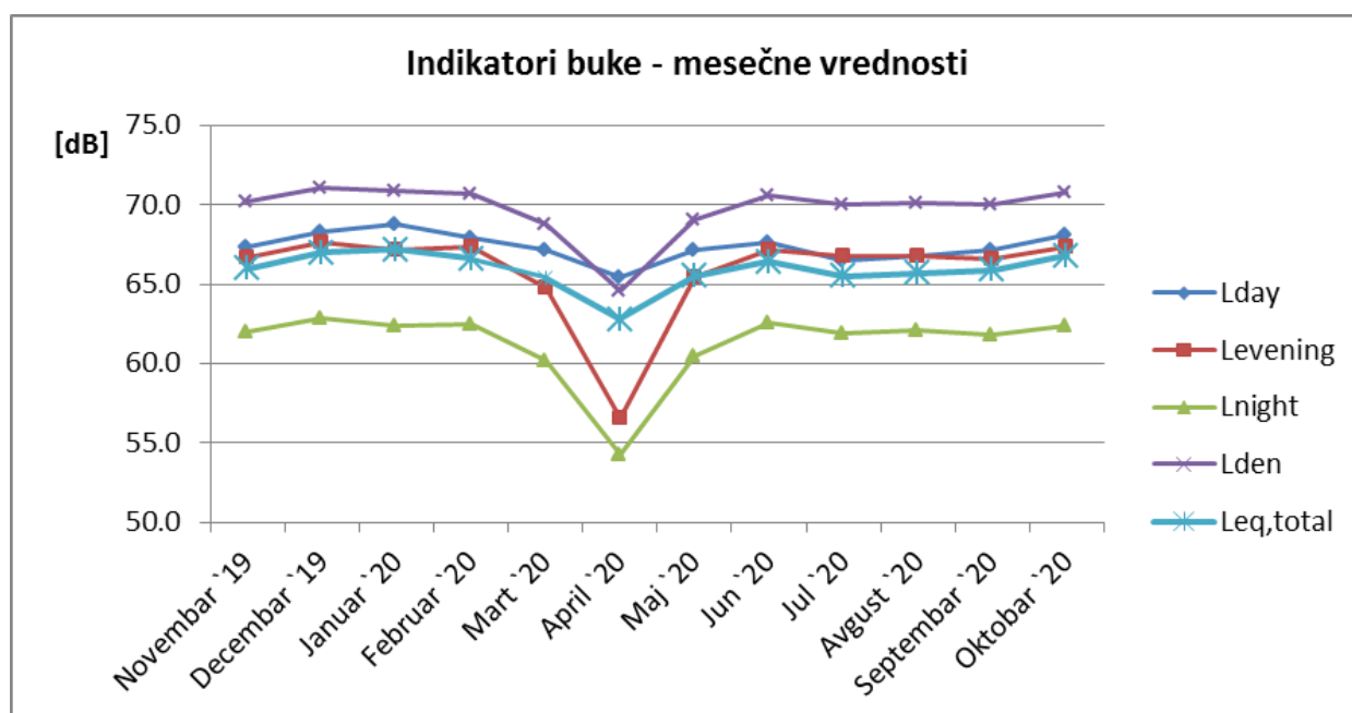
Sl. 1 Promene mesečnih vrednosti indikatora buke u toku 2019/2020 za NMT-1
