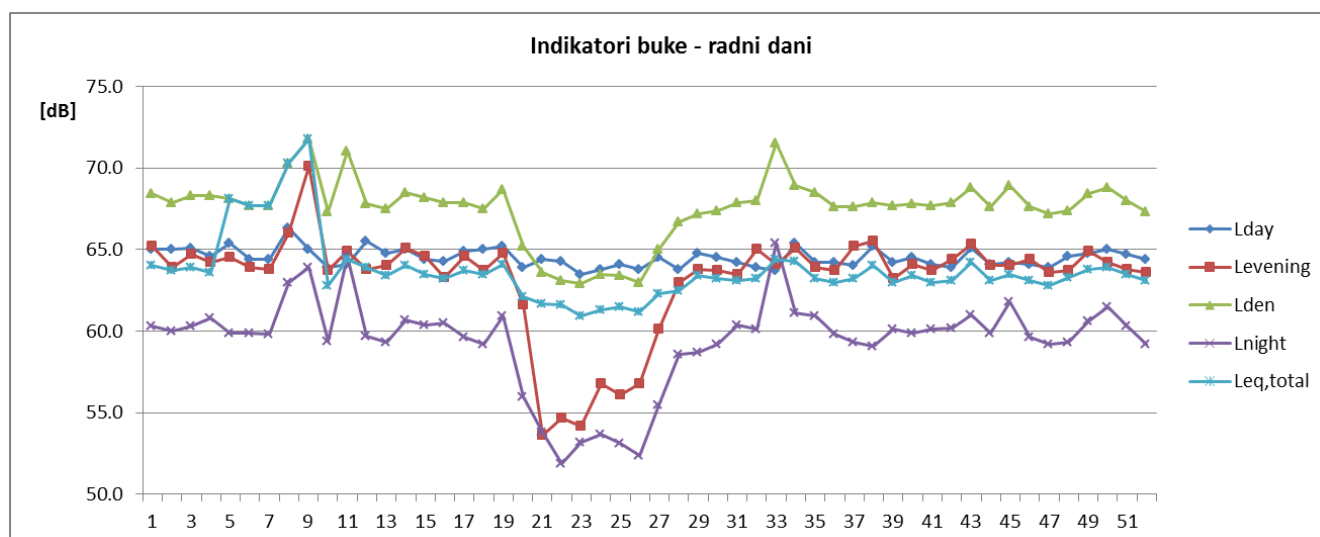
Sl. 6 Promene petodnevni (radni dani) vrednosti indikatora buke u toku 2019/2020 za NMT-2
