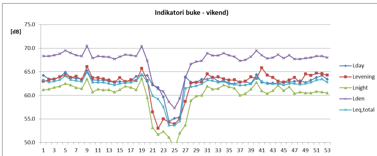
Sl. 8 Promene vikend vrednosti indikatora buke u toku 2019/2020 za NMT-2
