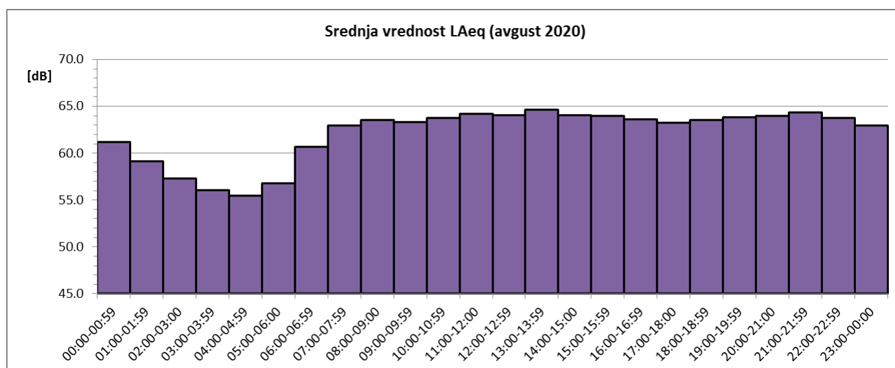
Sl. 4 Promene usrednjenih časovnih vrednosti ekvivalentnog nivoa buke u toku avgusta 2020. za NMT-2
