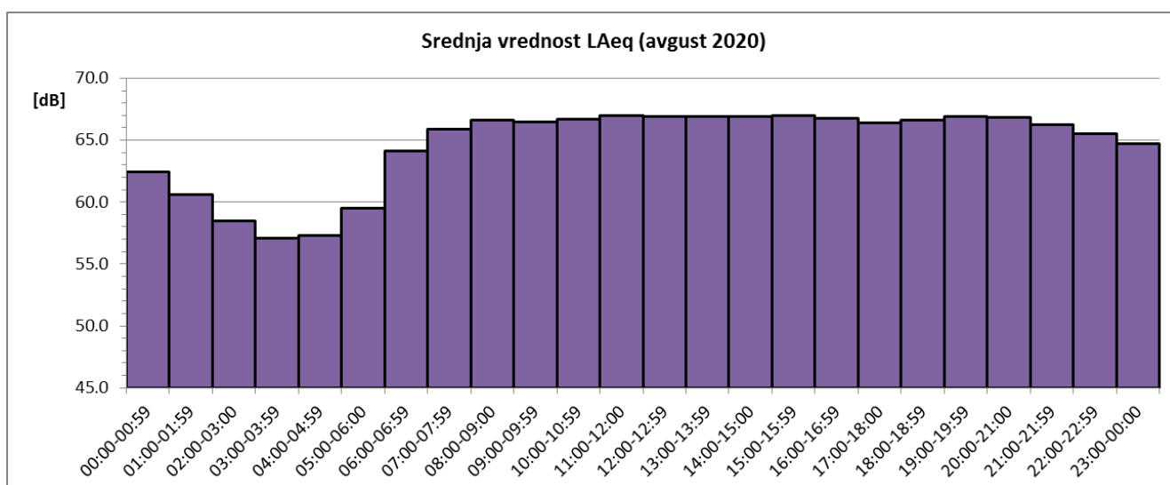
Sl. 3 Promene usrednjenih časovnih vrednosti ekvivalentnog nivoa buke u toku avgusta 2020. za NMT-1
