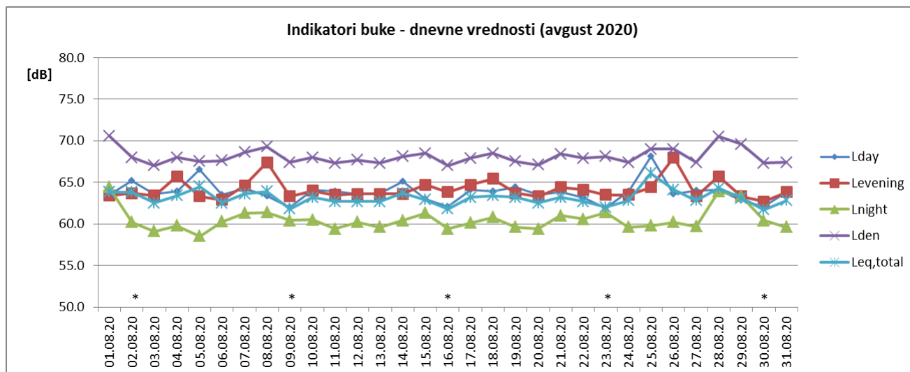
Sl. 2 Promene dnevnih vrednosti indikatora buke u toku avgusta 2020. za NMT-2
