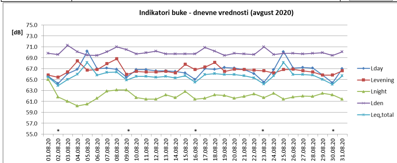
Sl. 1 Promene dnevnih vrednosti indikatora buke u toku avgusta 2020. za NMT-1
