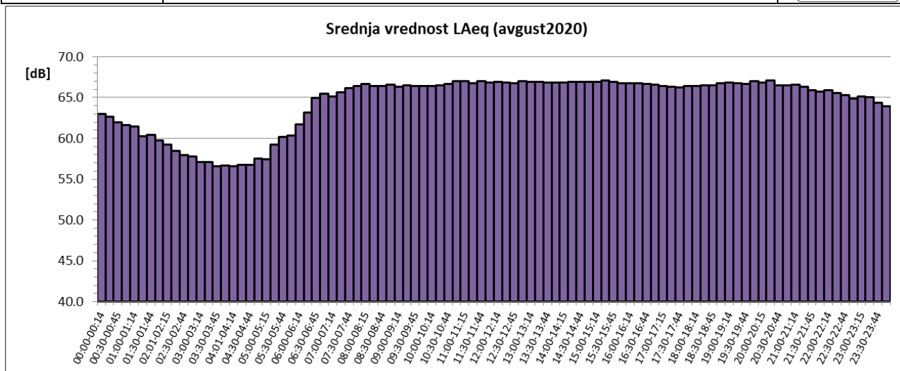
Sl. 5 Promene usrednjenih petnaestominutnih vrednosti ekvivalentnog nivoa buke u toku avgusta 2020. za NMT-1
