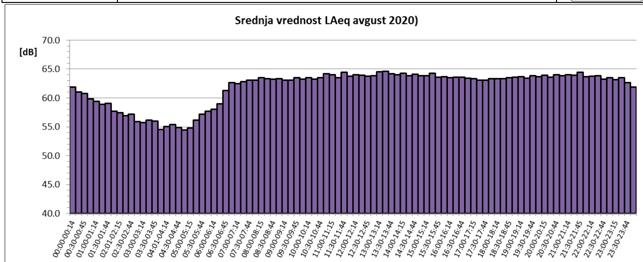
Sl. 6 Promene usrednjenih petnaestominutnih vrednosti ekvivalentnog nivoa buke u toku avgusta 2020. za NMT-2
