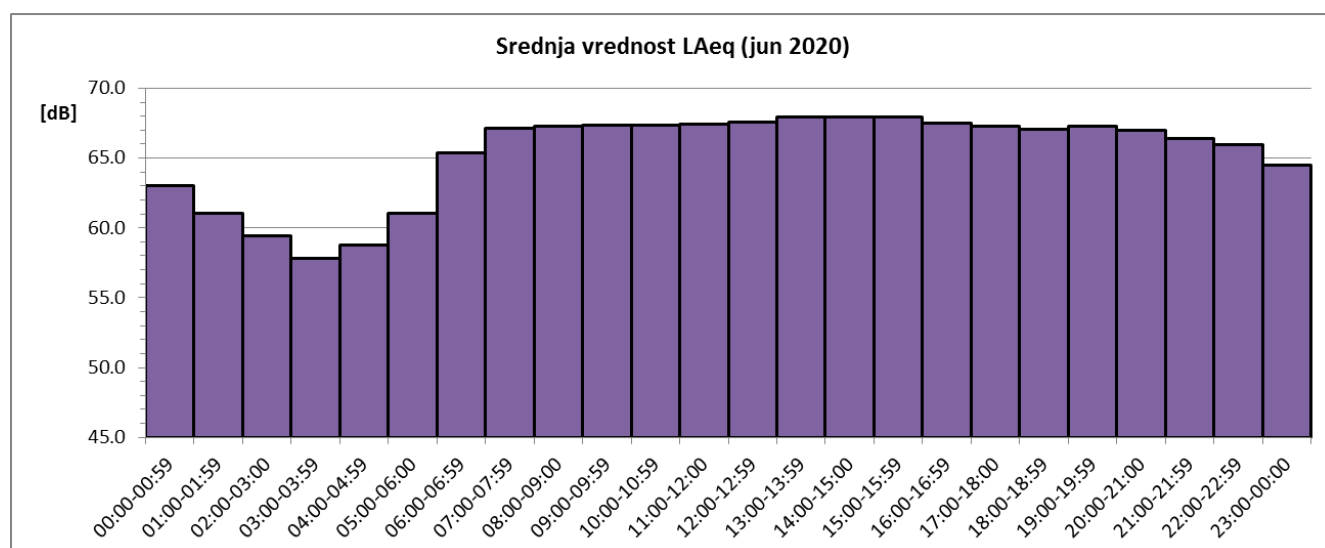
Sl. 3 Promene usrednjenih časovnih vrednosti ekvivalentnog nivoa buke u toku juna 2020. za NMT-1
