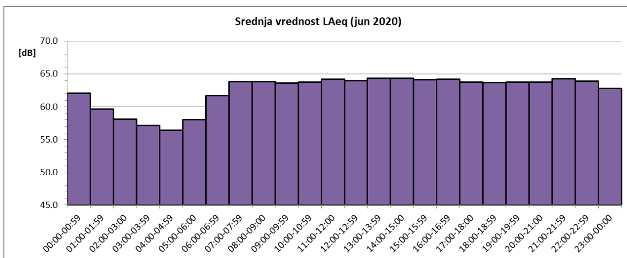
Sl. 4 Promene usrednjenih časovnih vrednosti ekvivalentnog nivoa buke u toku juna 2020. za NMT-2
