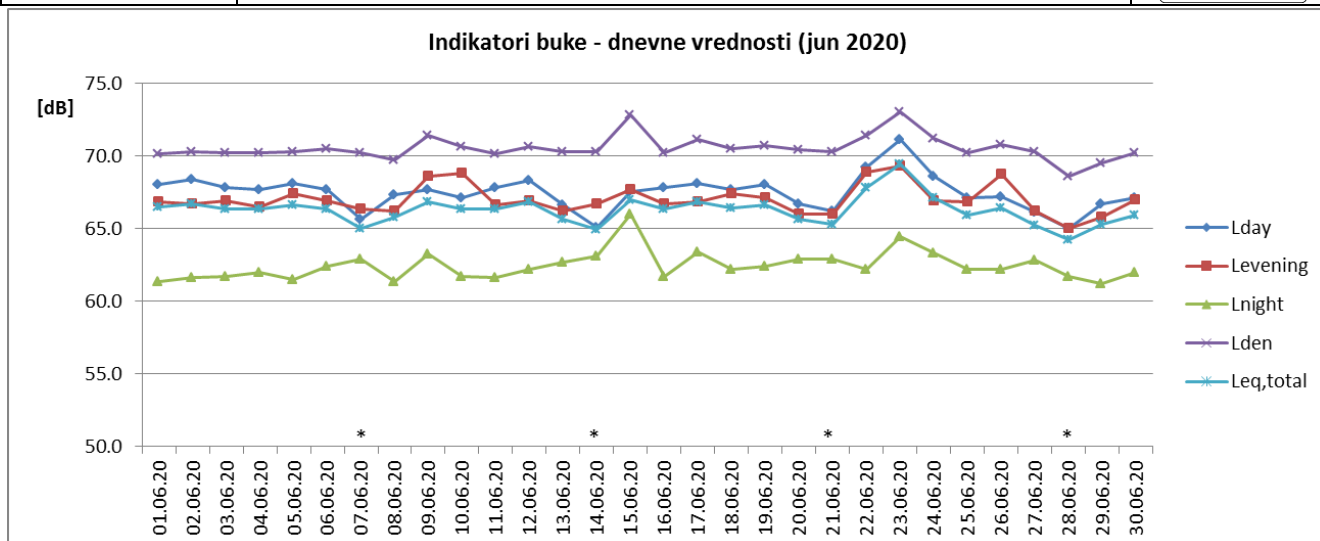
Sl. 1 Promene dnevnih vrednosti indikatora buke u toku juna 2020. za NMT-1
