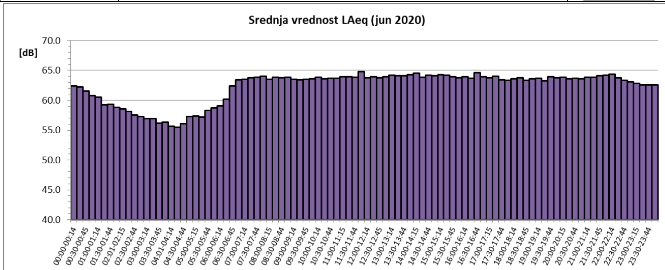
Sl. 6 Promene usrednjenih petnaestominutnih vrednosti ekvivalentnog nivoa buke u toku juna 2020. za NMT-2
