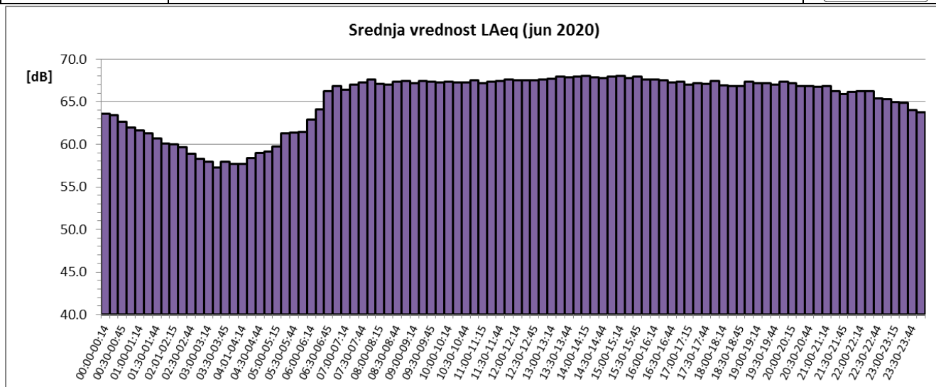
Sl. 5 Promene usrednjenih petnaestominutnih vrednosti ekvivalentnog nivoa buke u toku juna 2020. za NMT-1
