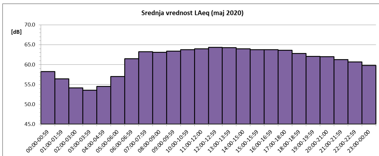
Sl. 4 Promene usrednjenih časovnih vrednosti ekvivalentnog nivoa buke u toku maja 2020. za NMT-2
