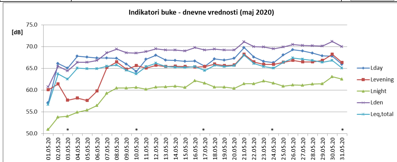
Sl. 1 Promene dnevnih vrednosti indikatora buke u toku maja 2020. za NMT-1
