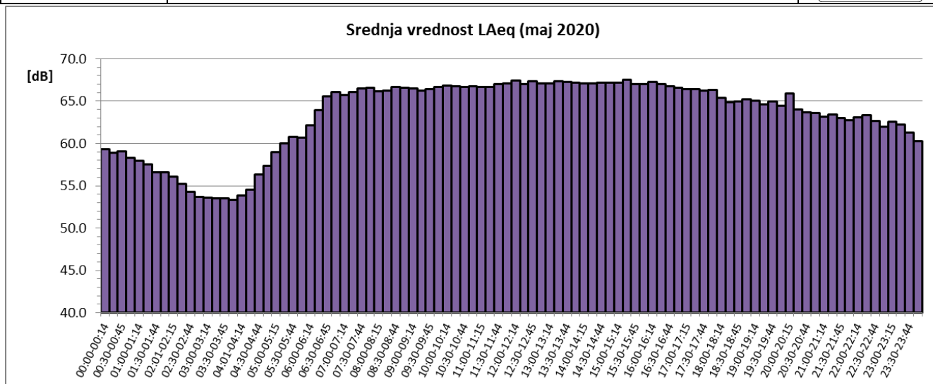
Sl. 5 Promene usrednjenih petnaestominutnih vrednosti ekvivalentnog nivoa buke u toku maja 2020. za NMT-1
