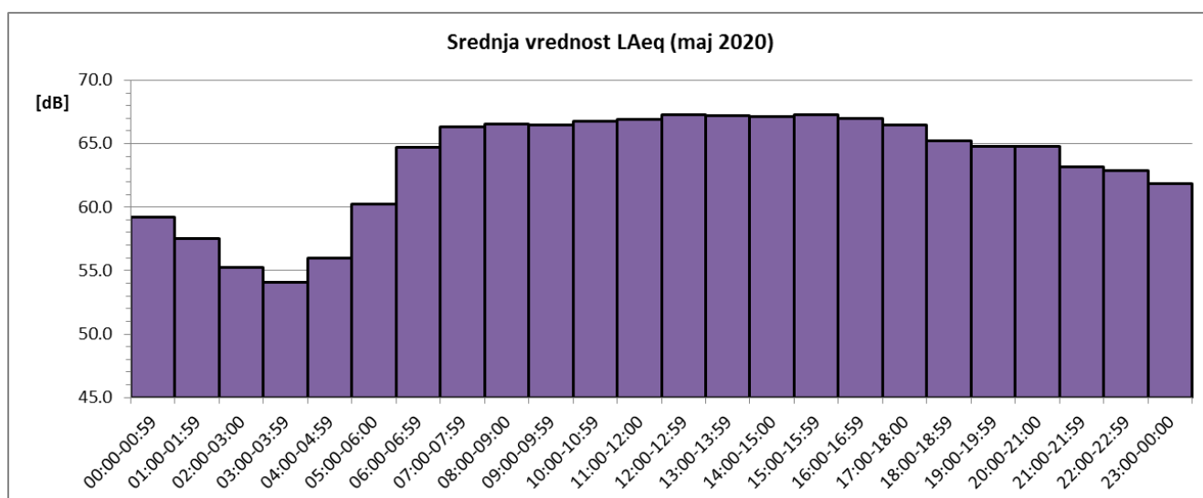
Sl. 3 Promene usrednjenih časovnih vrednosti ekvivalentnog nivoa buke u toku maja 2020. za NMT-1
