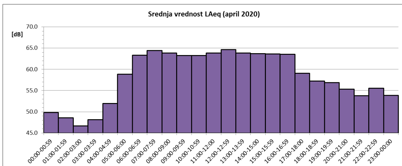
Sl. 3 Promene usrednjenih časovnih vrednosti ekvivalentnog nivoa buke u toku aprila 2020. za NMT-1
