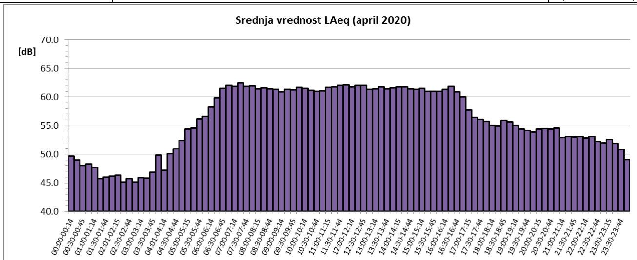
Sl. 6 Promene usrednjenih petnaestominutnih vrednosti ekvivalentnog nivoa buke u toku aprila 2020. za NMT-2
