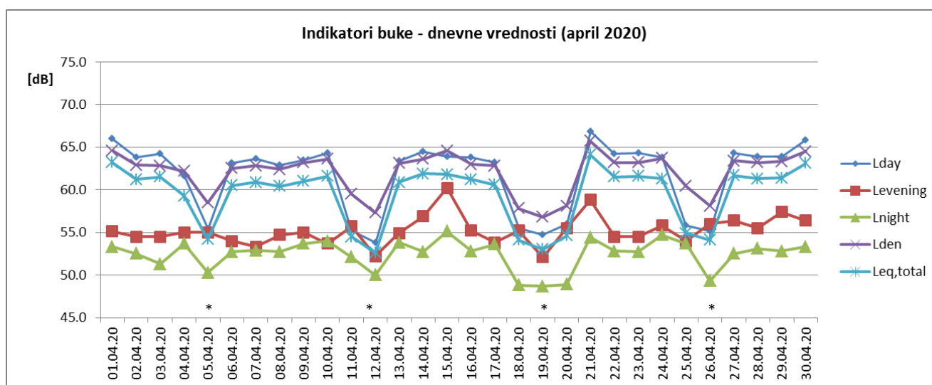
Sl. 4 Promene usrednjenih časovnih vrednosti ekvivalentnog nivoa buke u toku aprila 2020. za NMT-2
