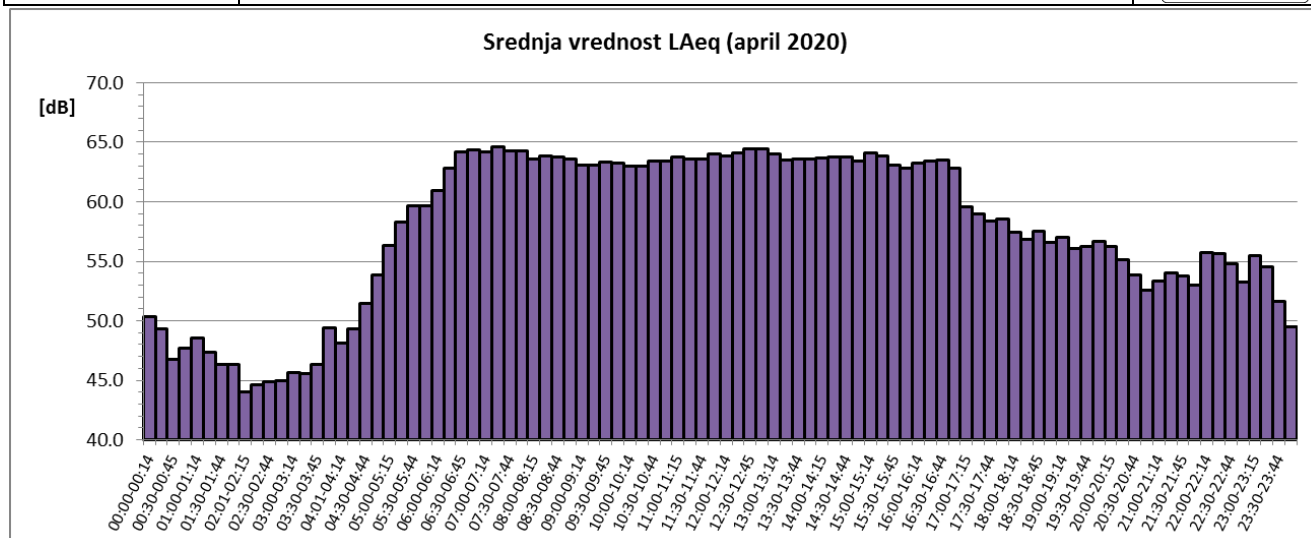
Sl. 5 Promene usrednjenih petnaestominutnih vrednosti ekvivalentnog nivoa buke u toku aprila 2020. za NMT-1
