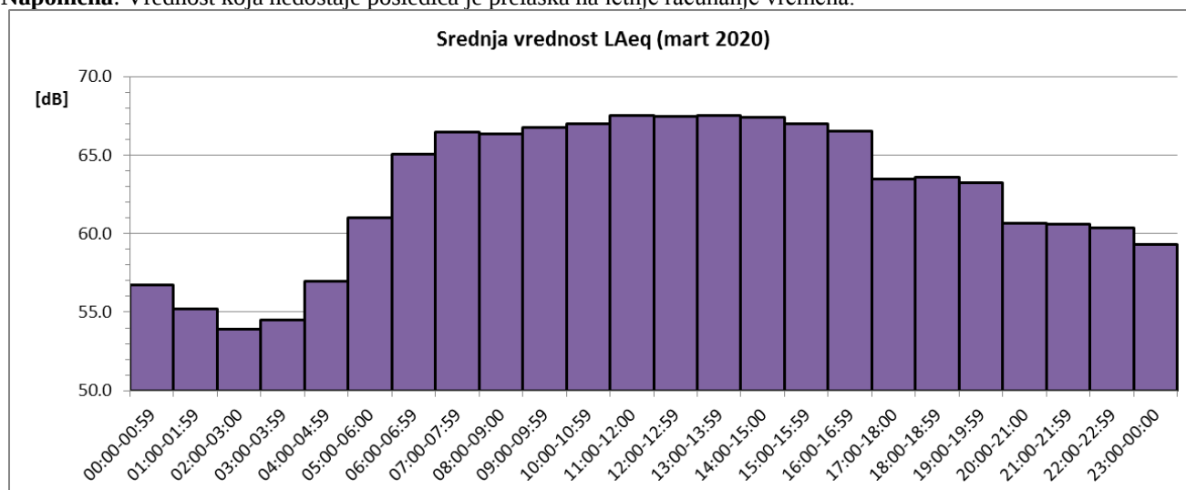
Sl. 3 Promene usrednjenih časovnih vrednosti ekvivalentnog nivoa buke u toku marta 2020. za NMT-1
