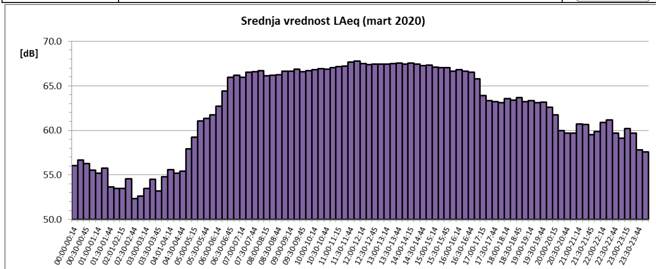
Sl. 5 Promene usrednjenih petnaestominutnih vrednosti ekvivalentnog nivoa buke u toku marta 2020. za NMT-1
