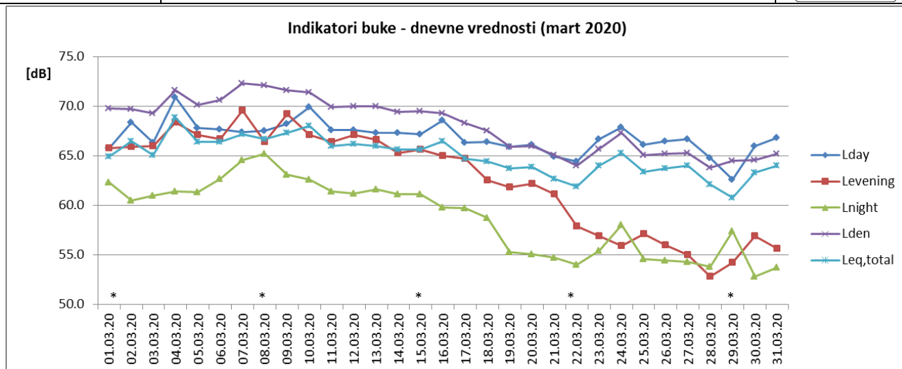
SI. 1 Promene dnevnih vrednosti indikatora buke u toku marta 2020. za NMT-1
