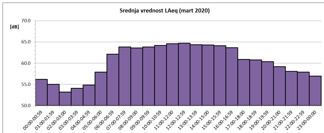
Sl. 4 Promene usrednjenih časovnih vrednosti ekvivalentnog nivoa buke u toku marta 2020. za NMT-2
