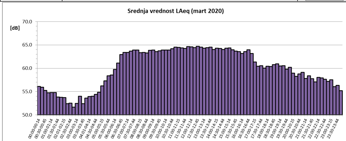
Sl. 6 Promene usrednjenih petnaestominutnih vrednosti ekvivalentnog nivoa buke u toku marta 2020. za NMT-2
