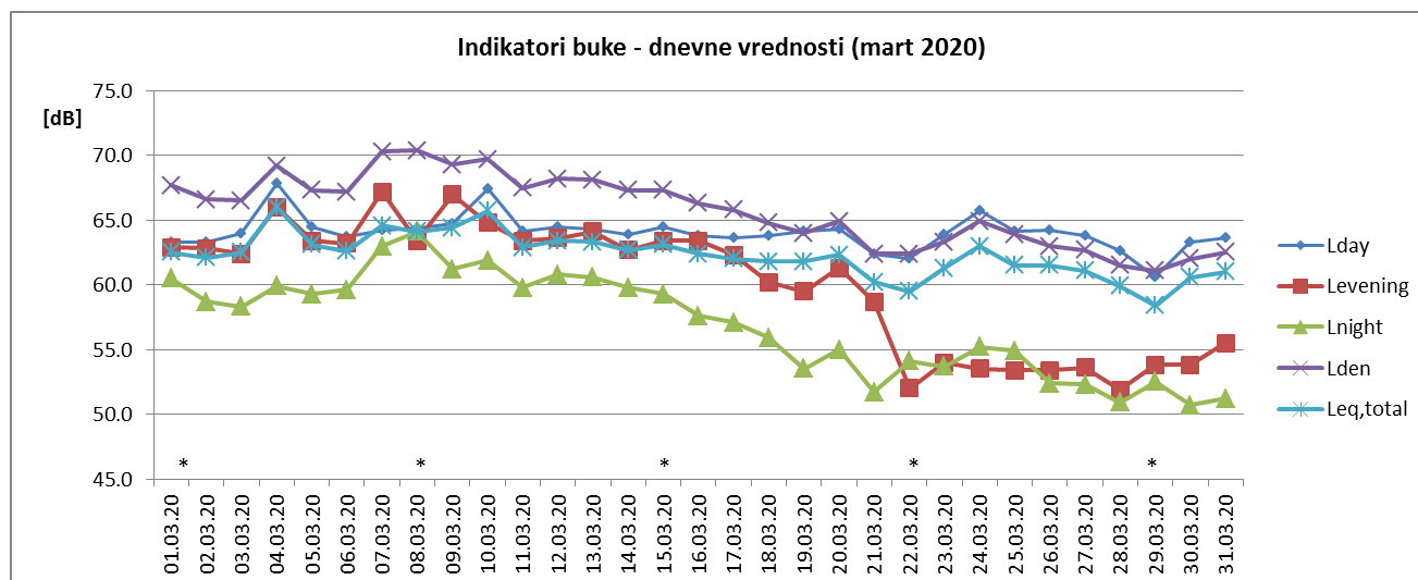
SI. 2 Promene dnevnih vrednosti indikatora buke u toku marta 2020. za NMT-2
