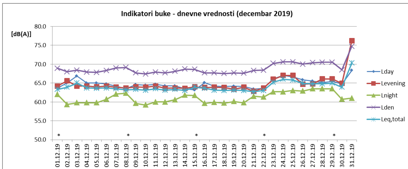
Sl. 2 Promene dnevnih vrednosti indikatora buke u toku decembra 2019 za NMT-2
