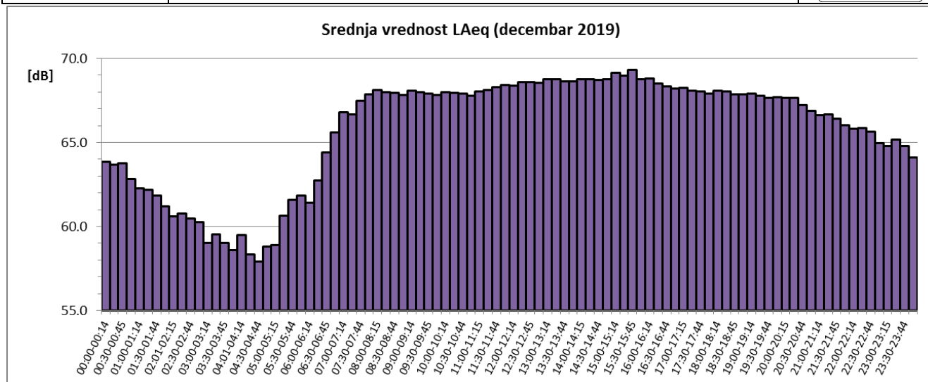
Sl. 5 Promene usrednjenih petnaestominutnih vrednosti ekvivalentnog nivoa buke u toku decembra 2019 za NMT-1
