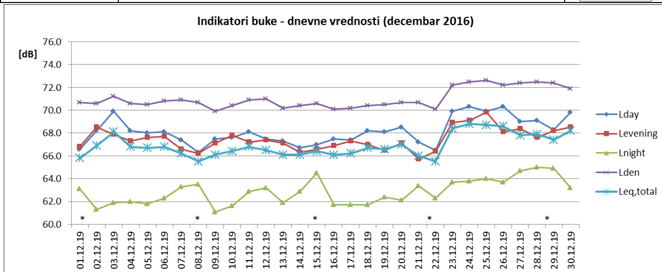
Sl. 1 Promene dnevnih vrednosti indikatora buke u toku decembra 2019 za NMT-1
