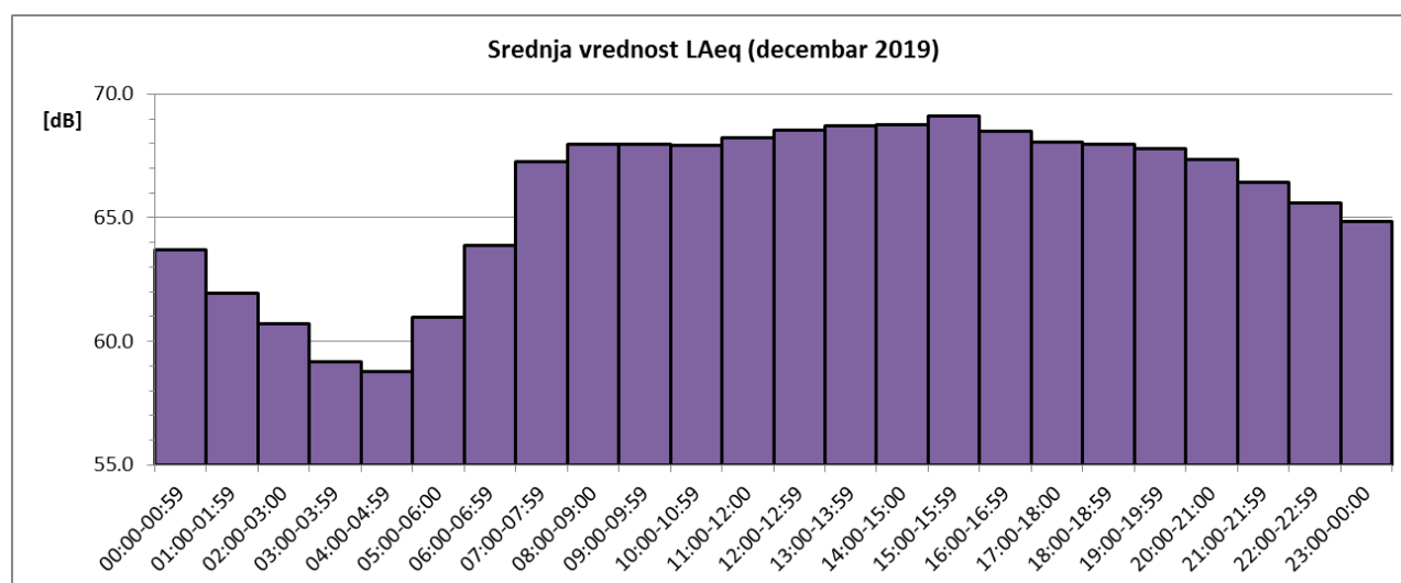
Sl. 3 Promene usrednjenih časovnih vrednosti ekvivalentnog nivoa buke u toku decembra 2019 za NMT-1
