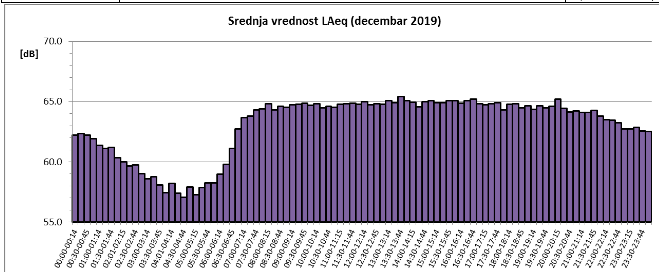
Sl. 6 Promene usrednjenih petnaestominutnih vrednosti ekvivalentnog nivoa buke u toku decembra 2019 za NMT-2
