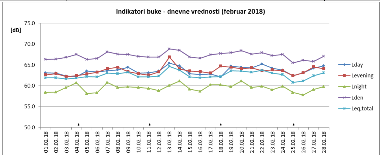
Sl. 1 Promene dnevnih vrednosti indikatora buke u toku februara 2018 za NMT-1
