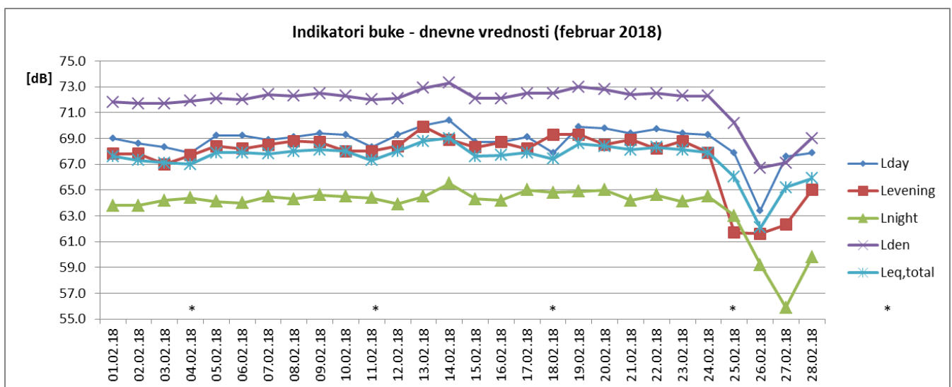
Sl. 2 Promene dnevnih vrednosti indikatora buke u toku februara 2018 za NMT-2
