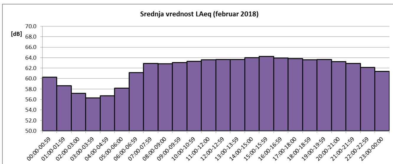
Sl. 3 Promene usrednjenih časovnih vrednosti ekvivalentnog nivoa buke u toku februara 2018 za NMT-1
