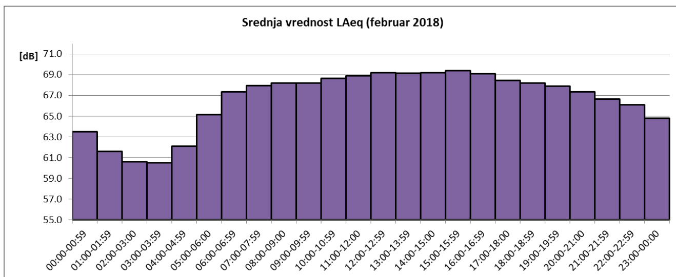
Sl. 4 Promene usrednjenih časovnih vrednosti ekvivalentnog nivoa buke u toku februara 2018 za NMT-2
