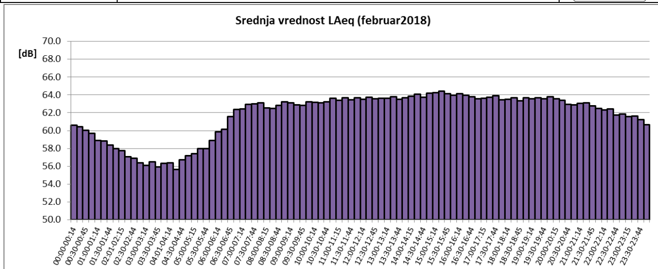
Sl. 5 Promene usrednjenih petnaestominutnih vrednosti ekvivalentnog nivoa buke u toku februara 2018 za NMT-1
