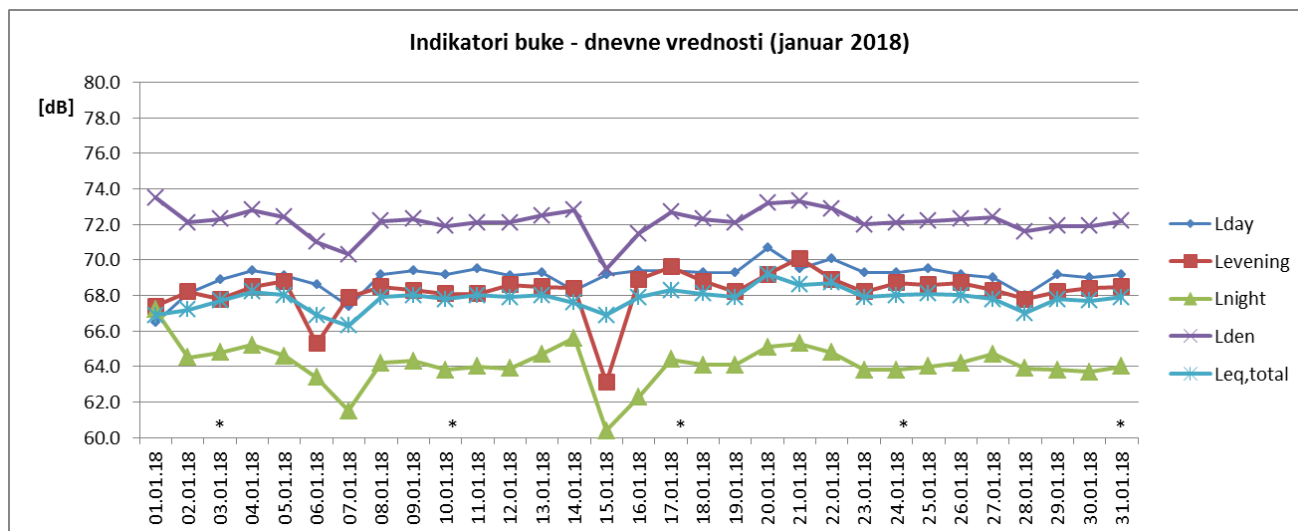
Sl. 1 Promene dnevnih vrednosti indikatora buke u toku januara 2018 za NMT-1
