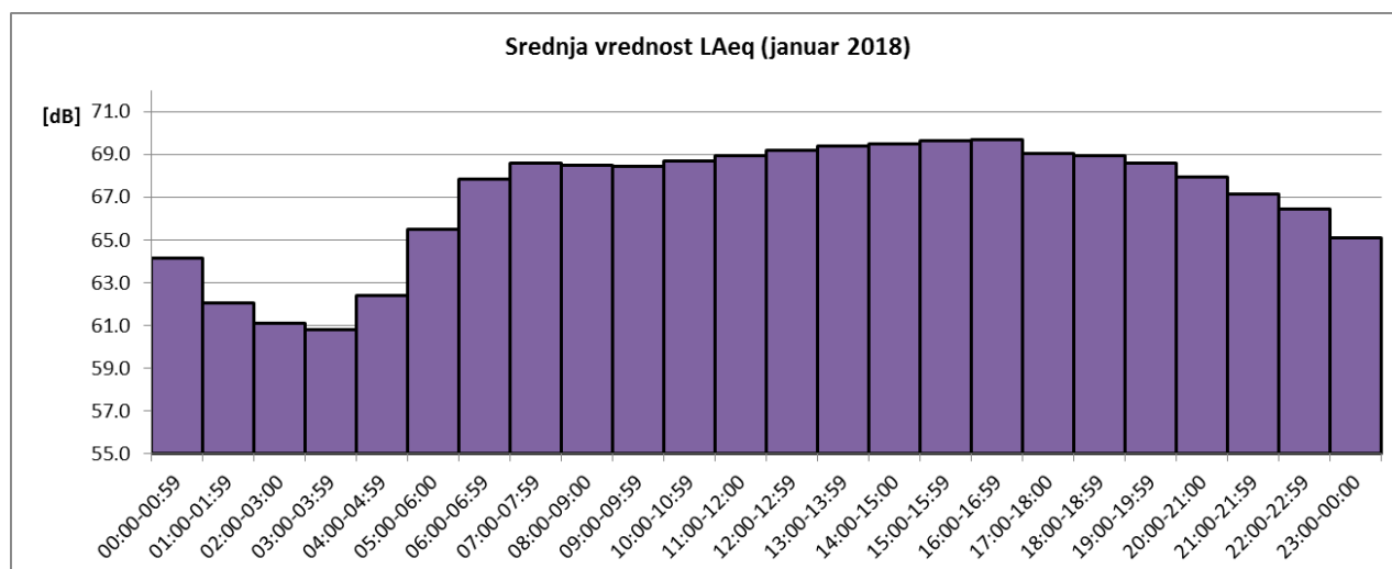
Sl. 4 Promene usrednjenih časovnih vrednosti ekvivalentnog nivoa buke u toku januara 2018 za NMT-2
