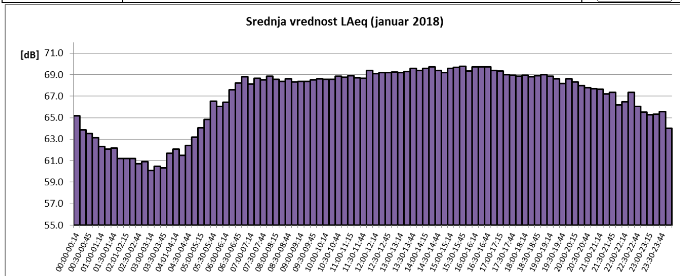
Sl. 5 Promene usrednjenih petnaestominutnih vrednosti ekvivalentnog nivoa buke u toku januara 2018 za NMT-1
