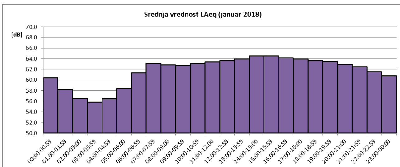
Sl. 3 Promene usrednjenih časovnih vrednosti ekvivalentnog nivoa buke u toku januara 2018 za NMT-1
