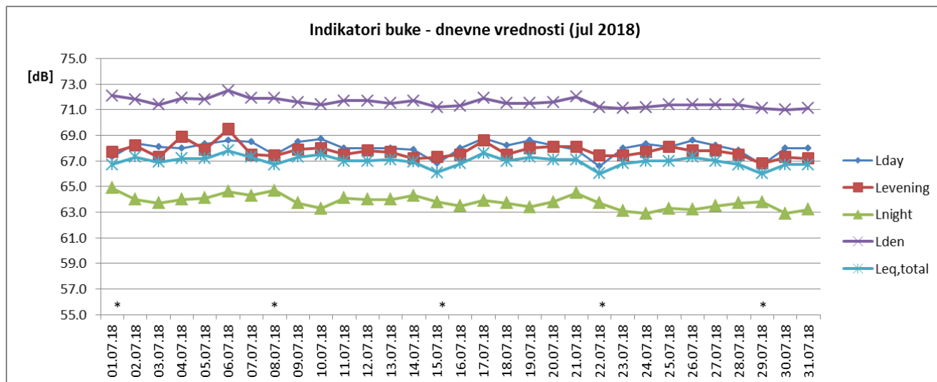
Sl. 2 Promene dnevnih vrednosti indikatora buke u toku jula 2018 za NMT-2
