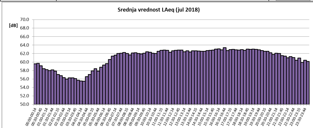
Sl. 5 Promene usrednjenih petnaestominutnih vrednosti ekvivalentnog nivoa buke u toku jula 2018 za NMT-1
