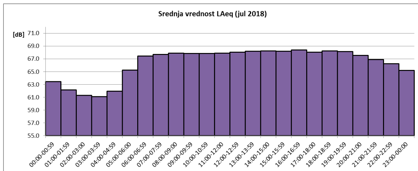
Sl. 4 Promene usrednjenih časovnih vrednosti ekvivalentnog nivoa buke u toku jula 2018 za NMT-2
