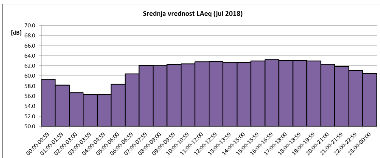
Sl. 3 Promene usrednjenih časovnih vrednosti ekvivalentnog nivoa buke u toku jula 2018 za NMT-1
