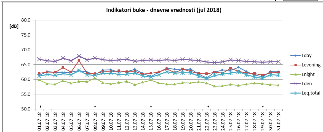
Sl. 1 Promene dnevnih vrednosti indikatora buke u toku jula 2018 za NMT-1
