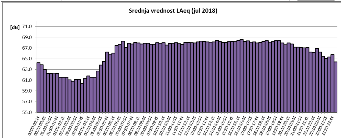
Sl. 6 Promene usrednjenih petnaestominutnih vrednosti ekvivalentnog nivoa buke u toku jula 2018 za NMT-2
