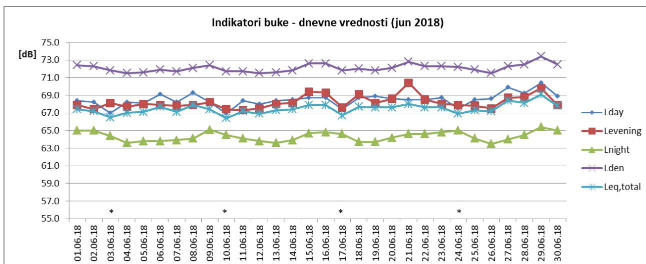
Sl. 2 Promene dnevnih vrednosti indikatora buke u toku juna 2018 za NMT-2
