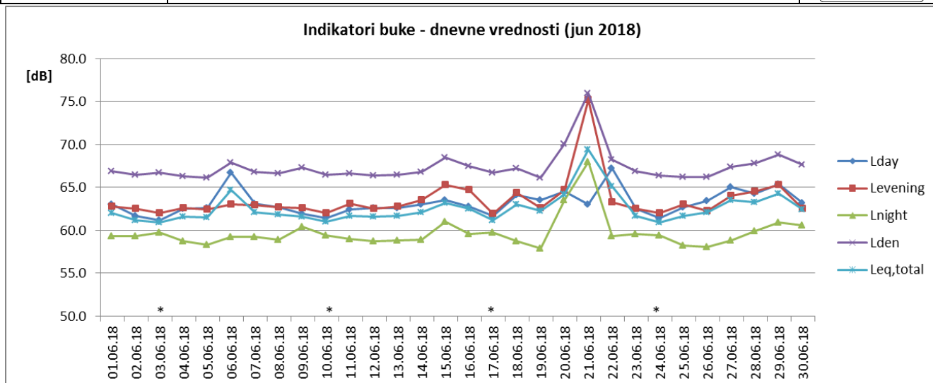
Sl. 1 Promene dnevnih vrednosti indikatora buke u toku juna 2018 za NMT-1
