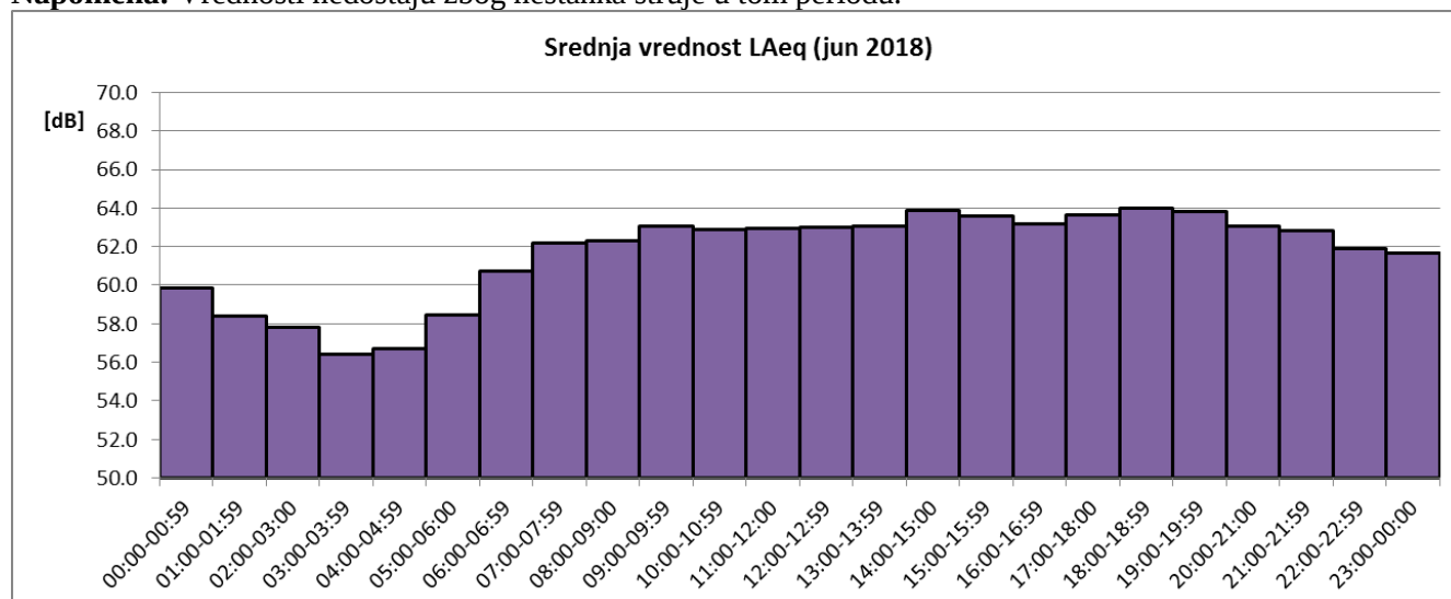
Sl. 3 Promene usrednjenih časovnih vrednosti ekvivalentnog nivoa buke u toku juna 2018 za NMT-1
