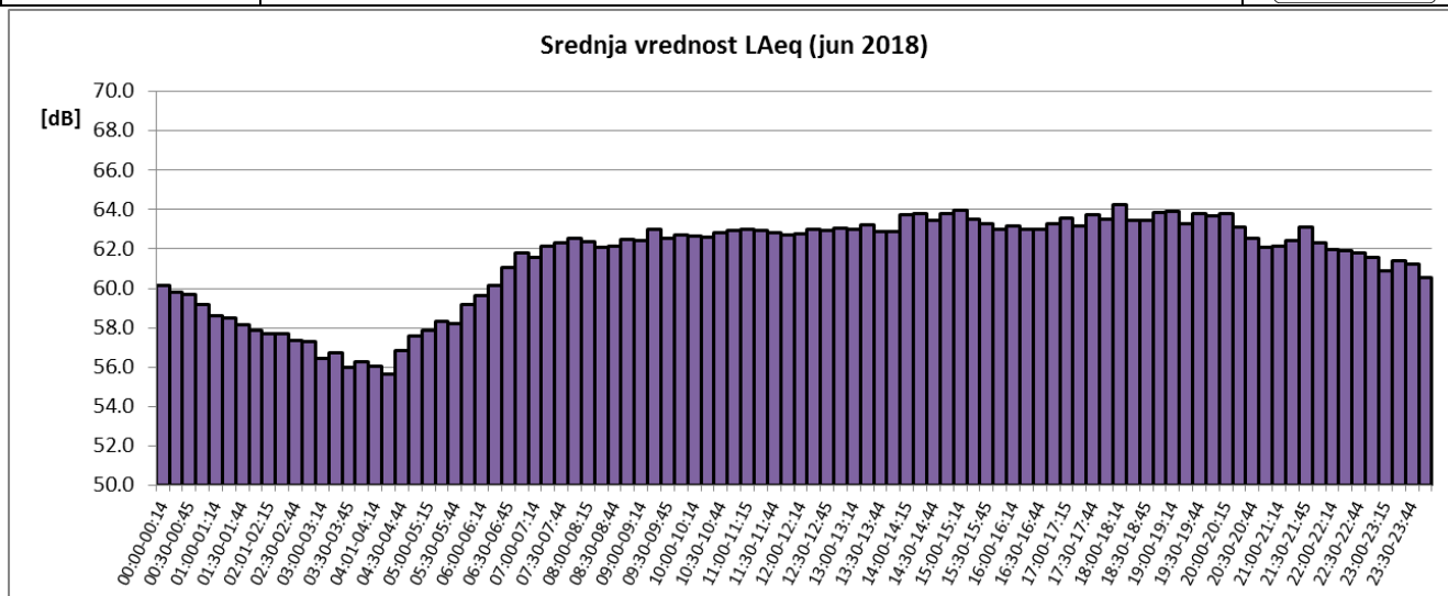
Sl. 6 Promene usrednjenih petnaestominutnih vrednosti ekvivalentnog nivoa buke u toku juna 2018 za NMT-2
