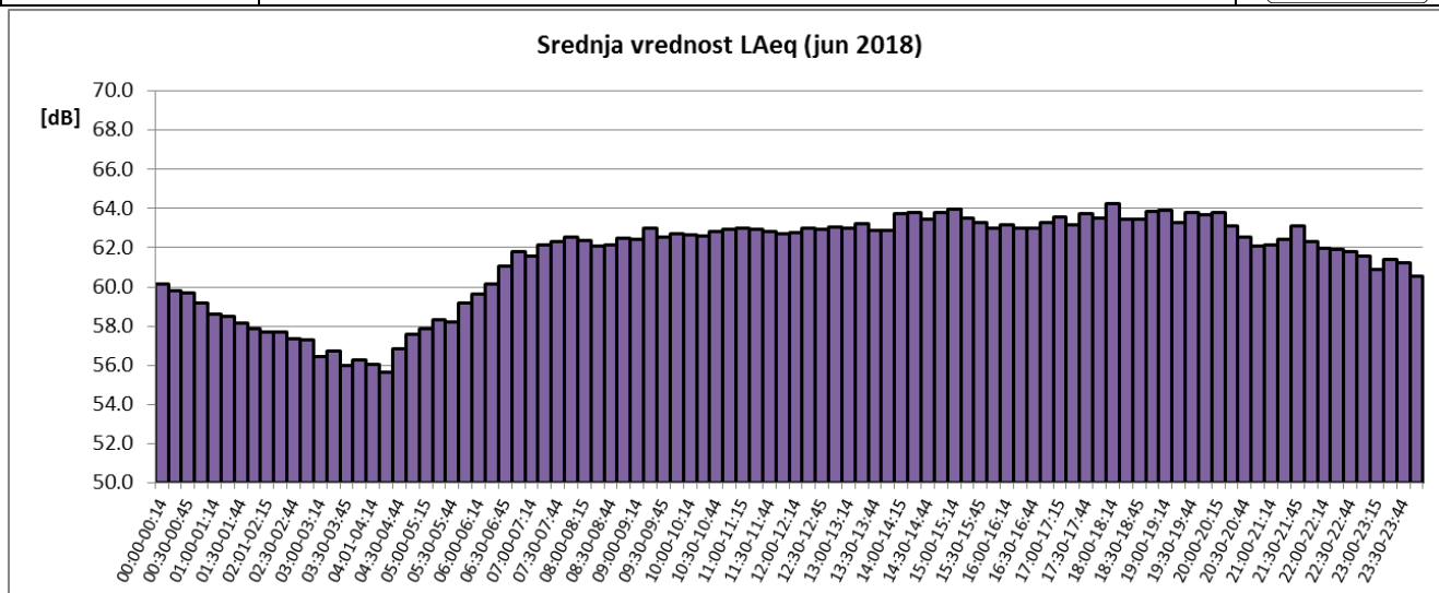
Sl. 5 Promene usrednjenih petnaestominutnih vrednosti ekvivalentnog nivoa buke u toku juna 2018 za NMT-1
