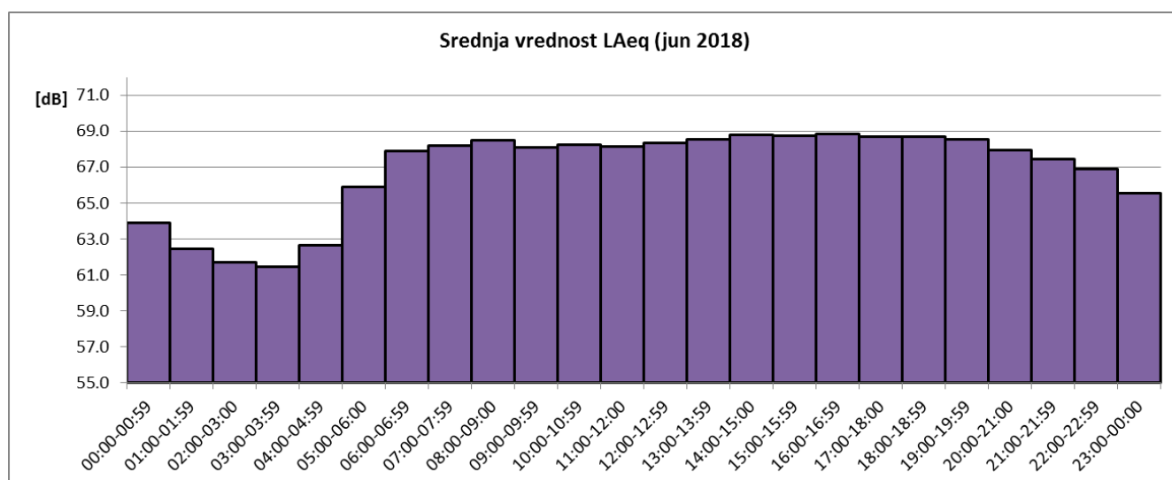
Sl. 4 Promene usrednjenih časovnih vrednosti ekvivalentnog nivoa buke u toku juna 2018 za NMT-2
