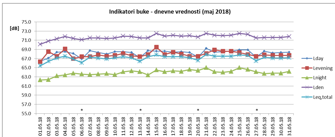
Sl. 2 Promene dnevnih vrednosti indikatora buke u toku maja 2018 za NMT-2
