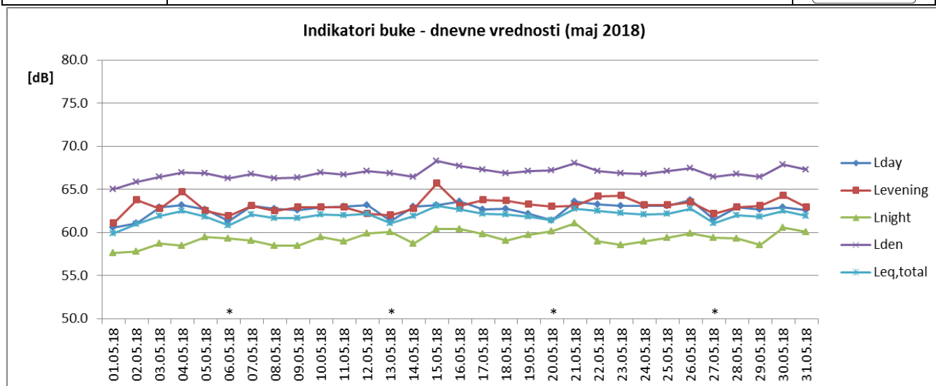
Sl. 1 Promene dnevnih vrednosti indikatora buke u toku maja 2018 za NMT-1
