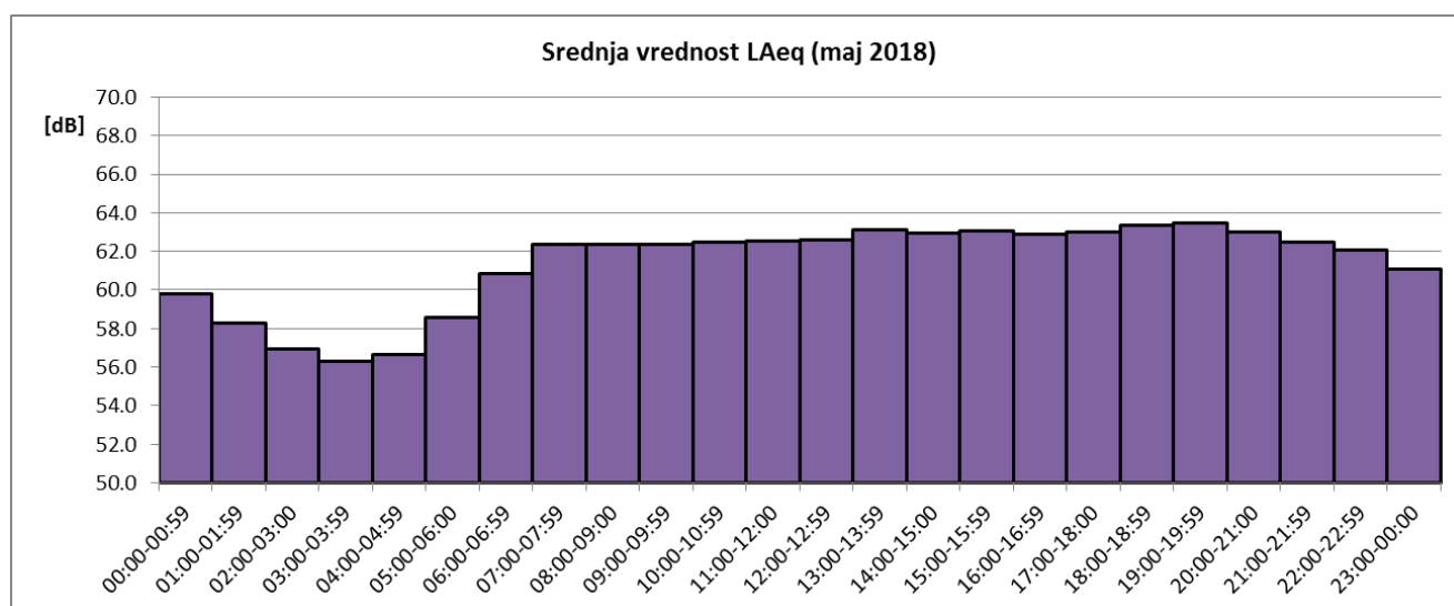
Sl. 3 Promene usrednjenih časovnih vrednosti ekvivalentnog nivoa buke u toku maja 2018 za NMT-1
