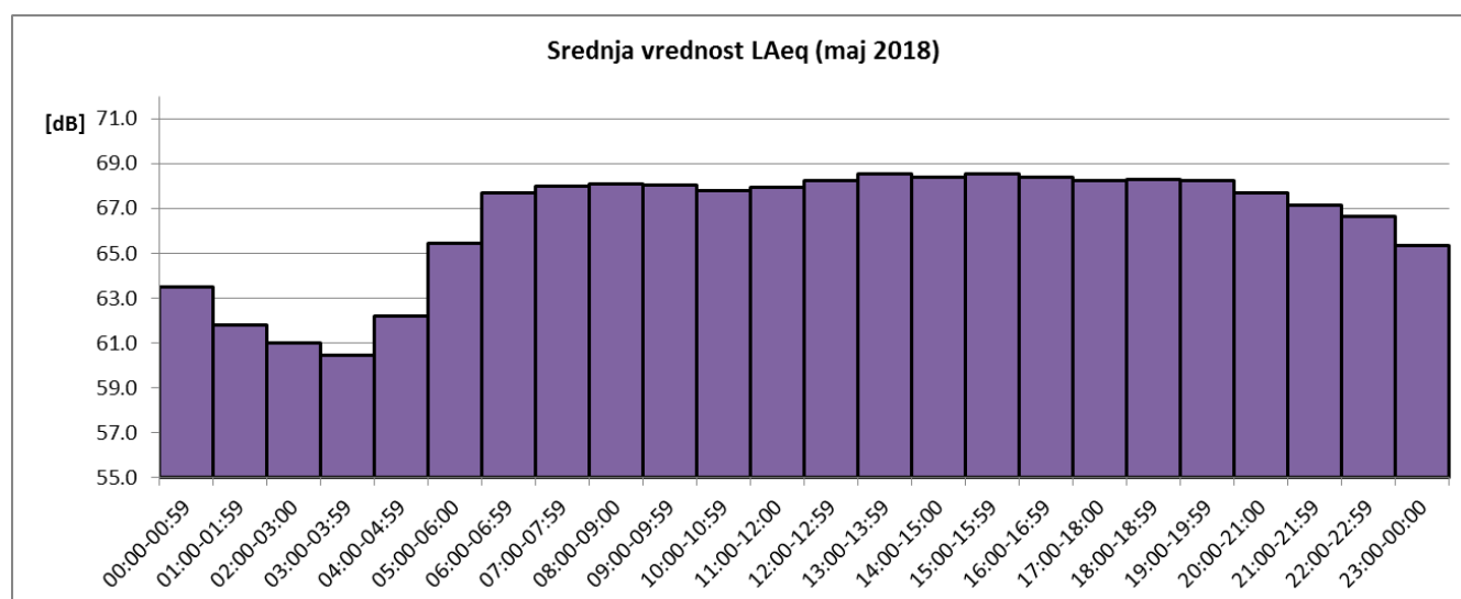
Sl. 4 Promene usrednjenih časovnih vrednosti ekvivalentnog nivoa buke u toku maja 2018 za NMT-2
