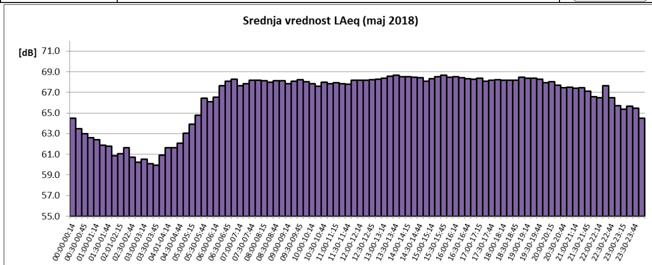
Sl. 6 Promene usrednjenih petnaestominutnih vrednosti ekvivalentnog nivoa buke u toku maja 2018 za NMT-2
