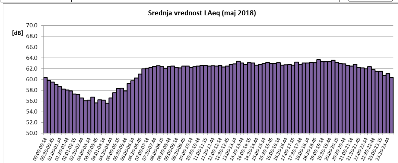
Sl. 5 Promene usrednjenih petnaestominutnih vrednosti ekvivalentnog nivoa buke u toku maja 2018 za NMT-1
