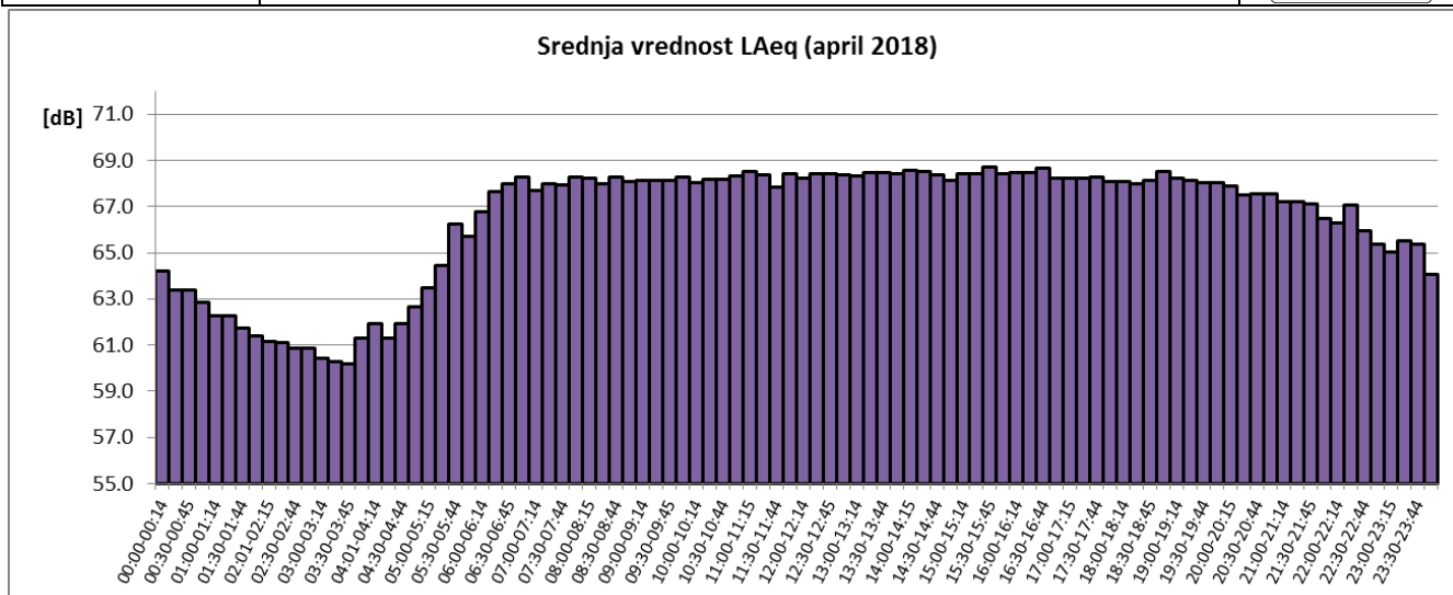
Sl. 6 Promene usrednjenih petnaestominutnih vrednosti ekvivalentnog nivoa buke u toku aprila 2018 za NMT-2
