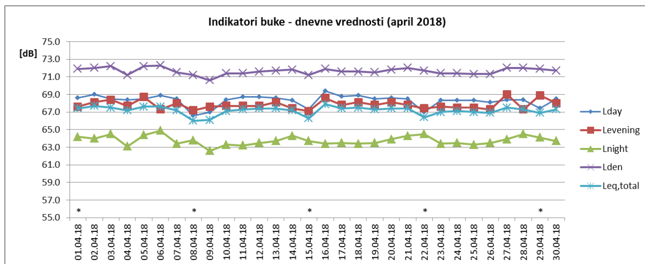
Sl. 2 Promene dnevnih vrednosti indikatora buke u toku aprila 2018 za NMT-2
