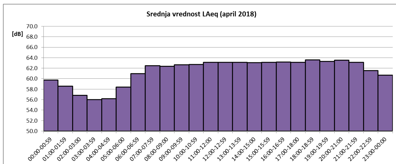
Sl. 3 Promene usrednjenih časovnih vrednosti ekvivalentnog nivoa buke u toku aprila 2018 za NMT-1
