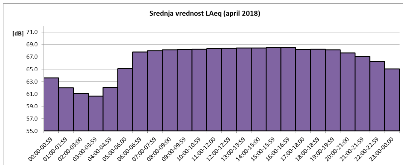
Sl. 4 Promene usrednjenih časovnih vrednosti ekvivalentnog nivoa buke u toku aprila 2018 za NMT-2
