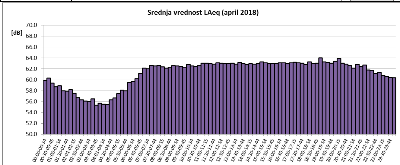
Sl. 5 Promene usrednjenih petnaestominutnih vrednosti ekvivalentnog nivoa buke u toku aprila 2018 za NMT-1
