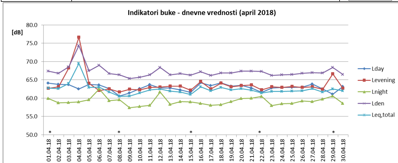
Sl. 1 Promene dnevnih vrednosti indikatora buke u toku aprila 2018 za NMT-1
