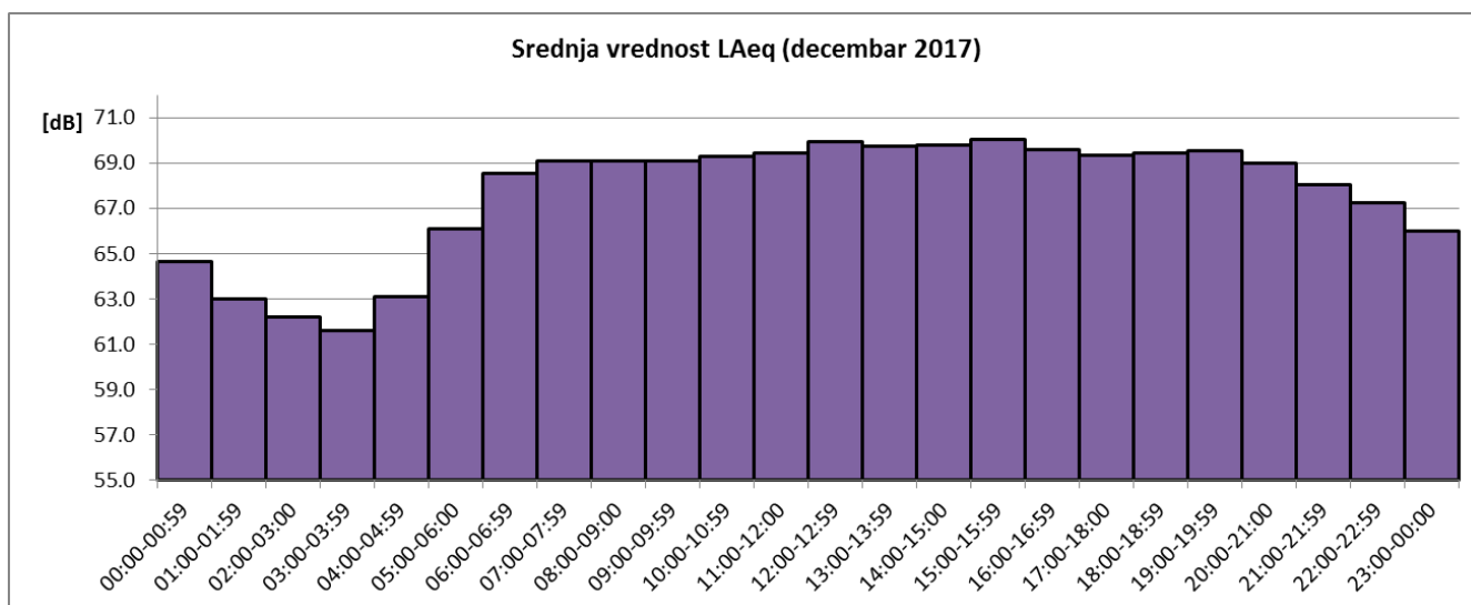
Sl. 4 Promene usrednjenih časovnih vrednosti ekvivalentnog nivoa buke u toku decembra 2017 za NMT-2
