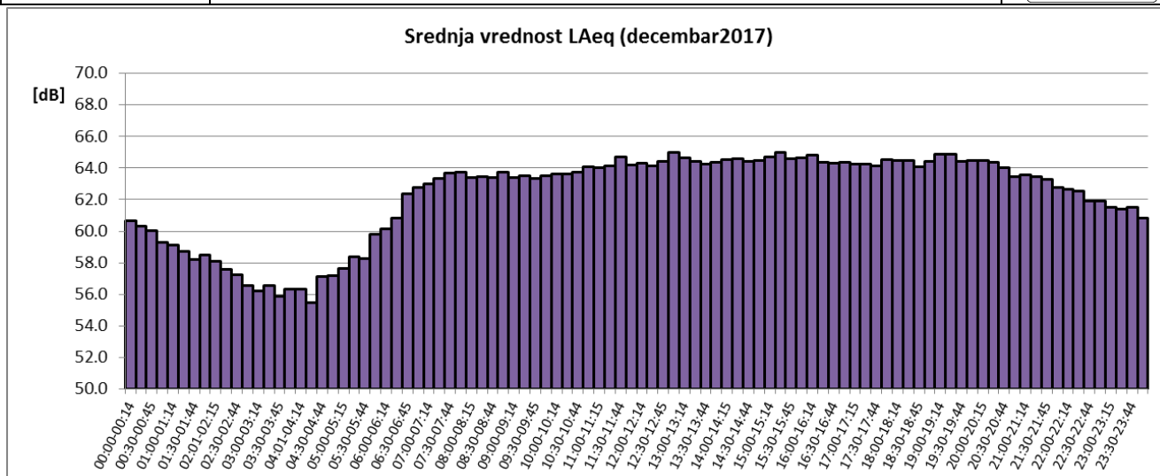
Sl. 5 Promene usrednjenih petnaestominutnih vrednosti ekvivalentnog nivoa buke u toku decembra 2017 za NMT-1
