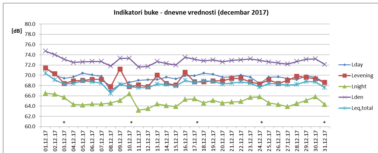
Sl. 2 Promene dnevnih vrednosti indikatora buke u toku decembra 2017 za NMT-2
