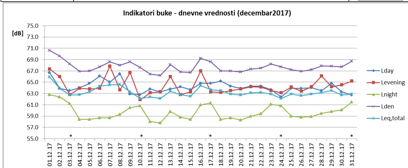
Sl. 1 Promene dnevnih vrednosti indikatora buke u toku decembra 2017 za NMT-1
