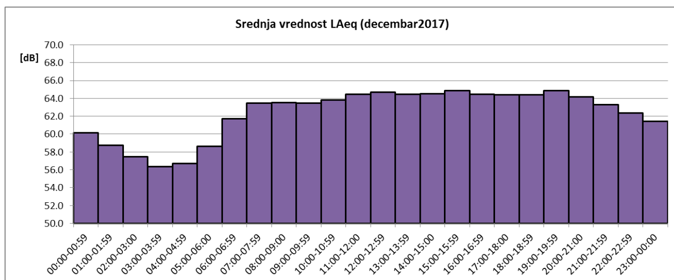
Sl. 3 Promene usrednjenih časovnih vrednosti ekvivalentnog nivoa buke u toku decembra 2017 za NMT-1
