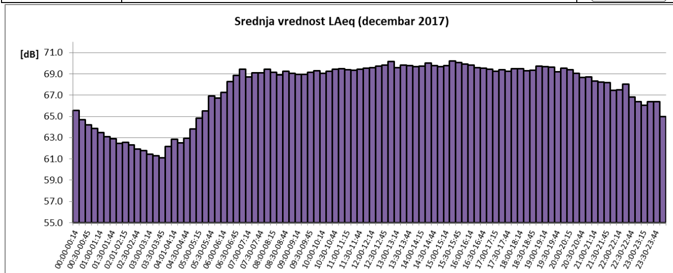
Sl. 6 Promene usrednjenih petnaestominutnih vrednosti ekvivalentnog nivoa buke u toku decembra 2017 za NMT-2
