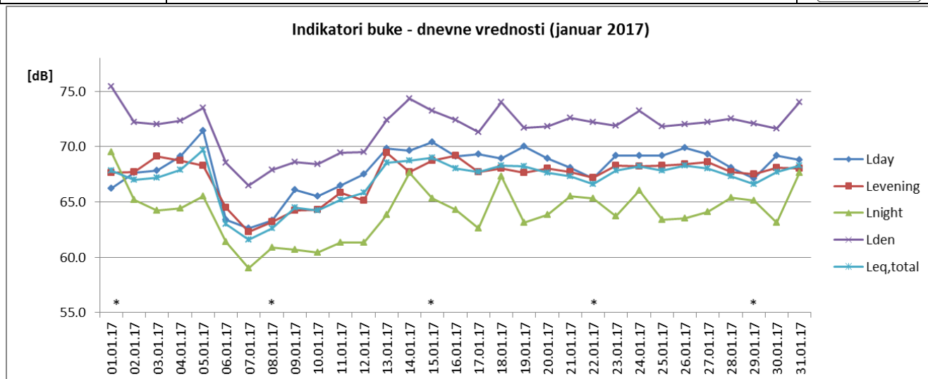
Sl. 1 Promene dnevnih vrednosti indikatora buke u toku januara 2017 za NMT-1
