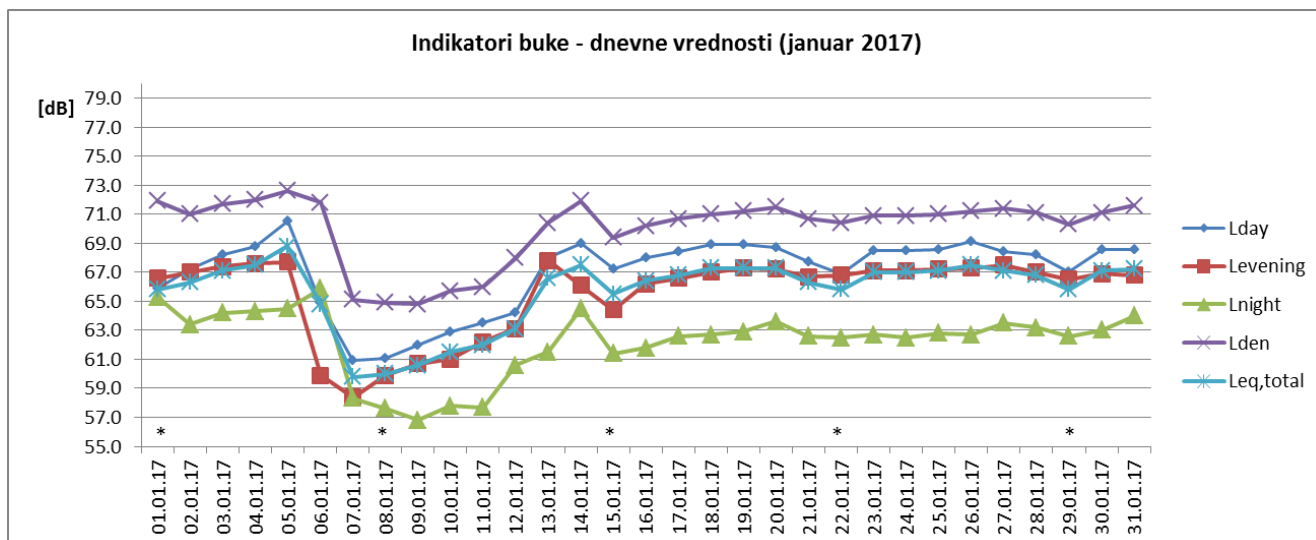
Sl. 2 Promene dnevnih vrednosti indikatora buke u toku januara 2017 za NMT-2
