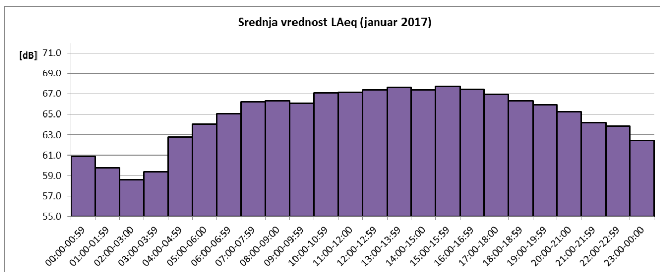
Sl. 4 Promene usrednjenih časovnih vrednosti ekvivalentnog nivoa buke u toku januara 2017 za NMT-2
