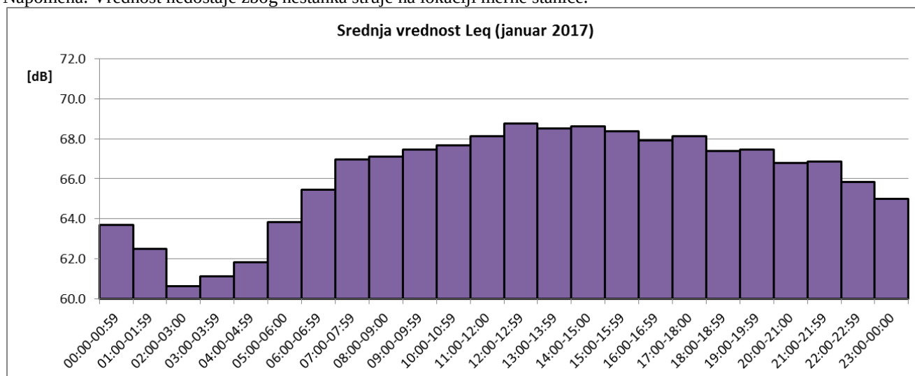
Sl. 3 Promene usrednjenih časovnih vrednosti ekvivalentnog nivoa buke u toku januara 2017 za NMT-1
