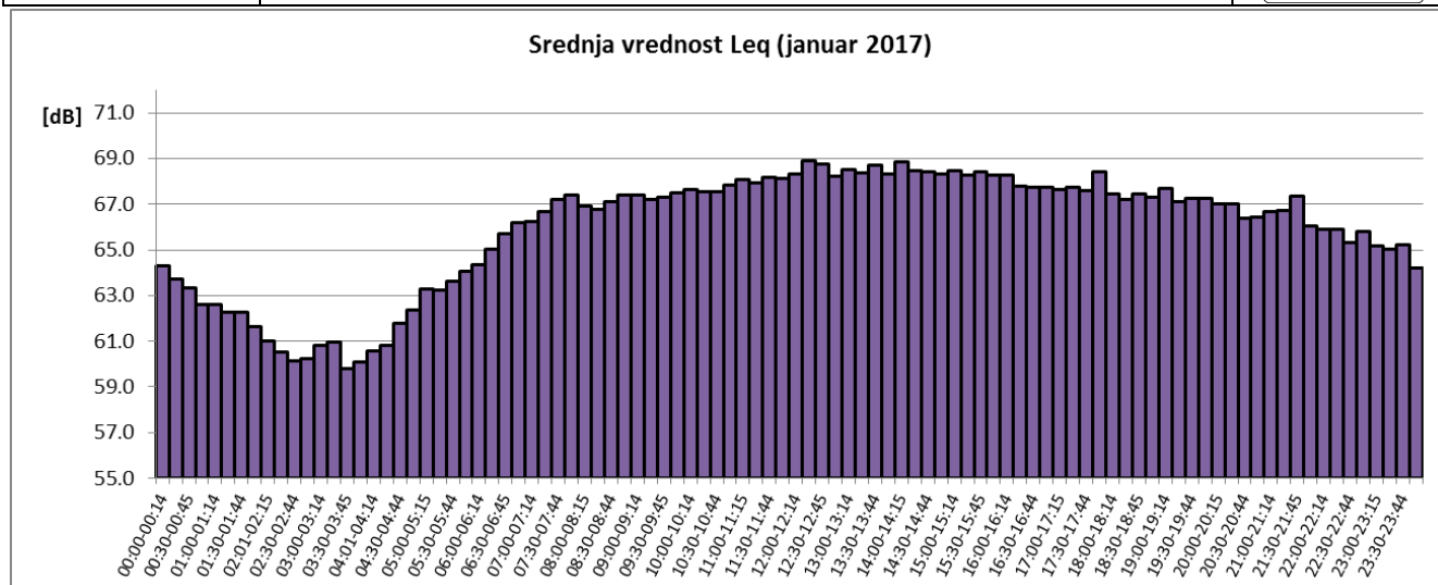
Sl. 5 Promene usrednjenih petnaestominutnih vrednosti ekvivalentnog nivoa buke u toku januara 2017 za NMT-1
