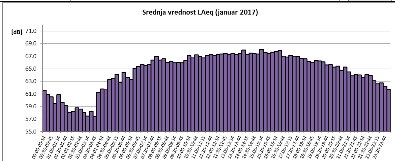
Sl. 6 Promene usrednjenih petnaestominutnih vrednosti ekvivalentnog nivoa buke u toku januara 2017 za NMT-2
