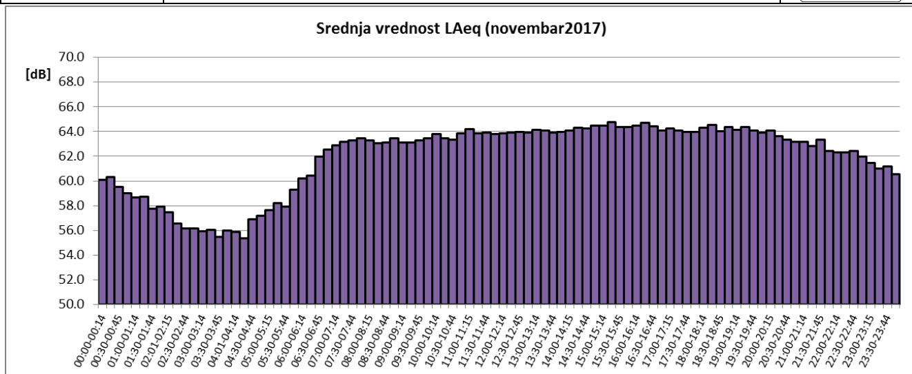
Sl. 5 Promene usrednjenih petnaestominutnih vrednosti ekvivalentnog nivoa buke u toku novembra 2017 za NMT-1
