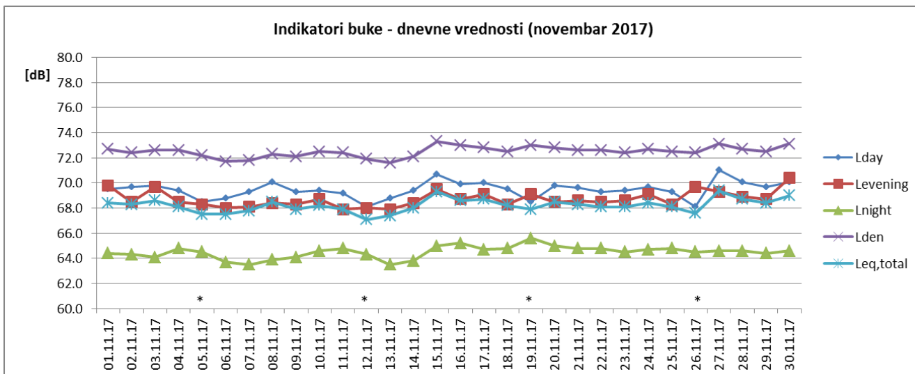
Sl. 2 Promene dnevnih vrednosti indikatora buke u toku novembra 2017 za NMT-2
