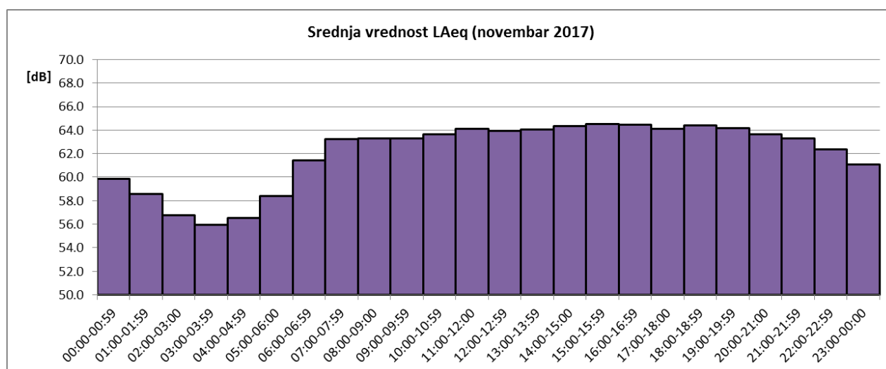
Sl. 3 Promene usrednjenih časovnih vrednosti ekvivalentnog nivoa buke u toku novembra 2017 za NMT-1
