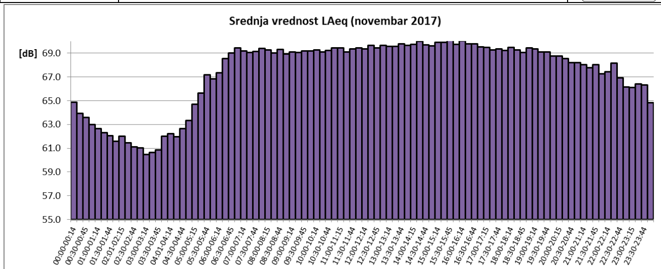
Sl. 6 Promene usrednjenih petnaestominutnih vrednosti ekvivalentnog nivoa buke u toku novembra 2017 za NMT-2
