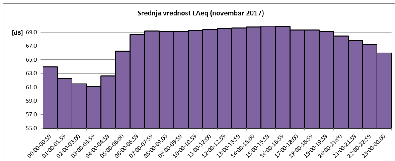
Sl. 4 Promene usrednjenih časovnih vrednosti ekvivalentnog nivoa buke u toku novembra 2017 za NMT-2
