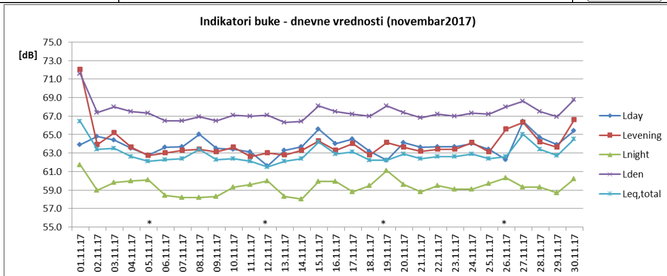
Sl. 1 Promene dnevnih vrednosti indikatora buke u toku novembra 2017 za NMT-1
