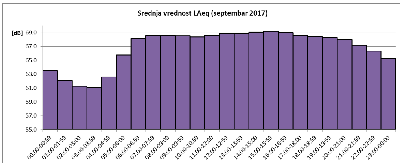
Sl. 4 Promene usrednjenih časovnih vrednosti ekvivalentnog nivoa buke u toku septembra 2017 za NMT-2
