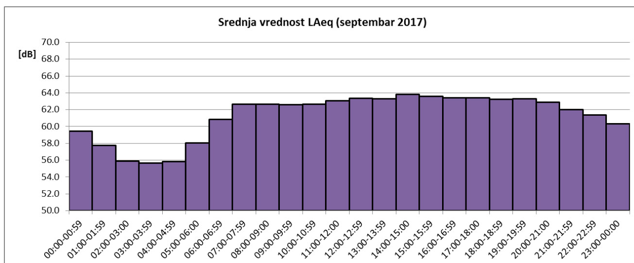
Sl. 3 Promene usrednjenih časovnih vrednosti ekvivalentnog nivoa buke u toku septembra 2017 za NMT-1
