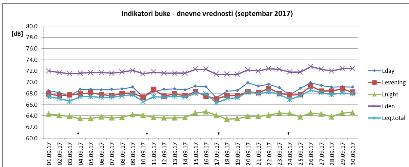
Sl. 2 Promene dnevnih vrednosti indikatora buke u toku septembra 2017 za NMT-2
