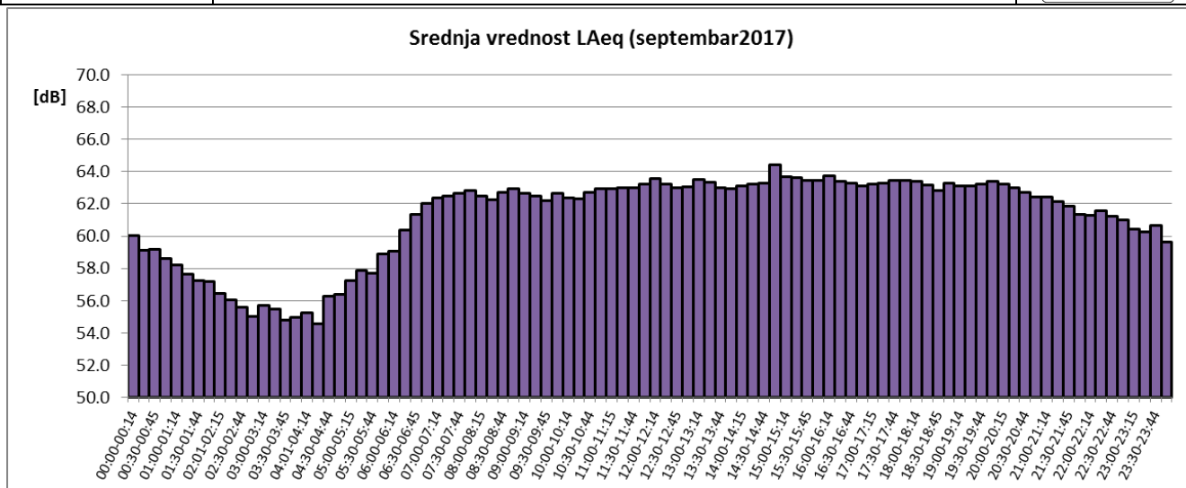
Sl. 5 Promene usrednjenih petnaestominutnih vrednosti ekvivalentnog nivoa buke u toku septembra 2017 za NMT-1
