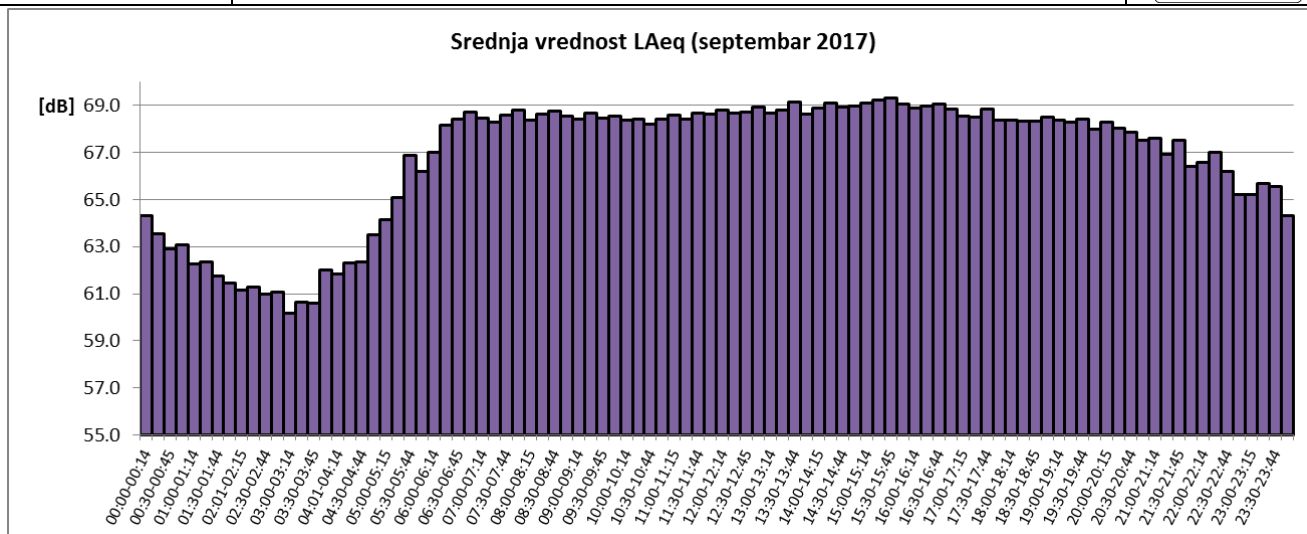
Sl. 6 Promene usrednjenih petnaestominutnih vrednosti ekvivalentnog nivoa buke u toku septembra 2017 za NMT-2
