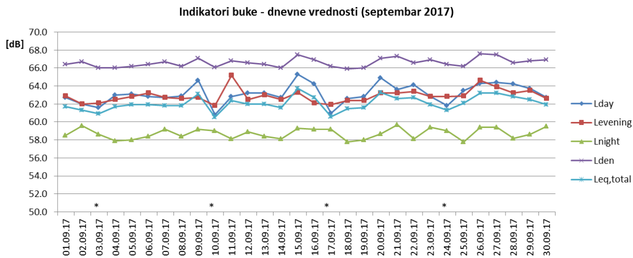
Sl. 1 Promene dnevnih vrednosti indikatora buke u toku septembra 2017 za NMT-1
