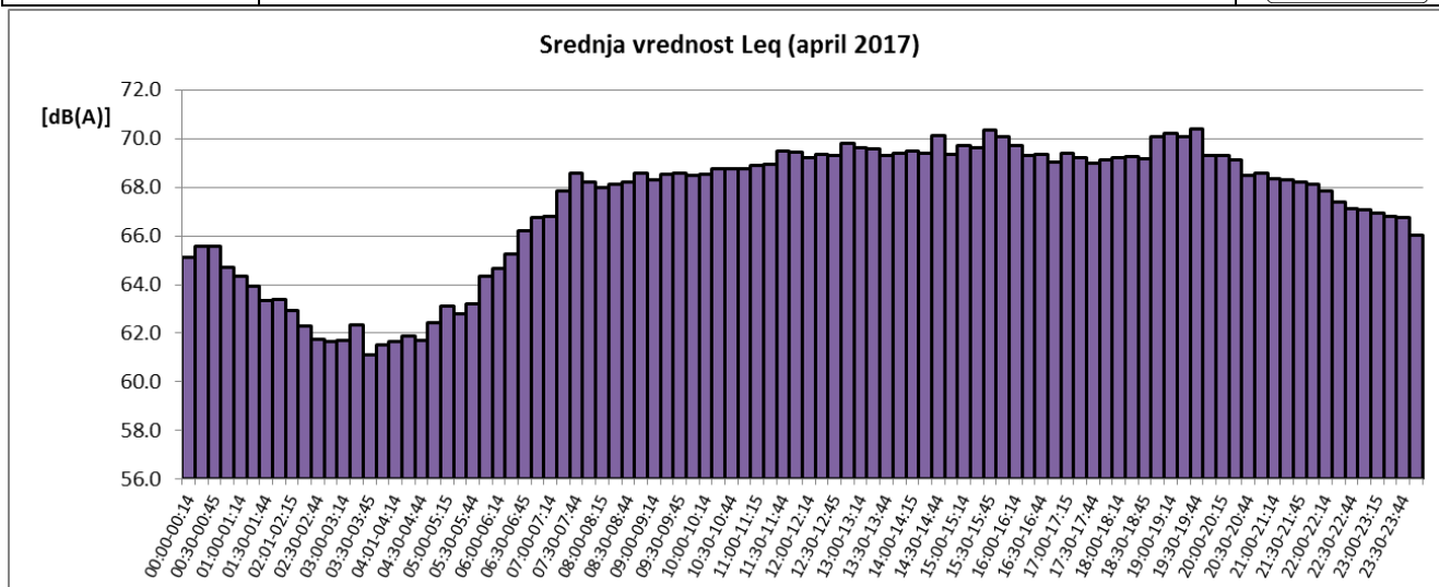
Sl. 5 Promene usrednjenih petnaestominutnih vrednosti ekvivalentnog nivoa buke u toku aprila 2017 za NMT-1
