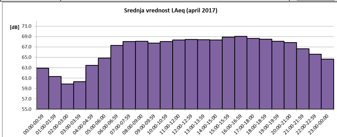
Sl. 6 Promene usrednjenih petnaestominutnih vrednosti ekvivalentnog nivoa buke u toku aprila 2017 za NMT-2
