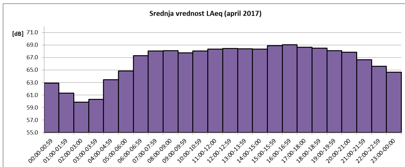
Sl. 4 Promene usrednjenih časovnih vrednosti ekvivalentnog nivoa buke u toku aprila 2017 za NMT-2
