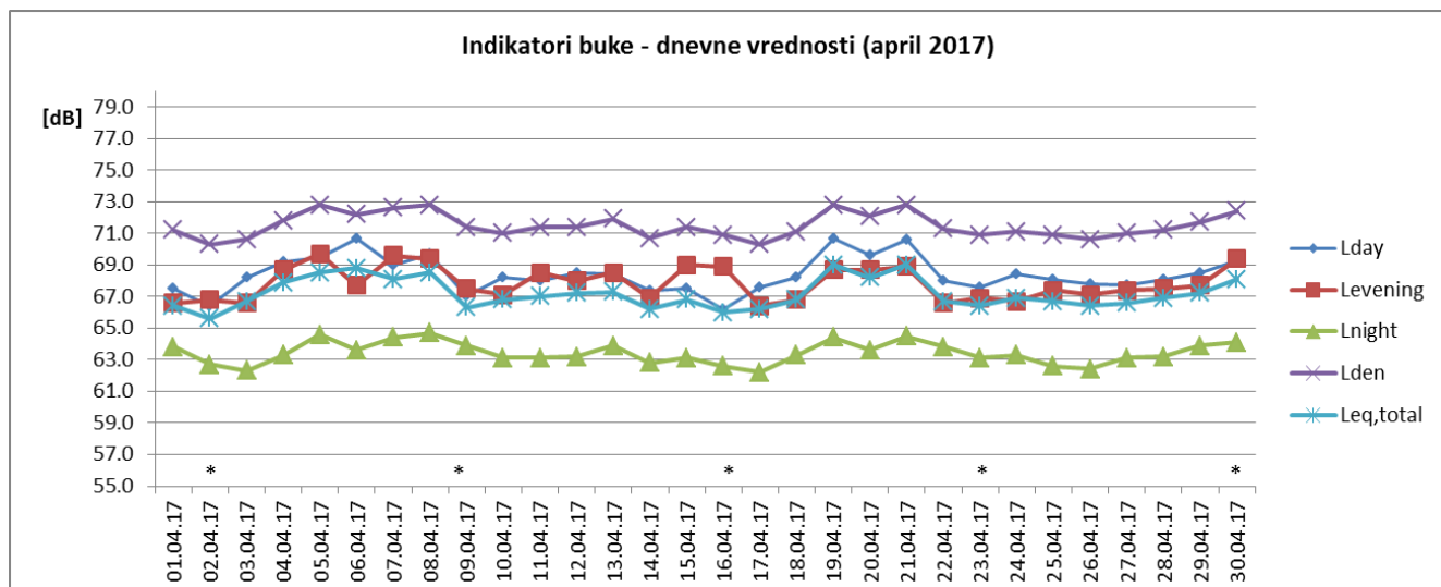
Sl. 2 Promene dnevnih vrednosti indikatora buke u toku aprila 2017 za NMT-2
