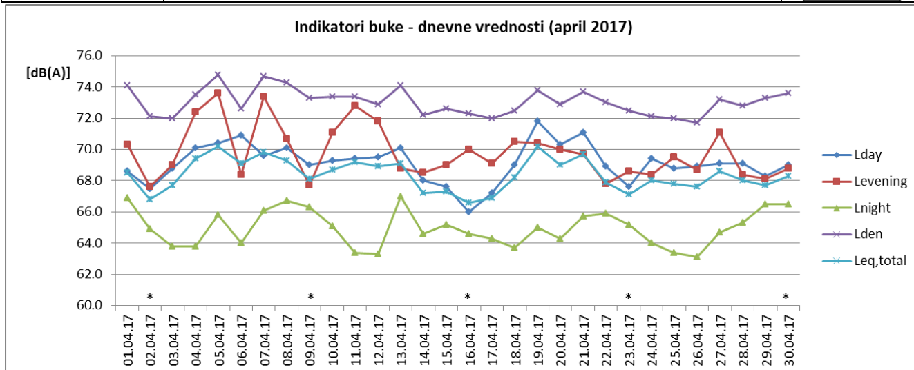
Sl. 1 Promene dnevnih vrednosti indikatora buke u toku aprila 2017 za NMT-1
