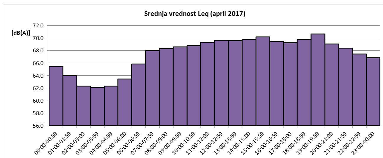
Sl. 3 Promene usrednjenih časovnih vrednosti ekvivalentnog nivoa buke u toku aprila 2017 za NMT-1
