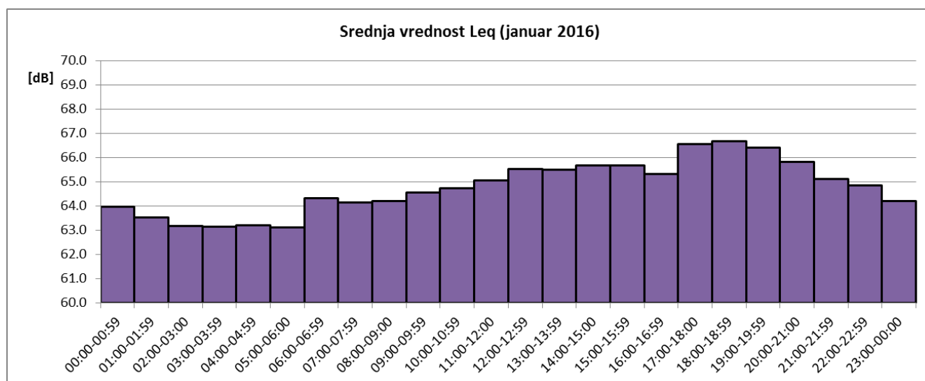
Sl. 4 Promene usrednjenih časovnih vrednosti ekvivalentnog nivoa buke u toku januara 2016 za NMT-2
