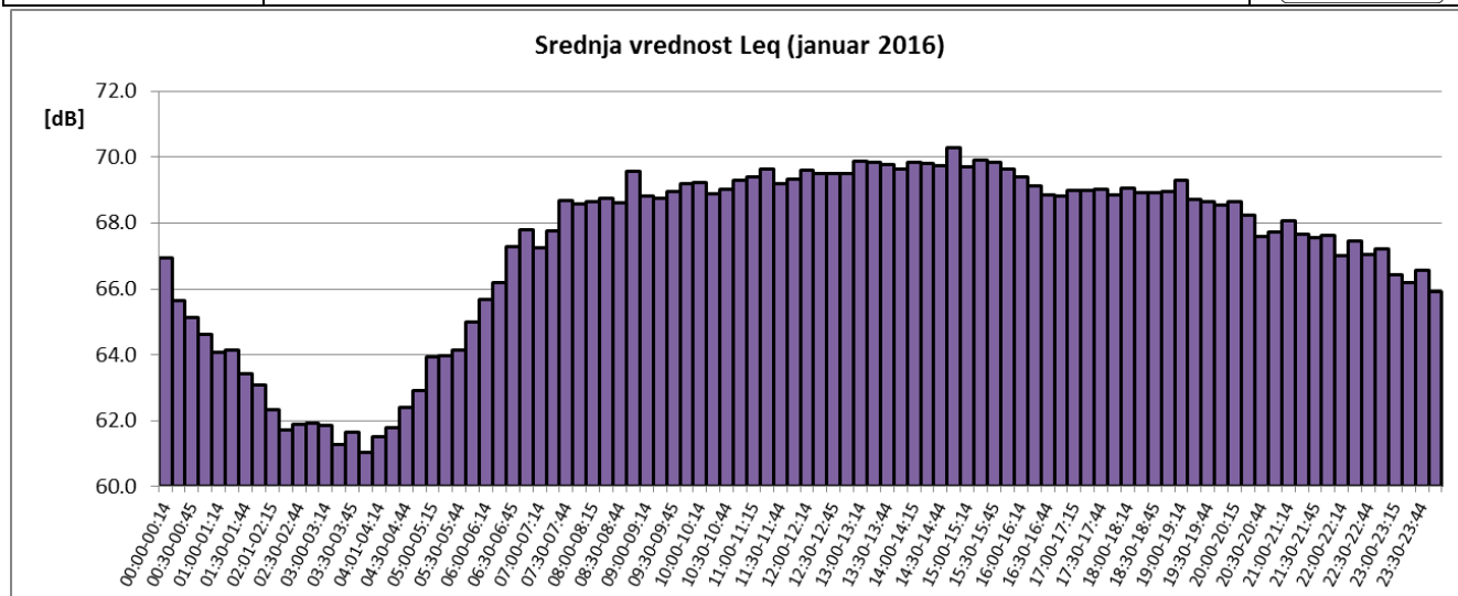
Sl. 5 Promene usrednjenih petnaestominutnih vrednosti ekvivalentnog nivoa buke u toku januara 2016 za NMT-1
