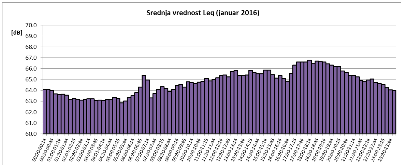
Sl. 6 Promene usrednjenih petnaestominutnih vrednosti ekvivalentnog nivoa buke u toku januara 2016 za NMT-2
