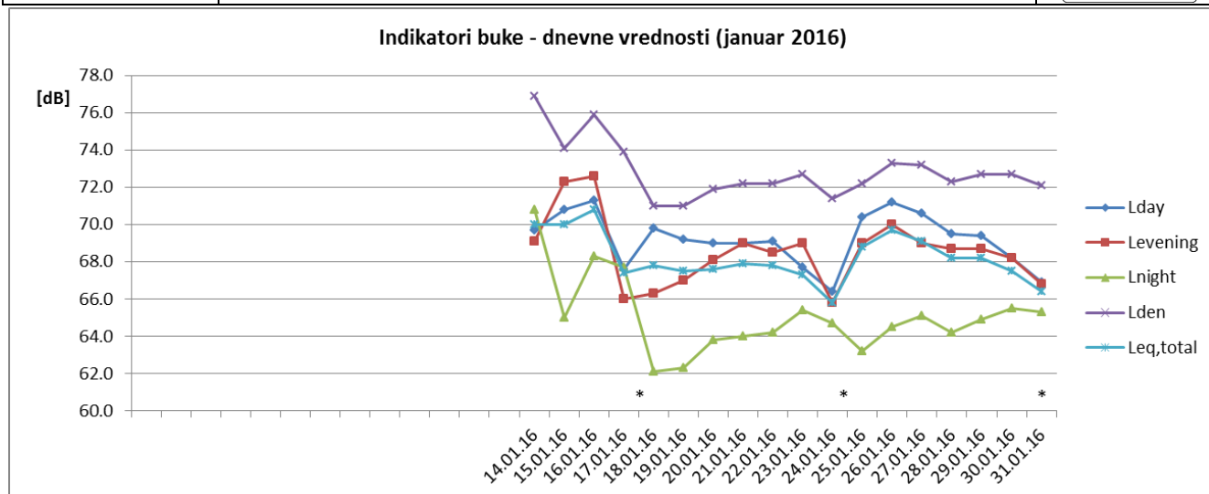
Sl. 1 Promene dnevnih vrednosti indikatora buke u toku januara 2016 za NMT-1
