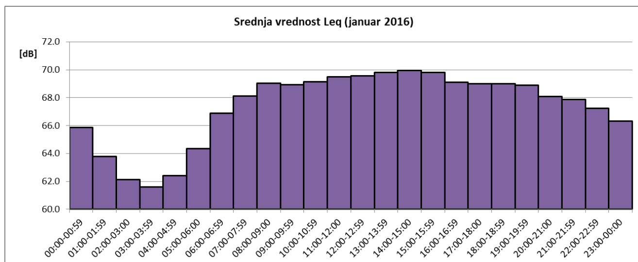
Sl. 3 Promene usrednjenih časovnih vrednosti ekvivalentnog nivoa buke u toku januara 2016 za NMT-1
