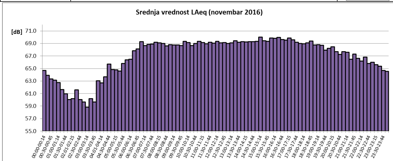
Sl. 6 Promene usrednjenih petnaestominutnih vrednosti ekvivalentnog nivoa buke u toku novembra 2016 za NMT-2
