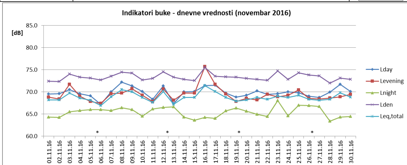
Sl. 1 Promene dnevnih vrednosti indikatora buke u toku novembra 2016 za NMT-1
