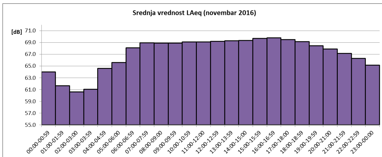
Sl. 4 Promene usrednjenih časovnih vrednosti ekvivalentnog nivoa buke u toku novembra 2016 za NMT-2
