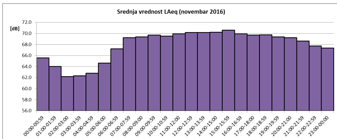
Sl. 3 Promene usrednjenih časovnih vrednosti ekvivalentnog nivoa buke u toku novembra 2016 za NMT-1
