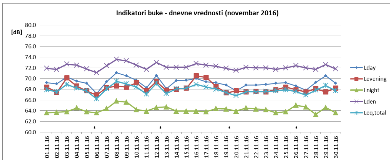
Sl. 2 Promene dnevnih vrednosti indikatora buke u toku novembra 2016 za NMT-2
