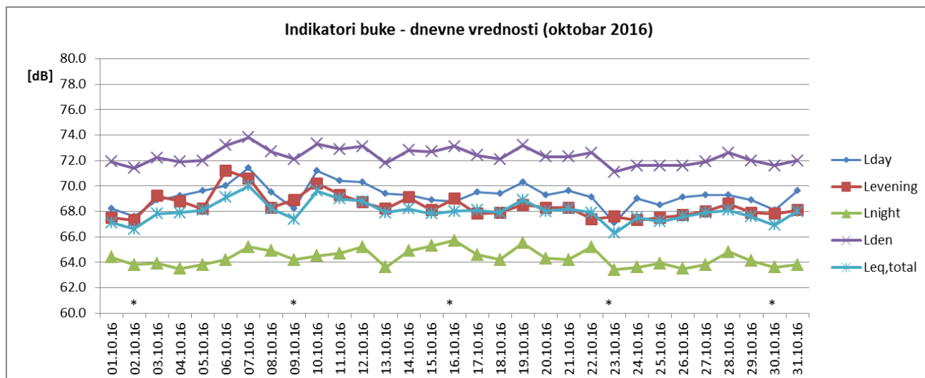
Sl. 2 Promene dnevnih vrednosti indikatora buke u toku oktobra 2016 za NMT-2
