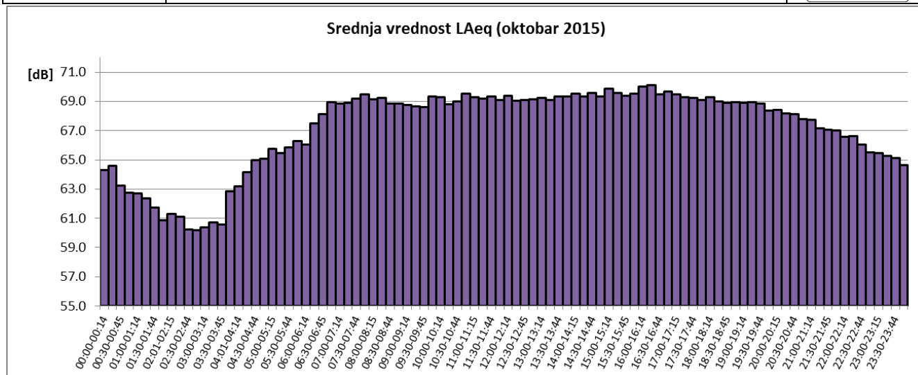
Sl. 6 Promene usrednjenih petnaestominutnih vrednosti ekvivalentnog nivoa buke u toku oktobra 2016 za NMT-2
