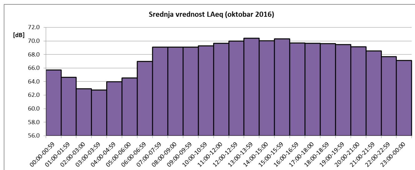
Sl. 3 Promene usrednjenih časovnih vrednosti ekvivalentnog nivoa buke u toku oktobra 2016 za NMT-1
