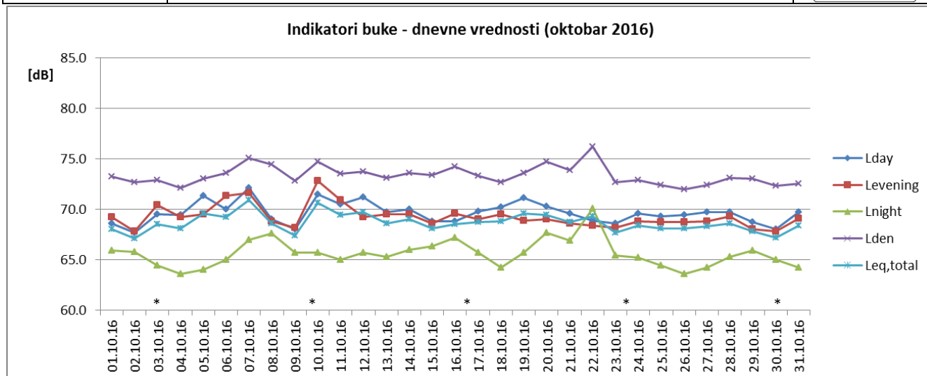
Sl. 1 Promene dnevnih vrednosti indikatora buke u toku oktobra 2016 za NMT-1
