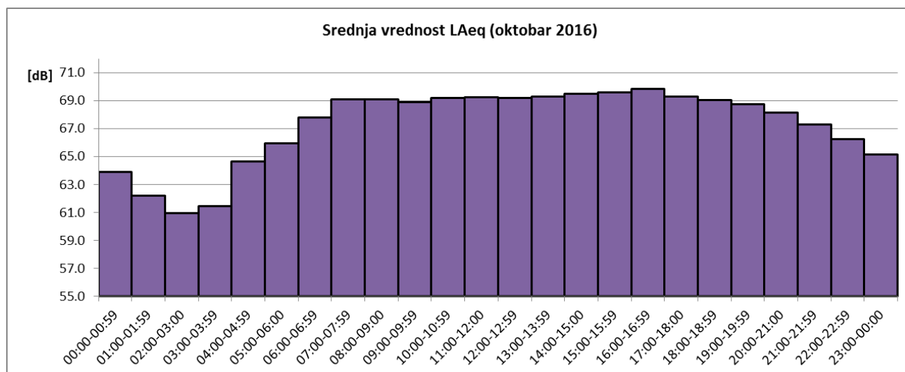
Sl. 4 Promene usrednjenih časovnih vrednosti ekvivalentnog nivoa buke u toku oktobra 2016 za NMT-2
