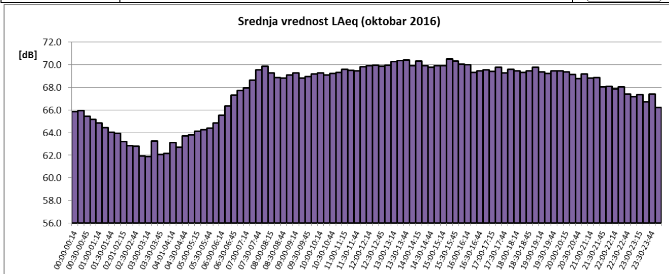
Sl. 5 Promene usrednjenih petnaestominutnih vrednosti ekvivalentnog nivoa buke u toku oktobra 2016 za NMT-1
