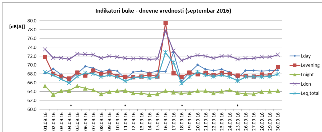
Sl. 2 Promene dnevnih vrednosti indikatora buke u toku septembra 2016 za NMT-2
