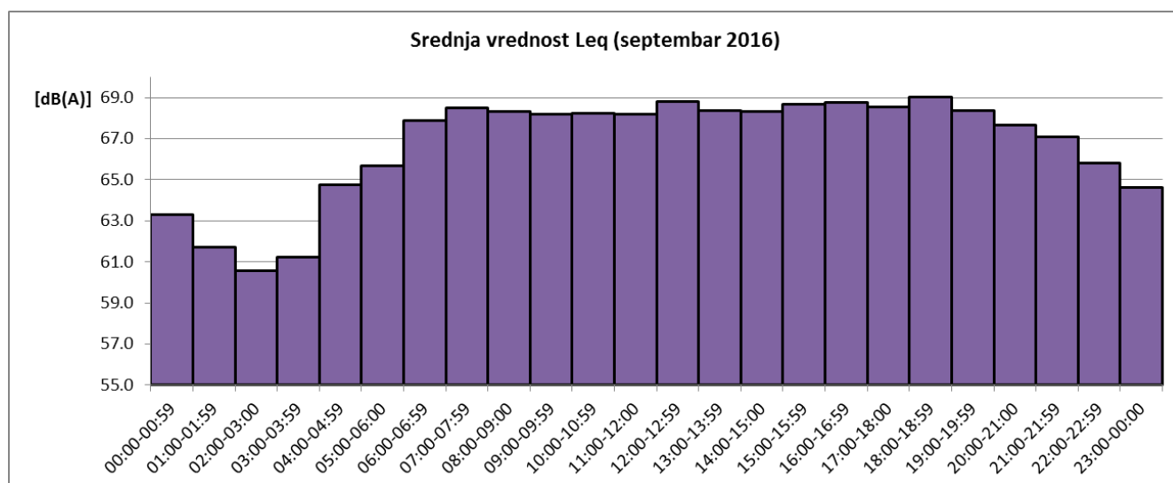
Sl. 4 Promene usrednjenih časovnih vrednosti ekvivalentnog nivoa buke u toku septembra 2016 za NMT-2
