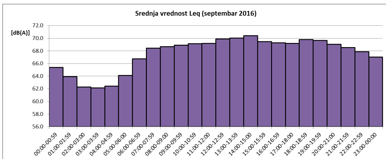
Sl. 3 Promene usrednjenih časovnih vrednosti ekvivalentnog nivoa buke u toku septembra 2016 za NMT-1
