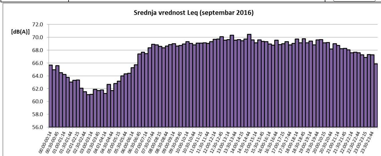
Sl. 5 Promene usrednjenih petnaestominutnih vrednosti ekvivalentnog nivoa buke u toku septembra 2016 za NMT-1
