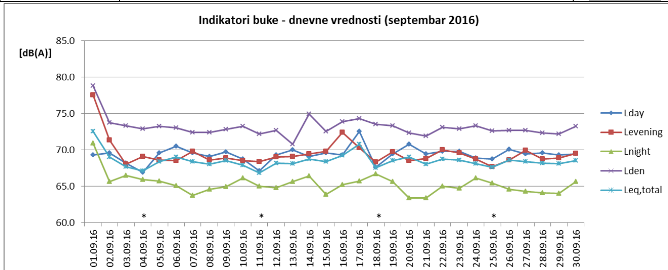
Sl. 1 Promene dnevnih vrednosti indikatora buke u toku septembra 2016 za NMT-1
