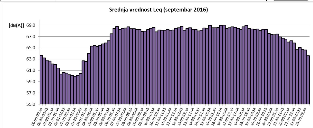
Sl. 6 Promene usrednjenih petnaestominutnih vrednosti ekvivalentnog nivoa buke u toku septembra 2016 za NMT-2
