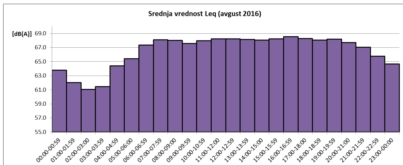
Sl. 4 Promene usrednjenih časovnih vrednosti ekvivalentnog nivoa buke u toku avgusta 2016 za NMT-2
