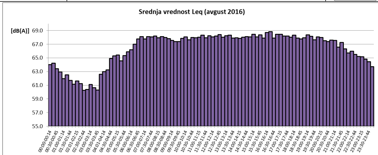
Sl. 6 Promene usrednjenih petnaestominutnih vrednosti ekvivalentnog nivoa buke u toku avgusta 2016 za NMT-2
