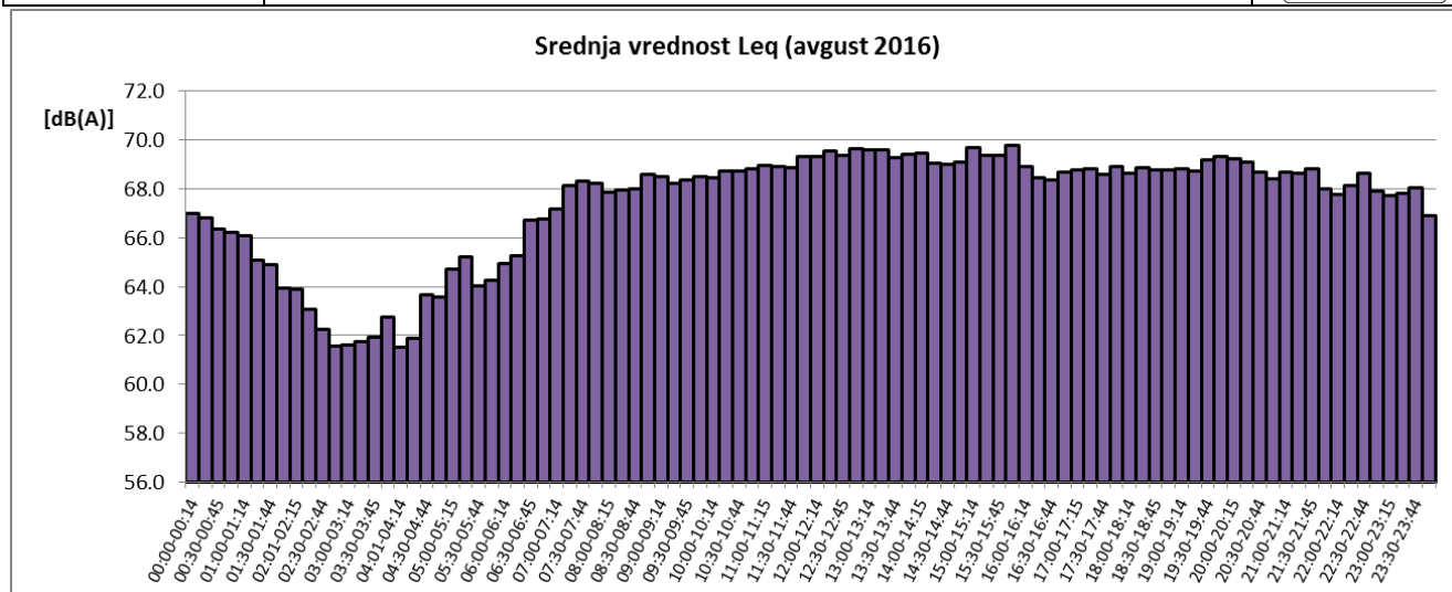
Sl. 5 Promene usrednjenih petnaestominutnih vrednosti ekvivalentnog nivoa buke u toku avgusta 2016 za NMT-1
