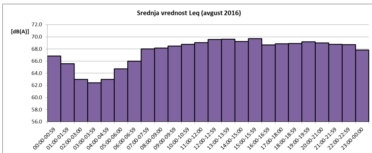
Sl. 3 Promene usrednjenih časovnih vrednosti ekvivalentnog nivoa buke u toku avgusta 2016 za NMT-1
