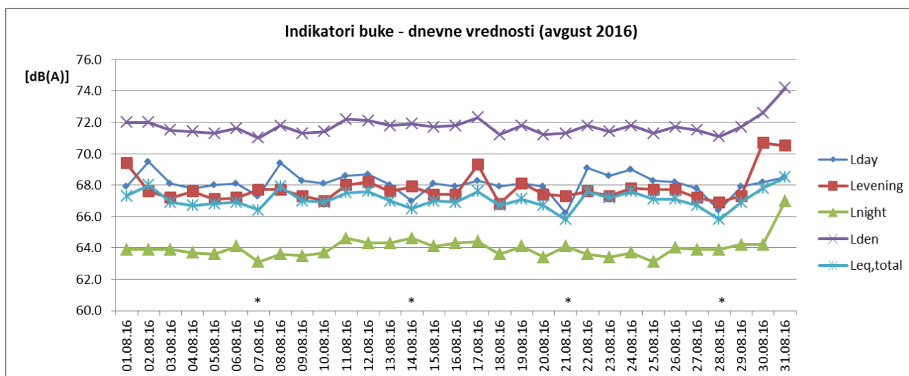
Sl. 2 Promene dnevnih vrednosti indikatora buke u toku avgusta 2016 za NMT-2
