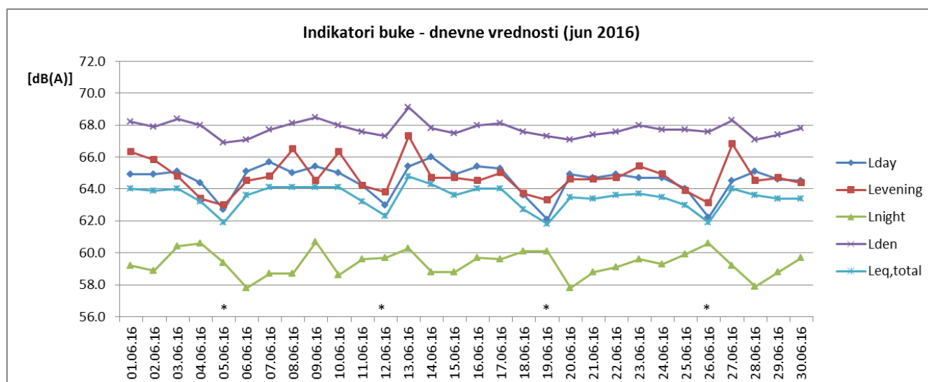
SI. 2 Promene dnevnih vrednosti indikatora buke u toku juna 2016 za NMT-2
