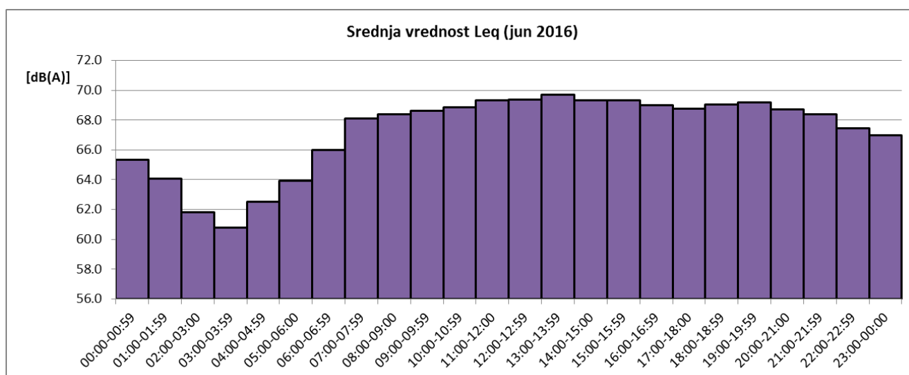
Sl. 3 Promene usrednjenih časovnih vrednosti ekvivalentnog nivoa buke u toku juna 2016 za NMT-1
