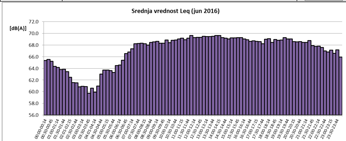
Sl. 5 Promene usrednjenih petnaestominutnih vrednosti ekvivalentnog nivoa buke u toku juna 2016 za NMT-1
