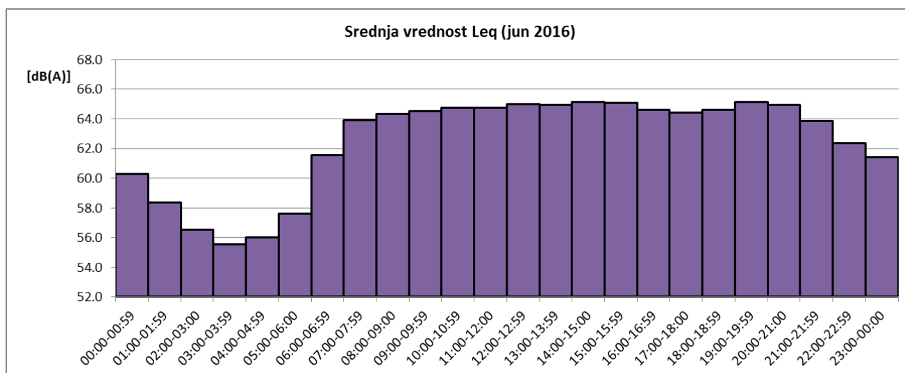
Sl. 4 Promene usrednjenih časovnih vrednosti ekvivalentnog nivoa buke u toku juna 2016 za NMT-2
