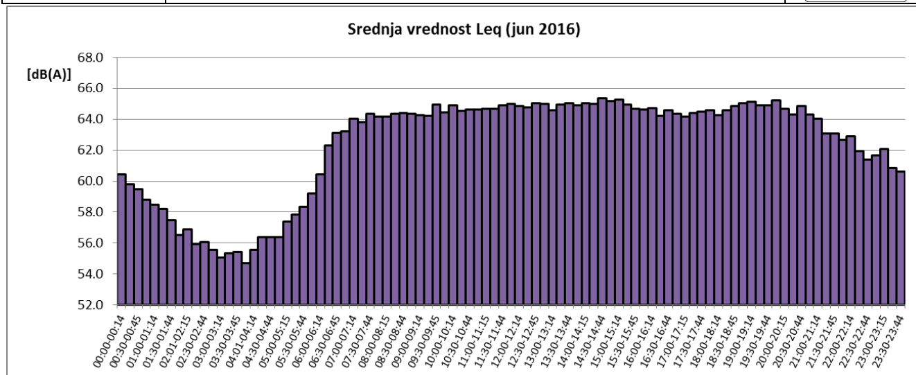
Sl. 6 Promene usrednjenih petnaestominutnih vrednosti ekvivalentnog nivoa buke u toku juna 2016 za NMT-2
