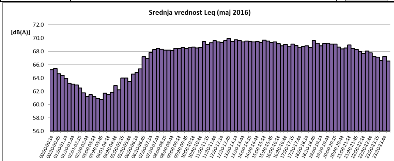
Sl. 5 Promene usrednjenih petnaestominutnih vrednosti ekvivalentnog nivoa buke u toku maja 2016 za NMT-1
