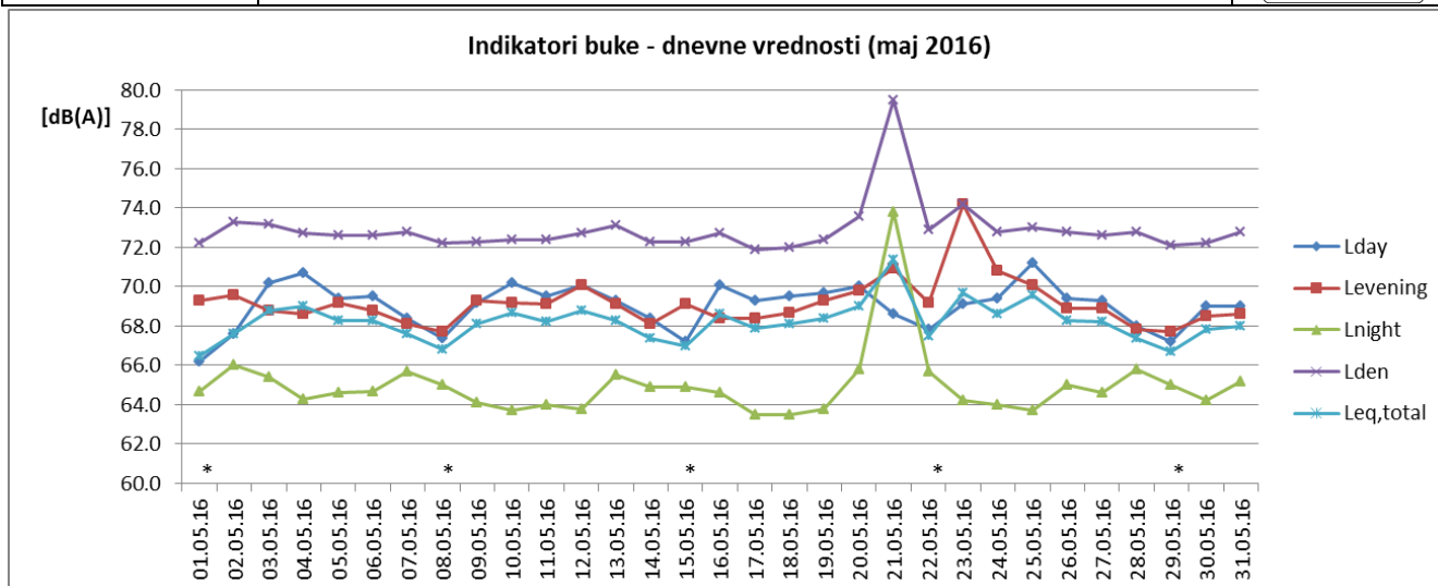
Sl. 1 Promene dnevnih vrednosti indikatora buke u toku maja 2016 za NMT-1
