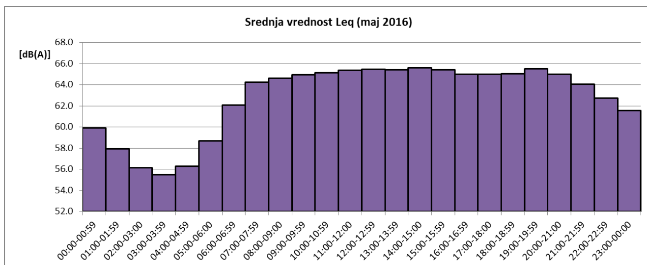
Sl. 4 Promene usrednjenih časovnih vrednosti ekvivalentnog nivoa buke u toku maja 2016 za NMT-2
