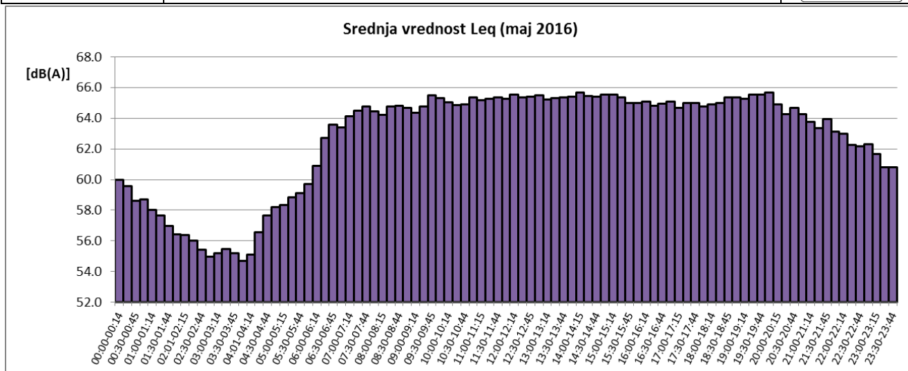
Sl. 6 Promene usrednjenih petnaestominutnih vrednosti ekvivalentnog nivoa buke u toku maja 2016 za NMT-2
