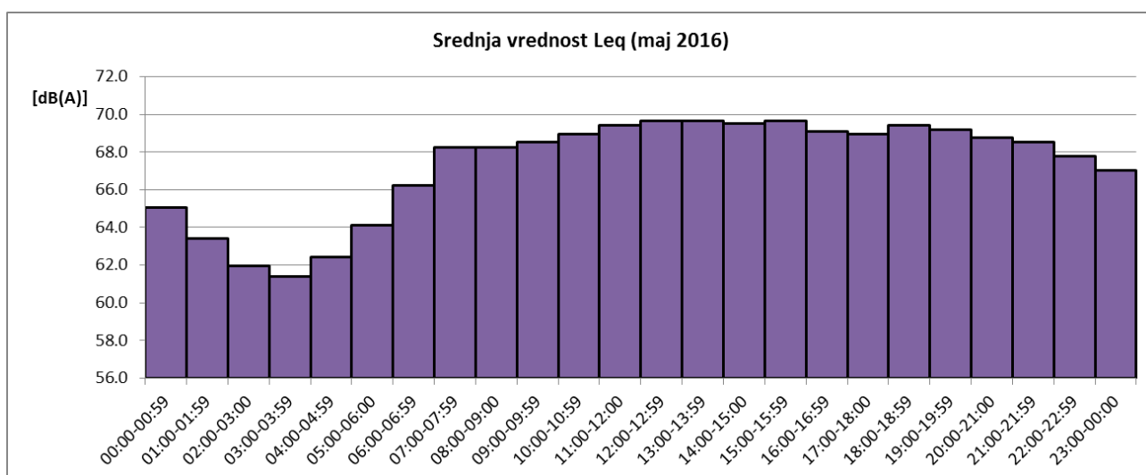
Sl. 3 Promene usrednjenih časovnih vrednosti ekvivalentnog nivoa buke u toku maja 2016 za NMT-1
