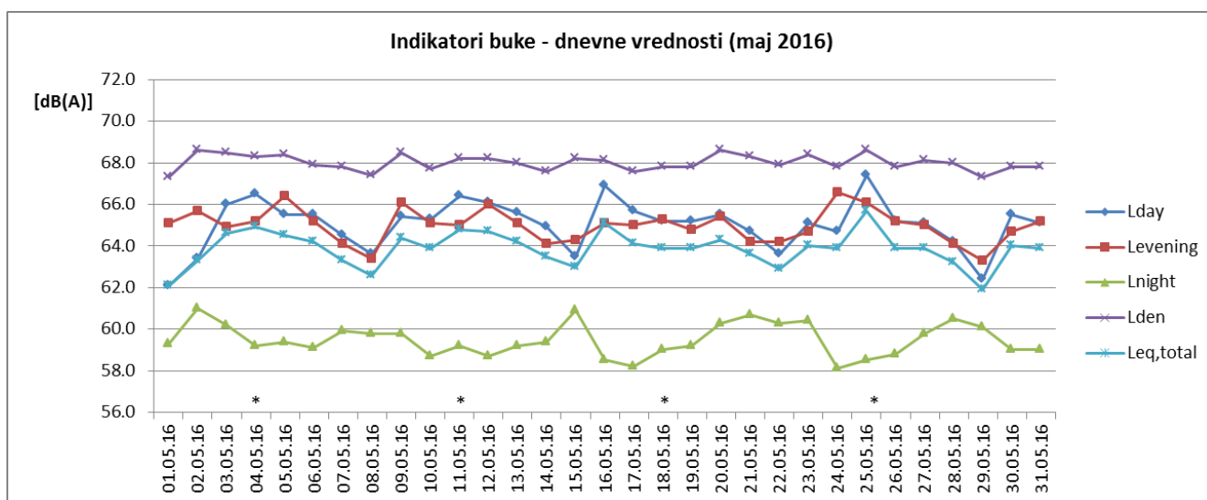
Sl. 2 Promene dnevnih vrednosti indikatora buke u toku maja 2016 za NMT-2
