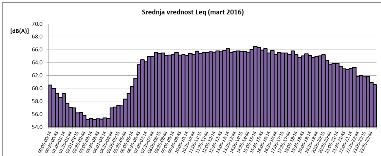
Sl. 6 Promene usrednjenih petnaestominutnih vrednosti ekvivalentnog nivoa buke u toku marta 2016 za NMT-2
