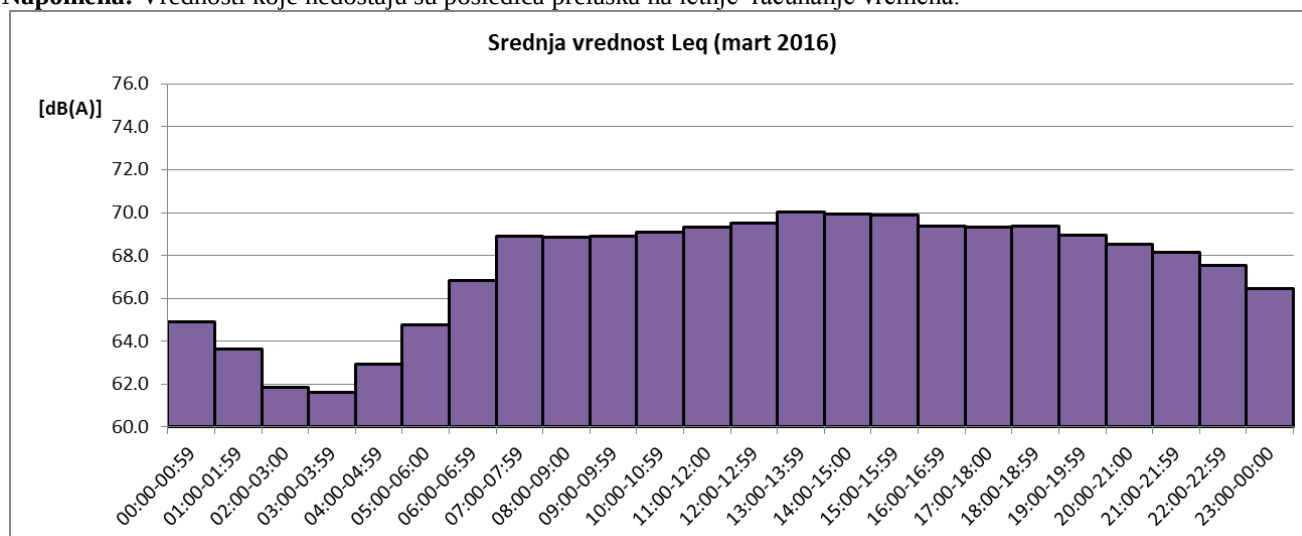
Sl. 3 Promene usrednjenih časovnih vrednosti ekvivalentnog nivoa buke u toku marta 2016 za NMT-1
