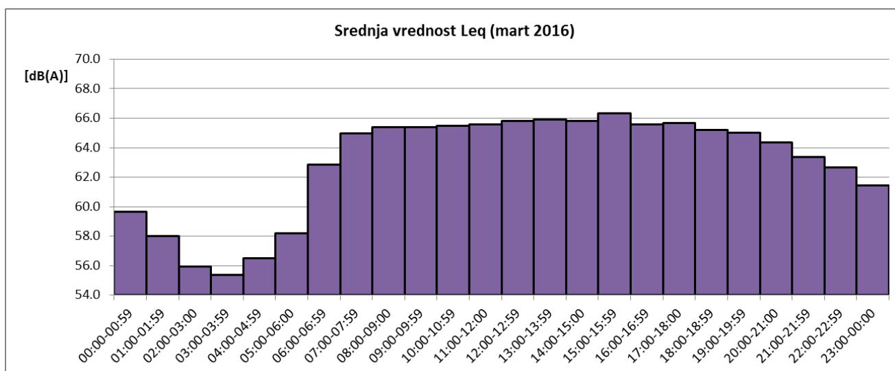
Sl. 4 Promene usrednjenih časovnih vrednosti ekvivalentnog nivoa buke u toku marta 2016 za NMT-2
