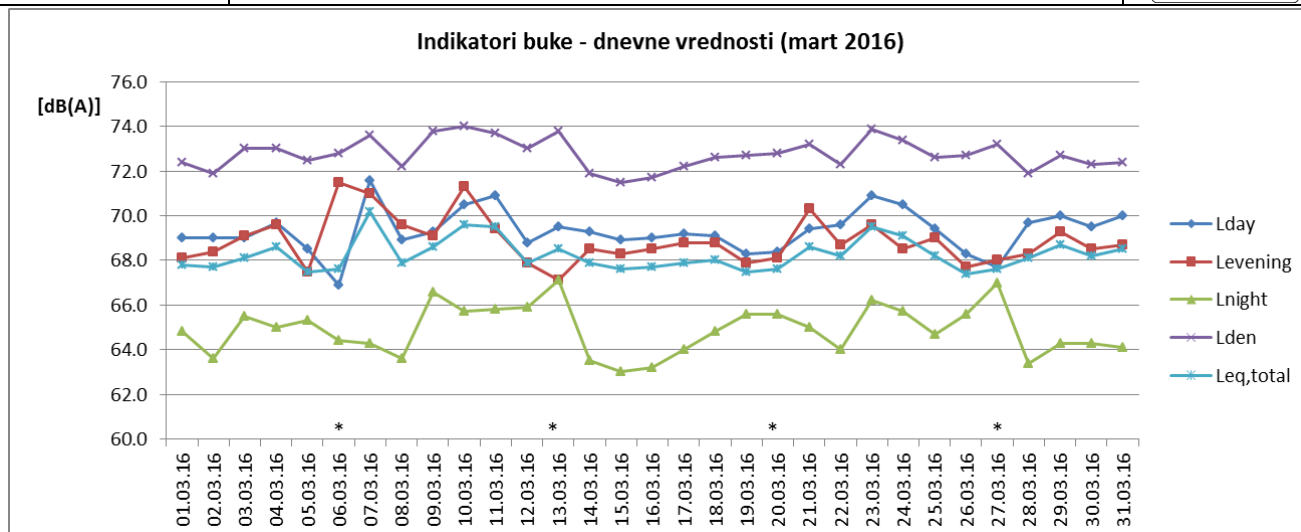
Sl. 1 Promene dnevnih vrednosti indikatora buke u toku marta 2016 za NMT-1
