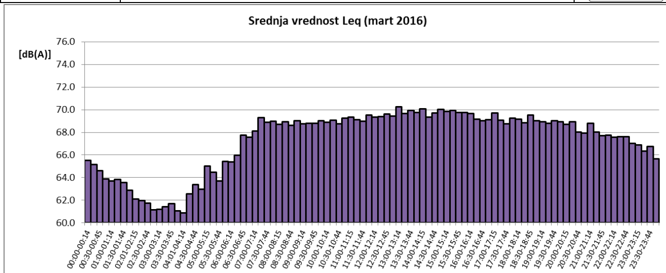
Sl. 5 Promene usrednjenih petnaestominutnih vrednosti ekvivalentnog nivoa buke u toku marta 2016 za NMT-1
