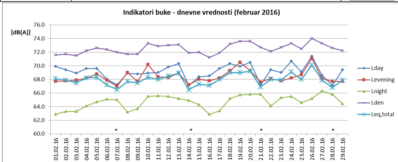
Sl. 1 Promene dnevnih vrednosti indikatora buke u toku februara 2016 za NMT-1
