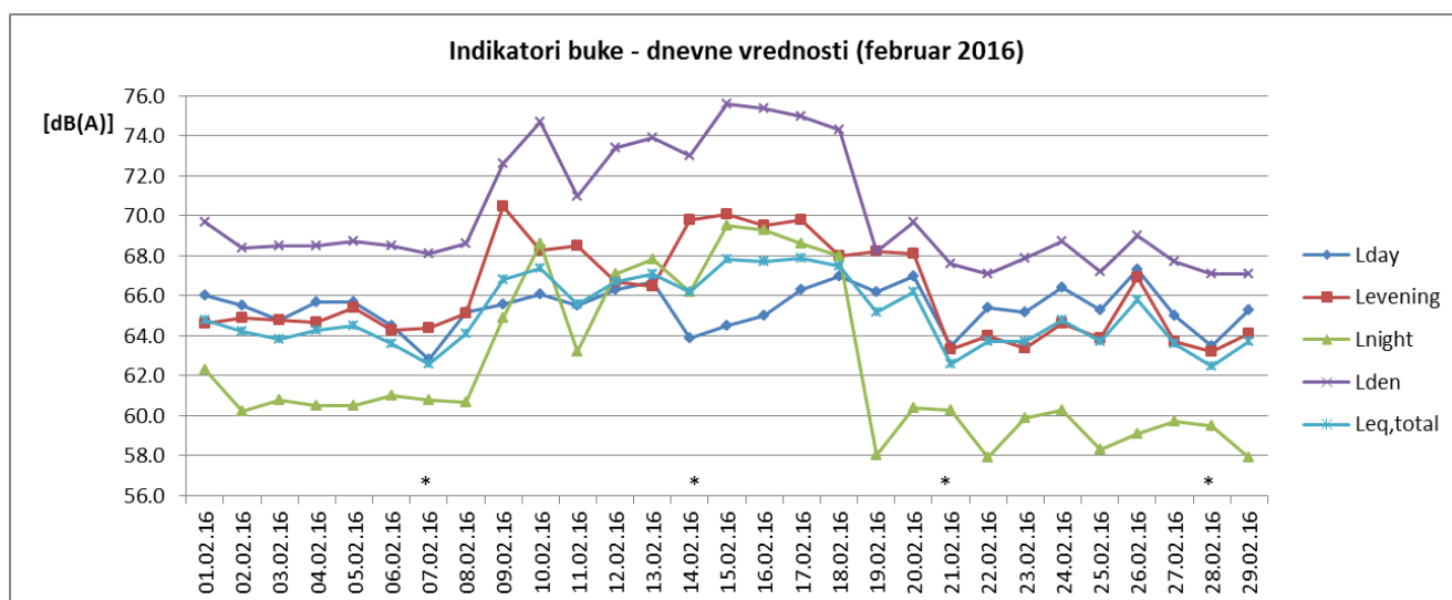
Sl. 2 Promene dnevnih vrednosti indikatora buke u toku februara 2016 za NMT-2
