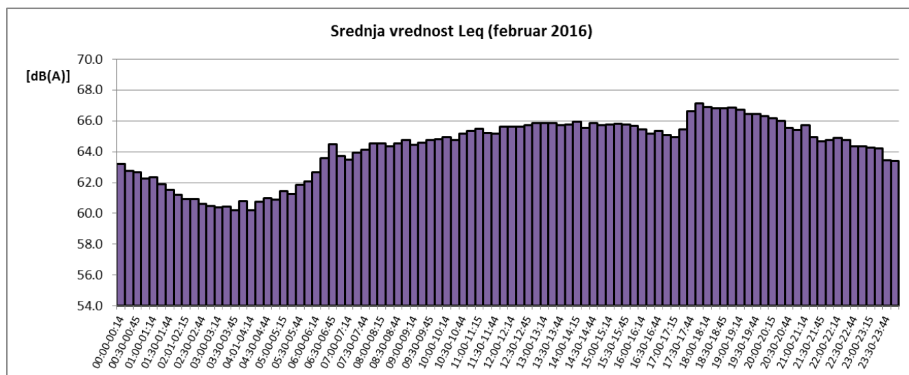
Sl. 6 Promene usrednjenih petnaestominutnih vrednosti ekvivalentnog nivoa buke u toku februara 2016 za NMT-2
