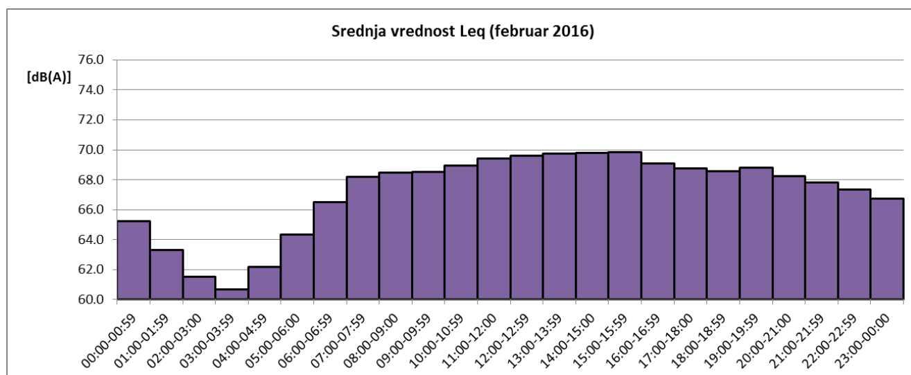
Sl. 3 Promene usrednjenih časovnih vrednosti ekvivalentnog nivoa buke u toku februara 2016 za NMT-1
