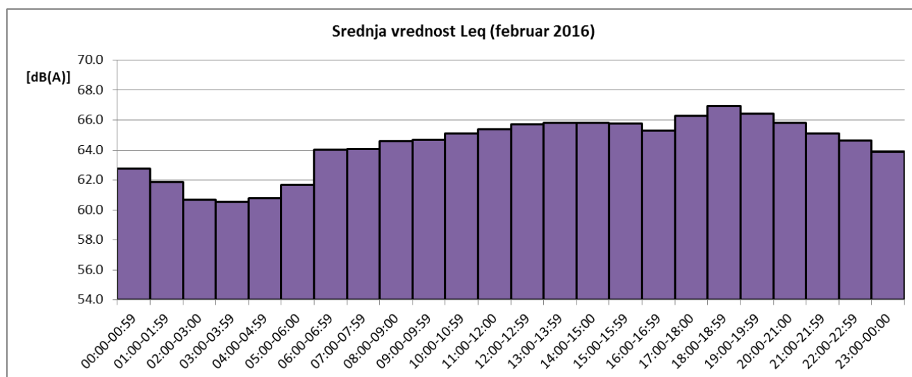
Sl. 4 Promene usrednjenih časovnih vrednosti ekvivalentnog nivoa buke u toku februara 2016 za NMT-2
