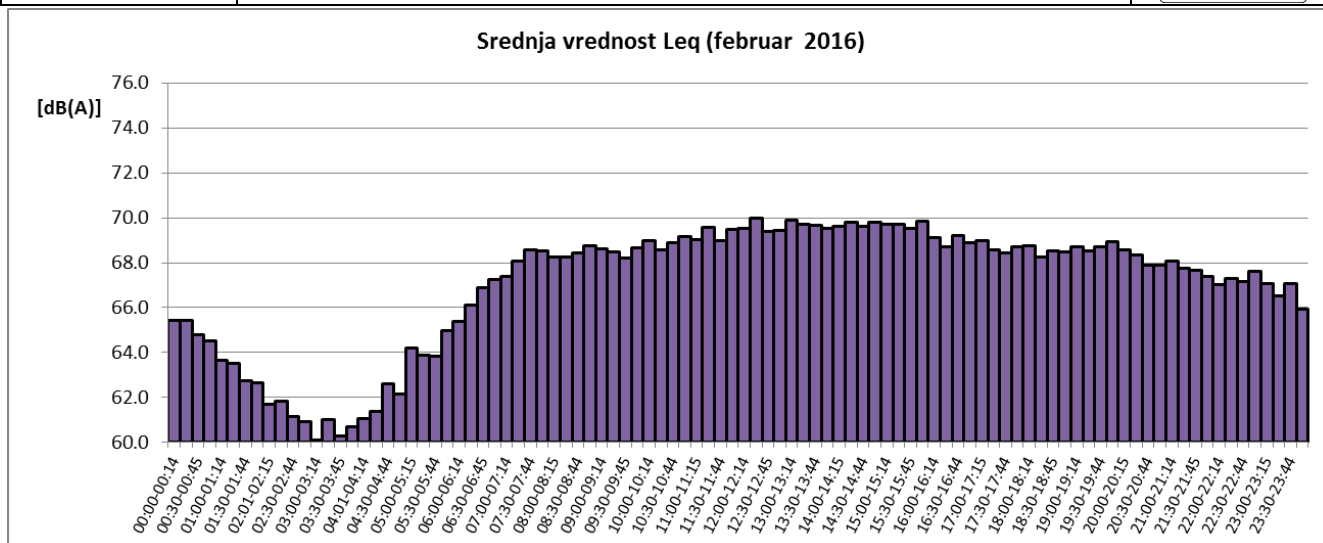
Sl. 5 Promene usrednjenih petnaestominutnih vrednosti ekvivalentnog nivoa buke u toku februara 2016 za NMT-1
