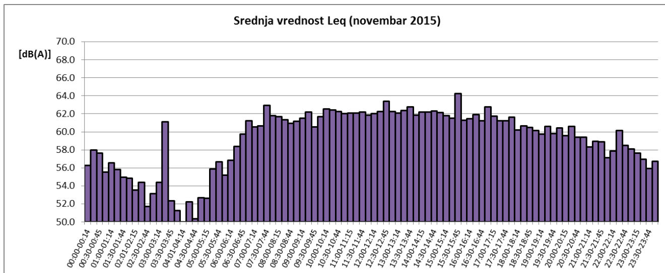
Sl. 6 Promene usrednjenih petnaestominutnih vrednosti ekvivalentnog nivoa buke u toku novembra 2015 za NMT-2
