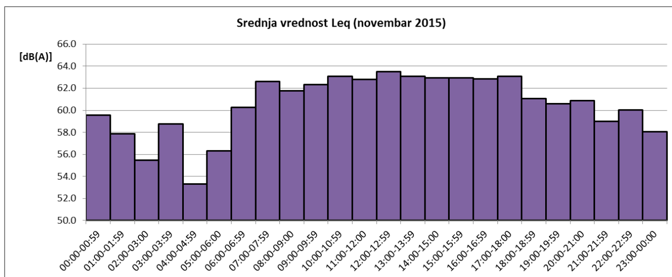
Sl. 4 Promene usrednjenih časovnih vrednosti ekvivalentnog nivoa buke u toku novembra 2015 za NMT-2
