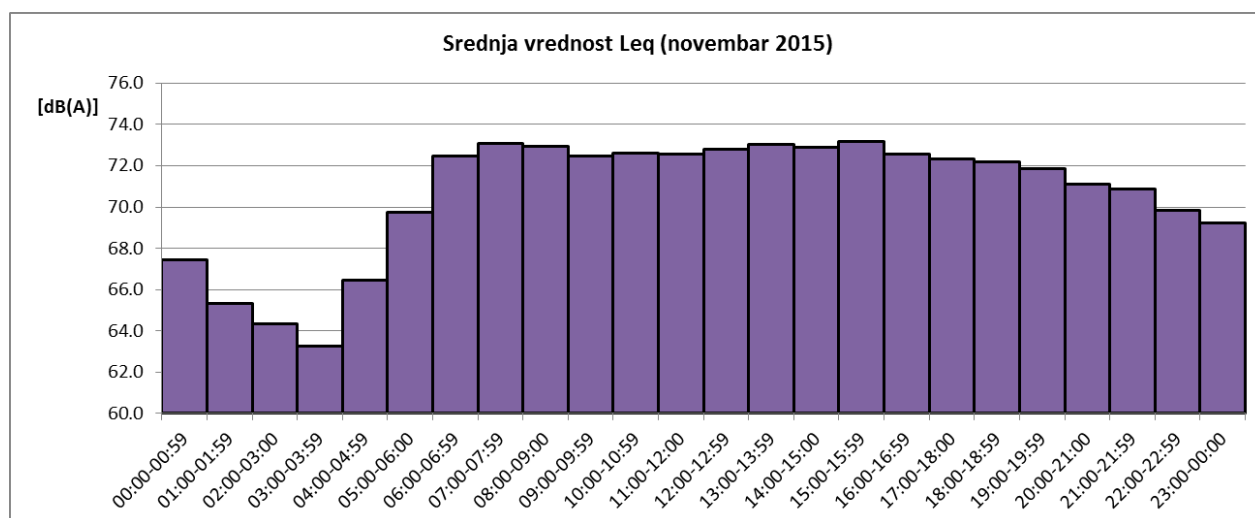
Sl. 3 Promene usrednjenih časovnih vrednosti ekvivalentnog nivoa buke u toku novembra 2015 za NMT-1
