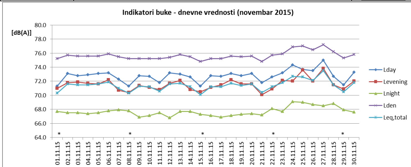
Sl. 1 Promene dnevnih vrednosti indikatora buke u toku novembra 2015 za NMT-1
