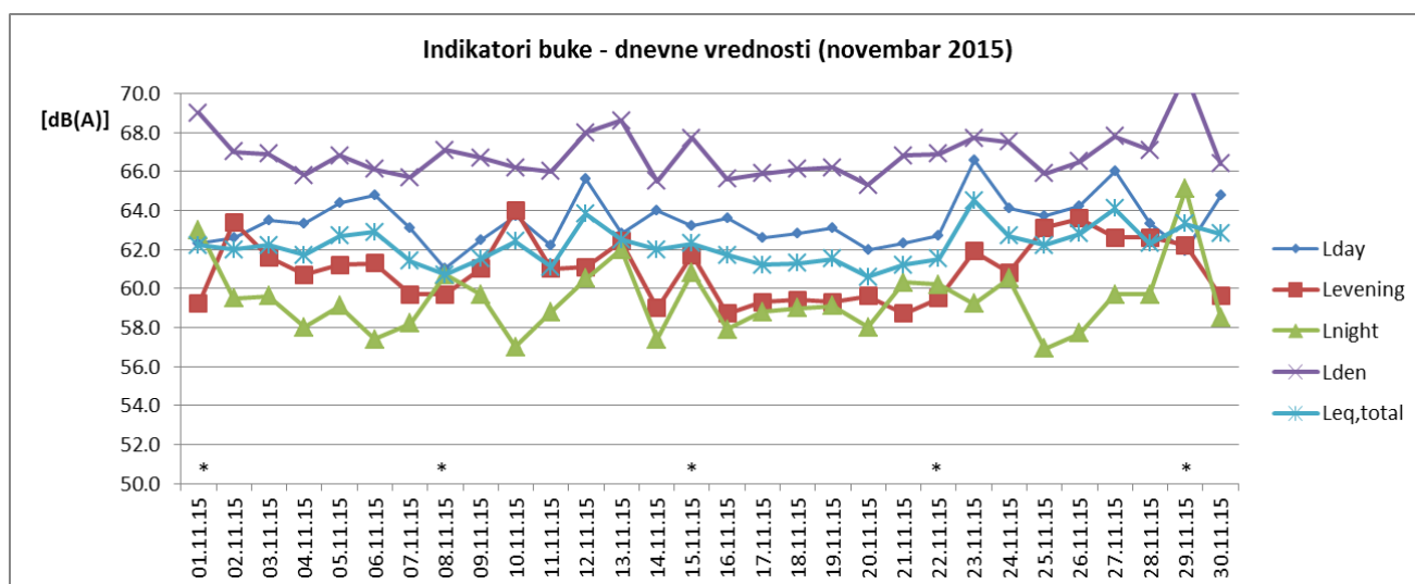
Sl. 2 Promene dnevnih vrednosti indikatora buke u toku novembra 2015 za NMT-2
