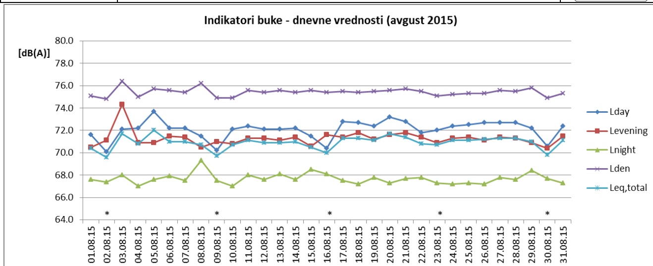
Sl. 1 Promene dnevnih vrednosti indikatora buke u toku avgusta 2015 za NMT-1
