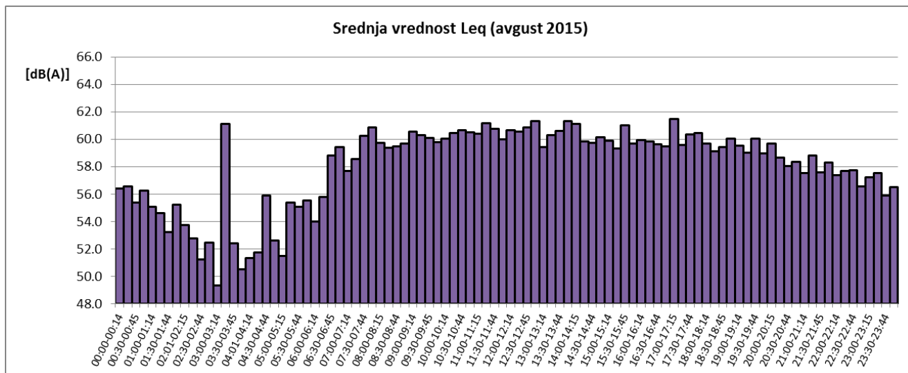
Sl. 6 Promene usrednjenih petnaestominutnih vrednosti ekvivalentnog nivoa buke u toku avgusta 2015 za NMT-2
