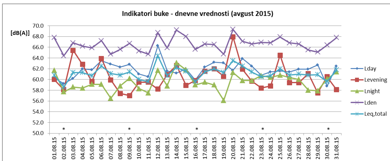
Sl. 2 Promene dnevnih vrednosti indikatora buke u toku avgusta 2015 za NMT-2
