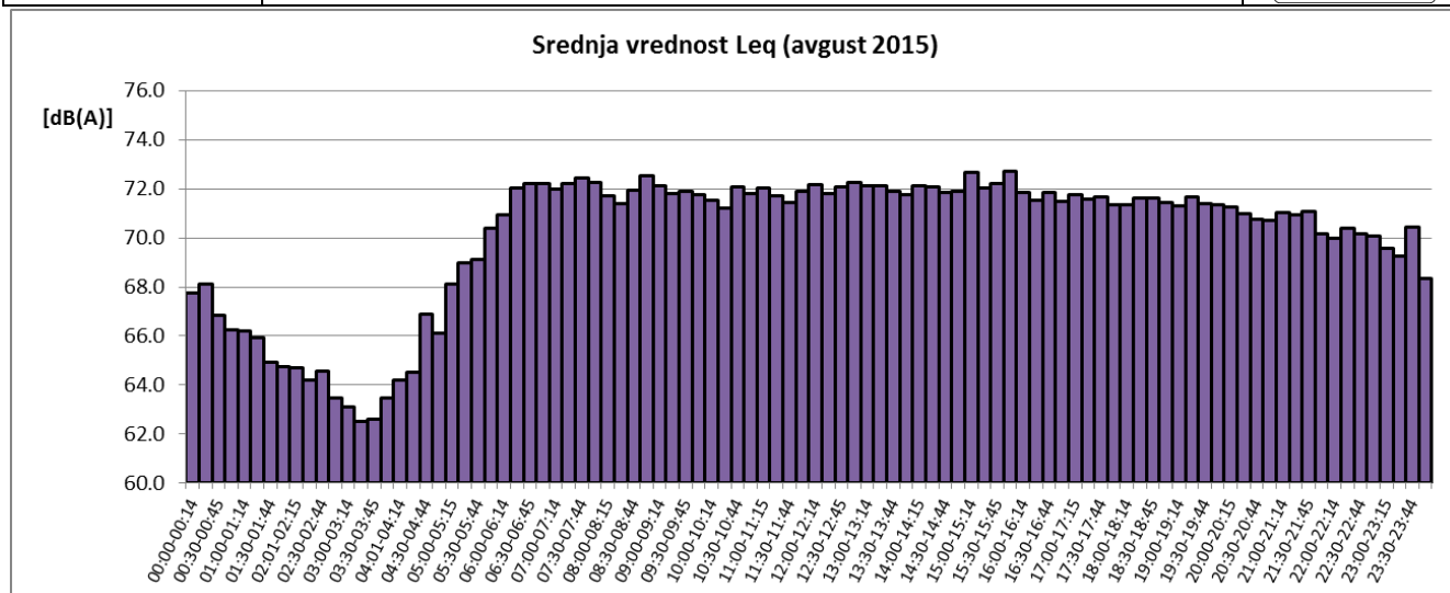
Sl. 5 Promene usrednjenih petnaestominutnih vrednosti ekvivalentnog nivoa buke u toku avgusta 2015 za NMT-1
