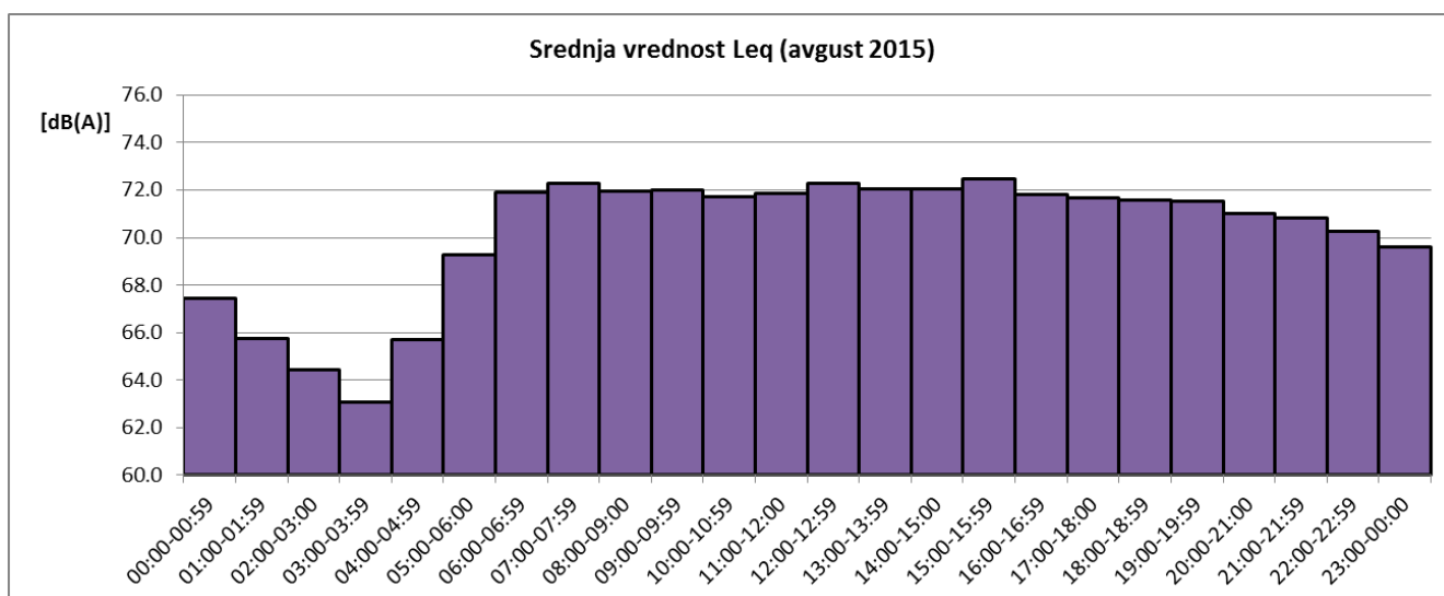
Sl. 3 Promene usrednjenih časovnih vrednosti ekvivalentnog nivoa buke u toku avgusta 2015 za NMT-1
