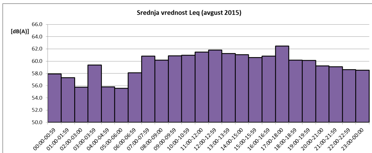
Sl. 4 Promene usrednjenih časovnih vrednosti ekvivalentnog nivoa buke u toku avgusta 2015 za NMT-2
