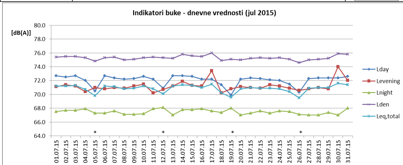
Sl. 1 Promene dnevnih vrednosti indikatora buke u toku jula 2015 za NMT-1
