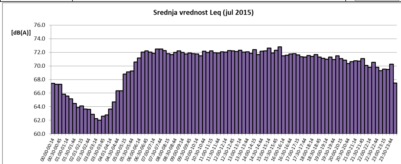
Sl. 5 Promene usrednjenih petnaestominutnih vrednosti ekvivalentnog nivoa buke u toku jula 2015 za NMT-1
