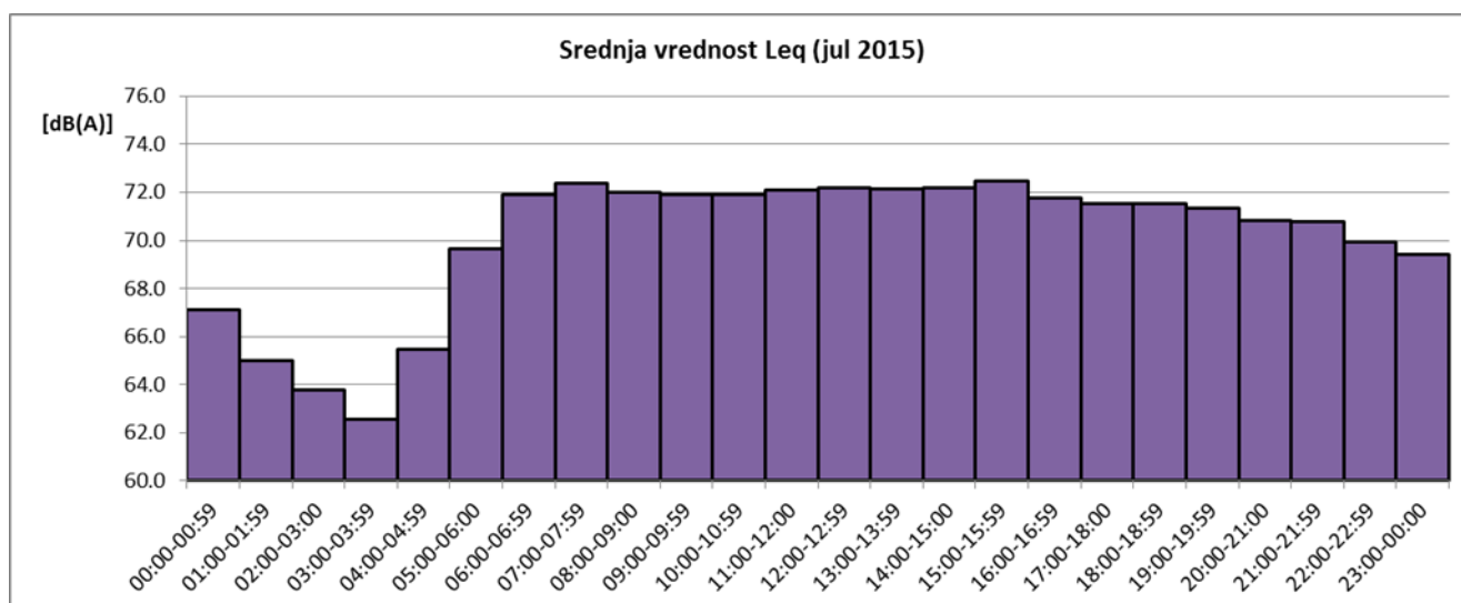
Sl. 3 Promene usrednjenih časovnih vrednosti ekvivalentnog nivoa buke u toku jula 2015 za NMT-1
