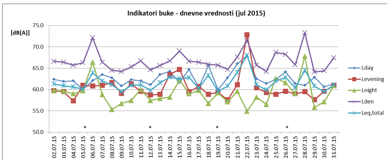
Sl. 2 Promene dnevnih vrednosti indikatora buke u toku jula 2015 za NMT-2
