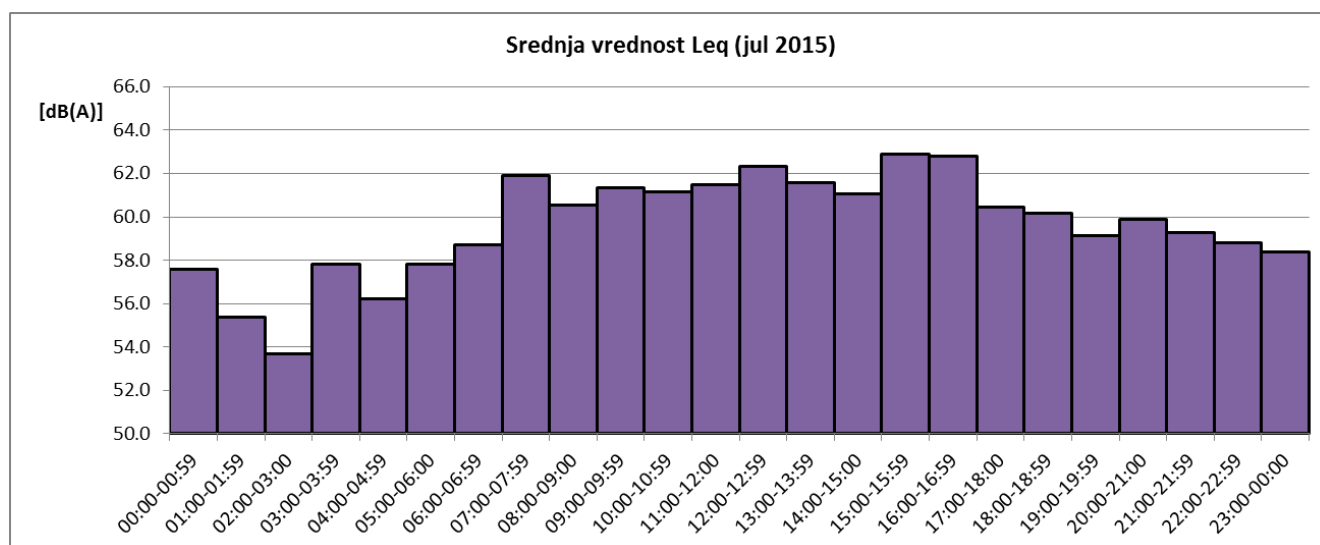
Sl. 4 Promene usrednjenih časovnih vrednosti ekvivalentnog nivoa buke u toku jula 2015 za NMT-2
