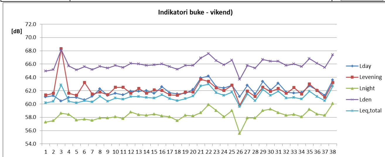
Sl. 14 Promene vikend vrednosti indikatora buke u toku 2014/2015 za NMT-2.1
