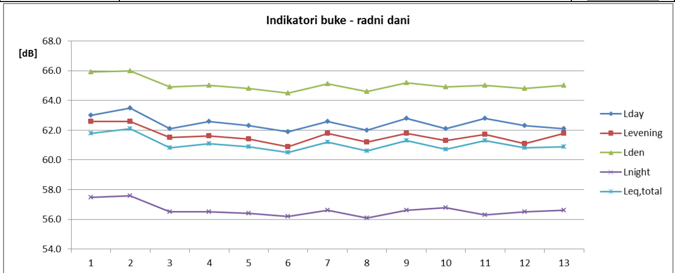
Sl. 11 Promene petodnevni (radni dani) vrednosti indikatora buke u toku 2015 za NMT-2.2
