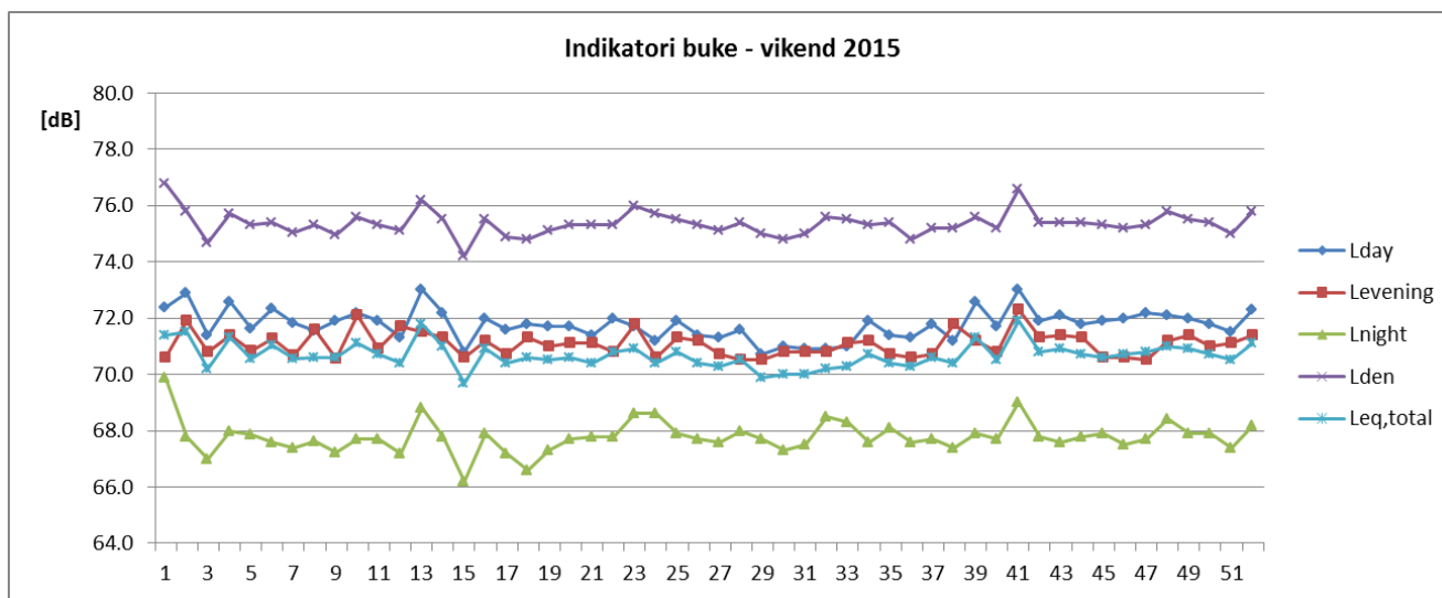
Sl. 13 Promene vikend vrednosti indikatora buke u toku 2015 za NMT-1
