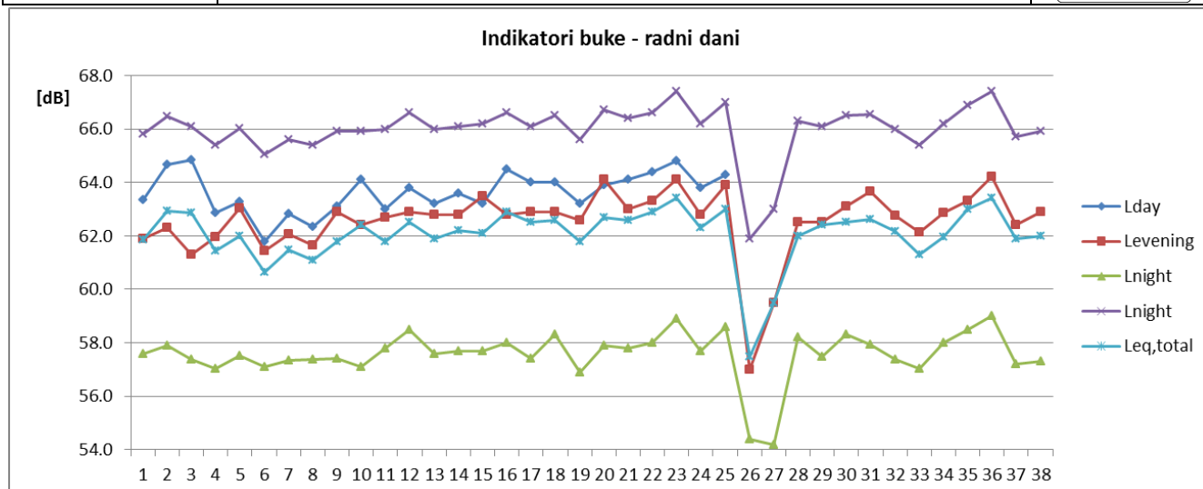
Sl. 10 Promene petodnevni (radni dani) vrednosti indikatora buke u toku 2014/2015 za NMT-2.1
