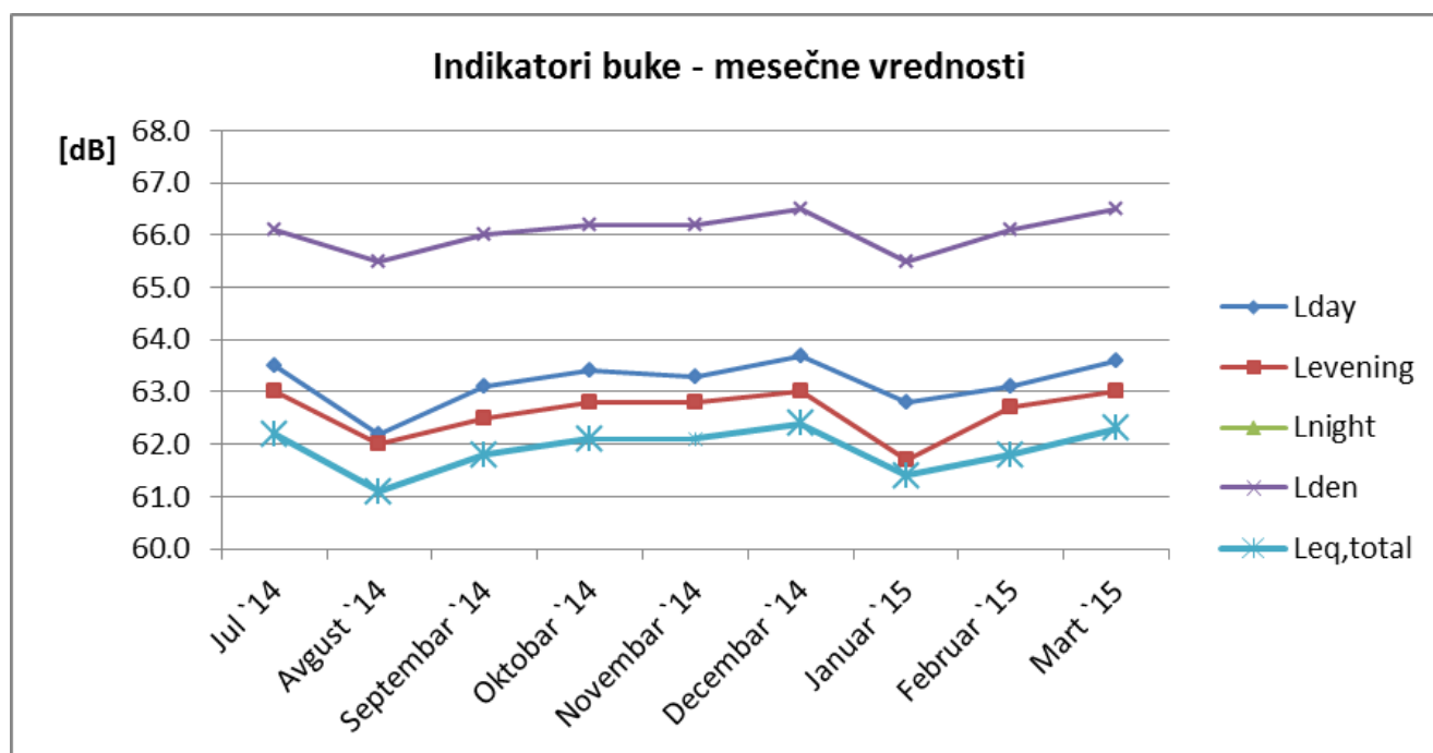
Sl. 2 Promene mesečnih vrednosti indikatora buke u toku 2014/2015 za NMT-2.1
