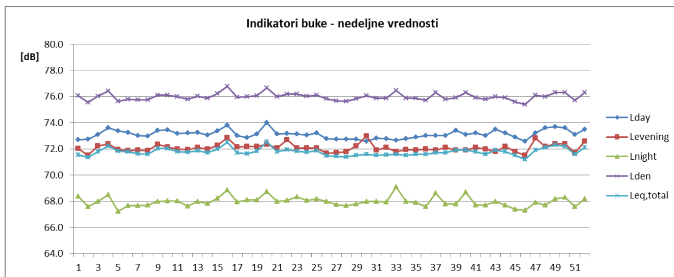
Sl. 5 Promene nedeljnih vrednosti indikatora buke u toku 2015 za NMT-1
