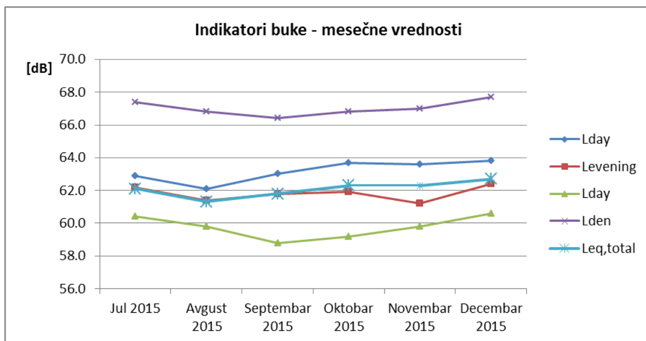
Sl. 4 Promene mesečnih vrednosti indikatora buke u toku 2015 za NMT-2.3
