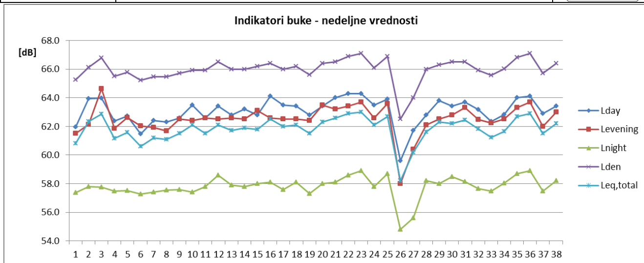
Sl. 6 Promene nedeljnih vrednosti indikatora buke u toku 2014/2015 za NMT-2.1
