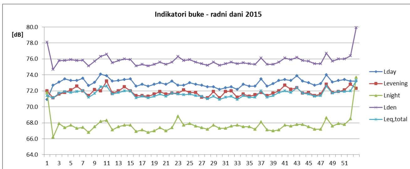
Sl. 9 Promene petodnevni (radni dani) vrednosti indikatora buke u toku 2015 za NMT-1
