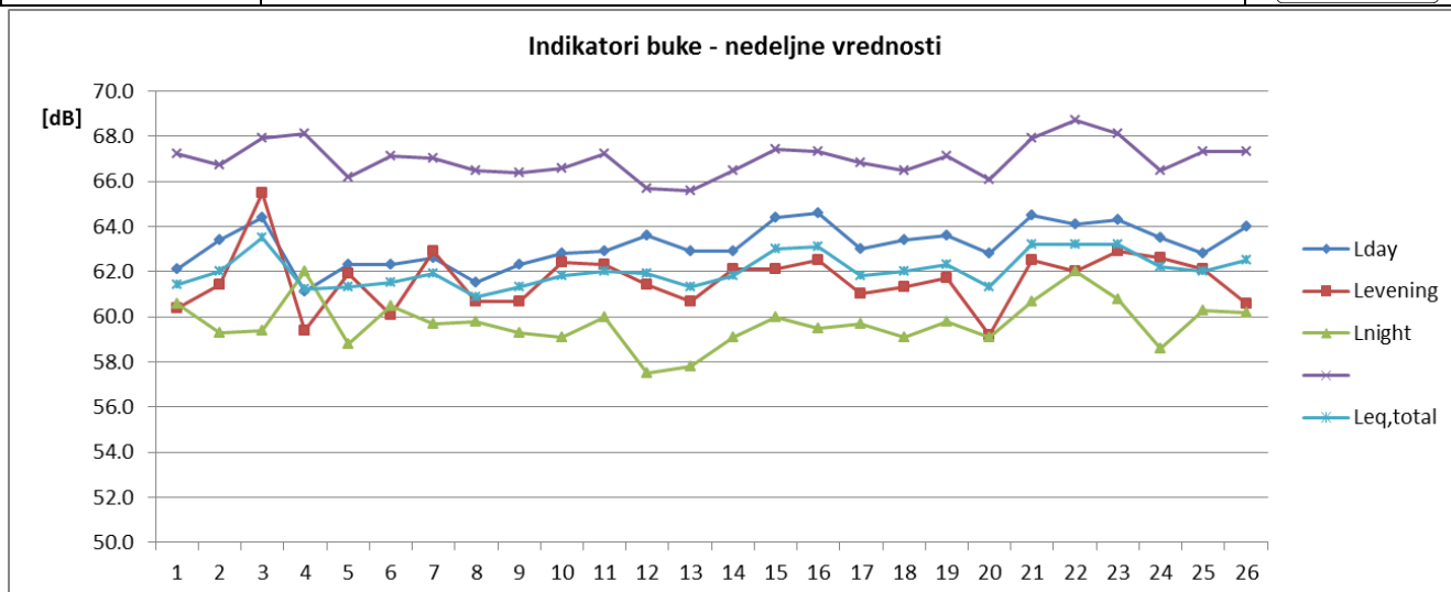
Sl. 8 Promene nedeljnih vrednosti indikatora buke u toku 2015 za NMT-2.3
