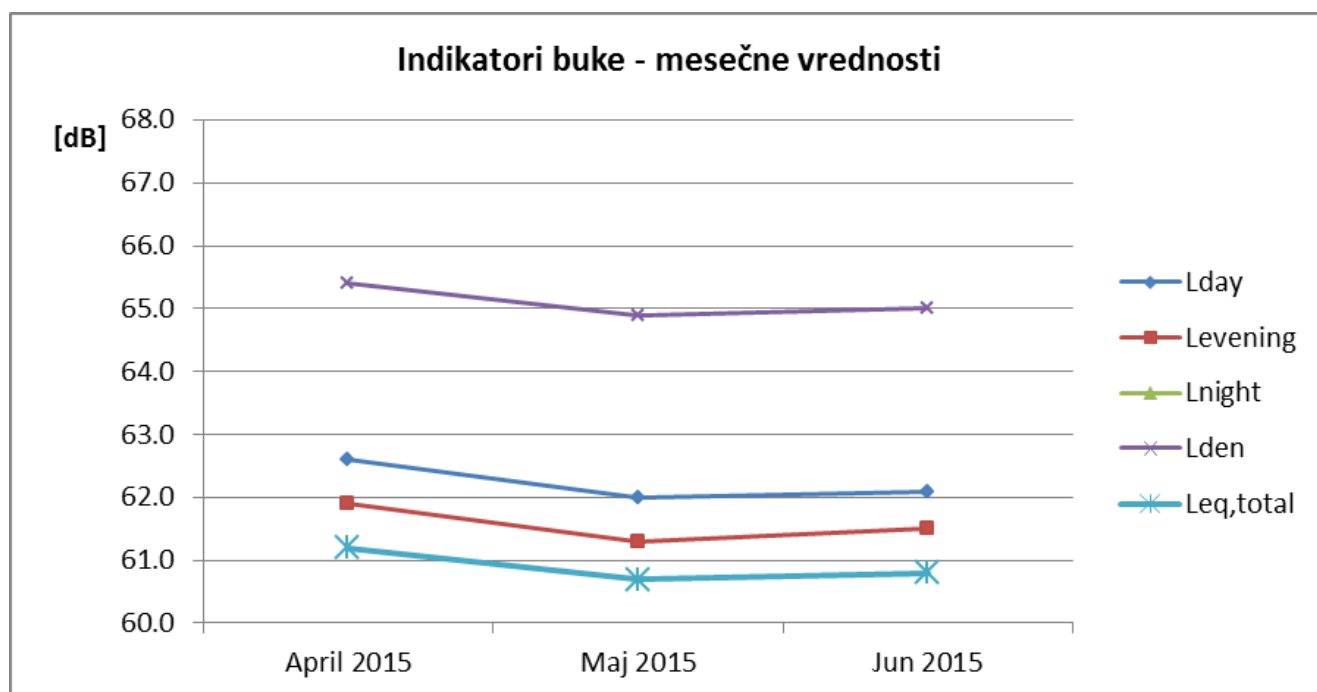
Sl. 3 Promene mesečnih vrednosti indikatora buke u toku 2015 za NMT-2.2
