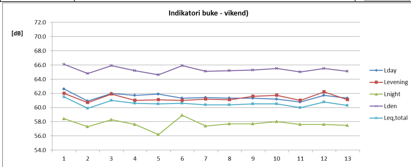
Sl. 15 Promene vikend vrednosti indikatora buke u toku 2015 za NMT-2.2
