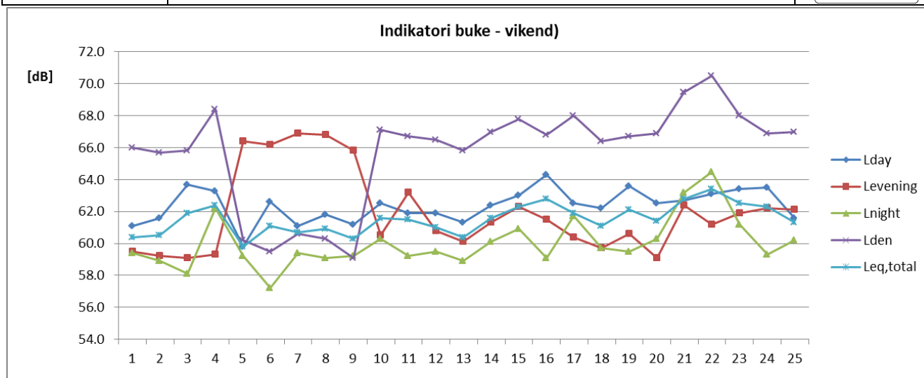
Sl. 16 Promene vikend vrednosti indikatora buke u toku 2015 za NMT-2.3
