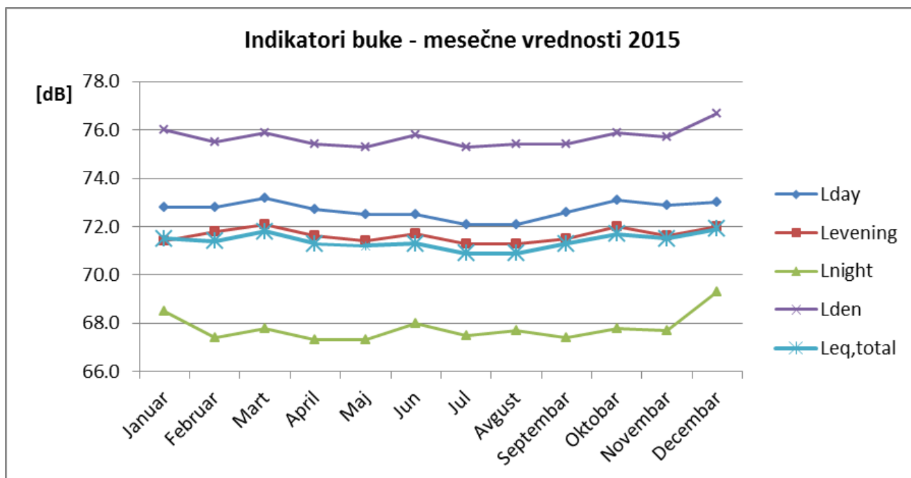
Sl. 1 Promene mesečnih vrednosti indikatora buke u toku 2015 za NMT-1
