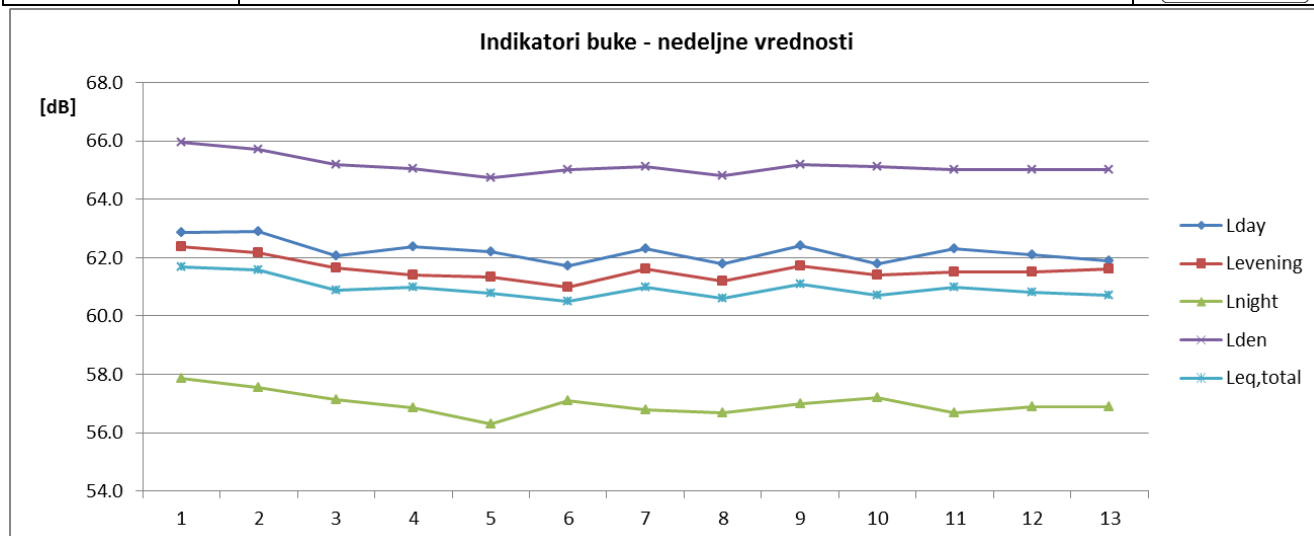
Sl. 7 Promene nedeljnih vrednosti indikatora buke u toku 2015 za NMT-2.2
