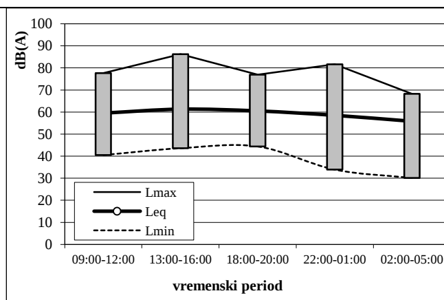
SI. 3.6 Dinamika izmerenog nivoa buke - merno mesto 8.1
