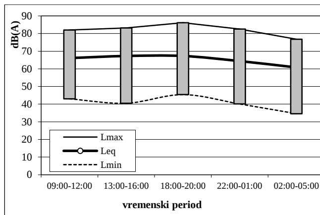
SI. 3.2 Dinamika izmerenog nivoa buke - merno mesto 4.1
