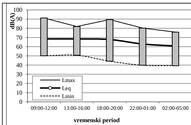
SI. 3.5 Dinamika izmerenog nivoa buke - merno mesto 7.1
