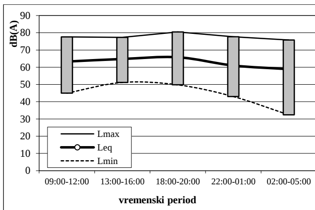
SI. 3.1 Dinamika izmerenog nivoa buke - merno mesto 3.1
