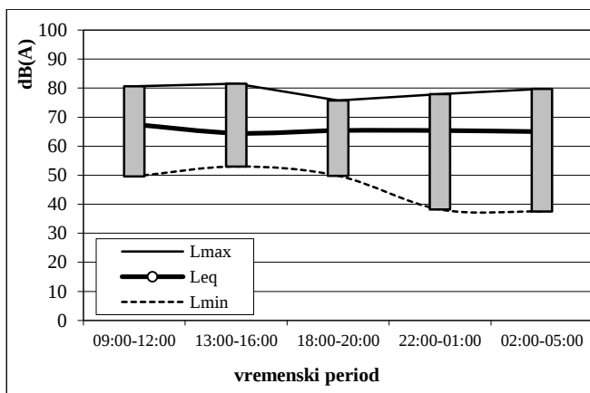
SI. 3.3 Dinamika izmerenog nivoa buke - merno mesto 5.1
