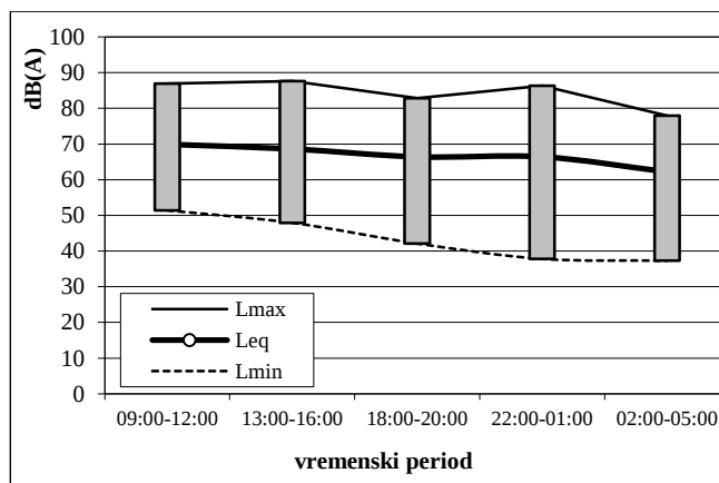
SI. 3.4 Dinamika izmerenog nivoa buke - merno mesto 6.1
