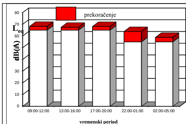
Sl. 4.5 Prekoračenje granične vrednosti - merno mesto 7.3
