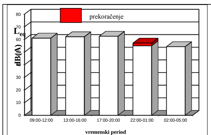
Sl. 4.9 Prekoračenje granične vrednosti - merno mesto 11.3
