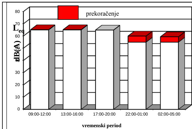
Sl. 4.1 Prekoračenje granične vrednosti - merno mesto 3.3
