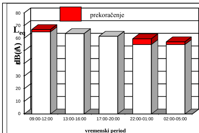
Sl. 4.3 Prekoračenje granične vrednosti - merno mesto 5.3
