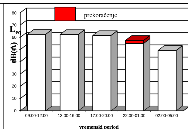
Sl. 4.8 Prekoračenje granične vrednosti - merno mesto 10.3
