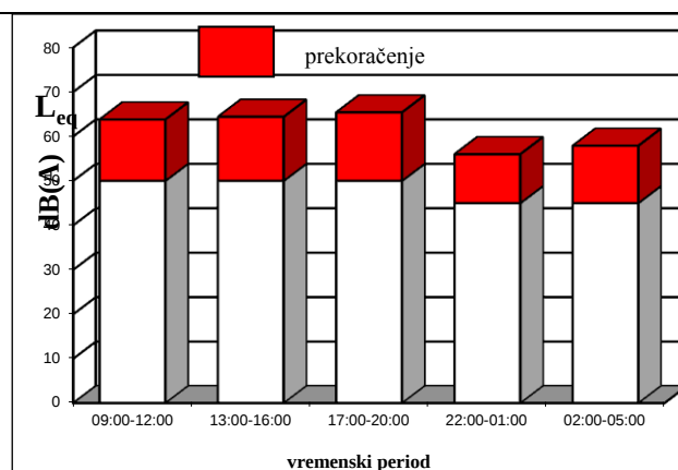
Sl. 4.6 Prekoračenje granične vrednosti - merno mesto 8.3
