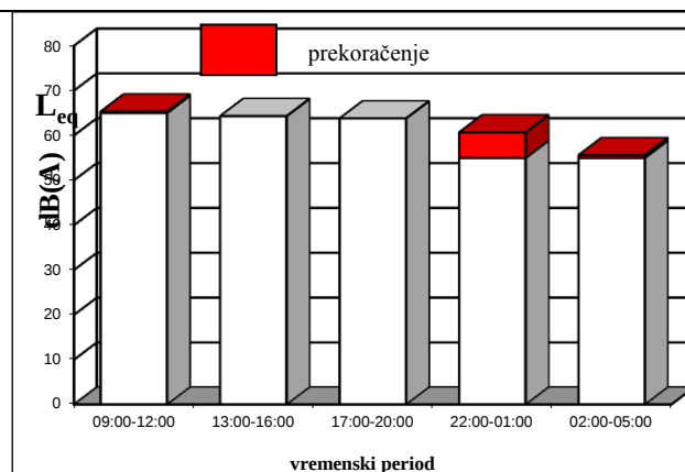
Sl. 4.4 Prekoračenje granične vrednosti - merno mesto 6.3
