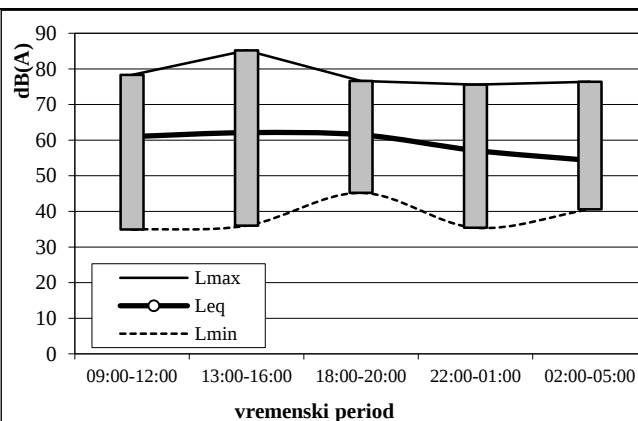
Sl. 3.9 Dinamika izmerenog nivoa buke - merno mesto 11.3
