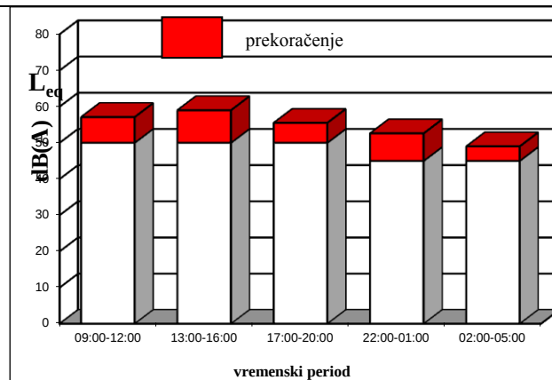
Sl. 4.2 Prekoračenje granične vrednosti - merno mesto 4.3
