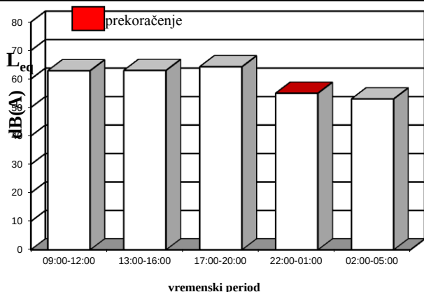
Sl. 4.7 Prekoračenje granične vrednosti - merno mesto 9.2
