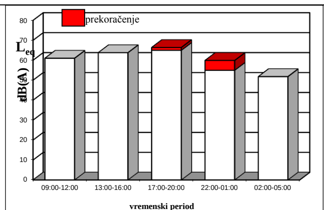
Sl. 4.4 Prekoračenje granične vrednosti - merno mesto 6.2
