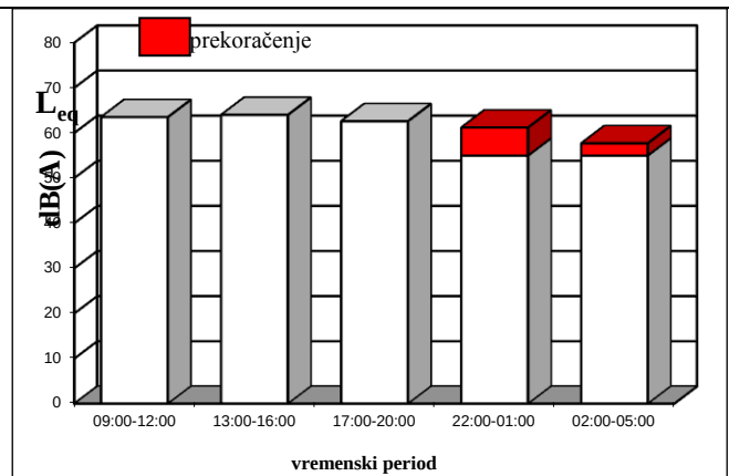
Sl. 4.2 Prekoračenje granične vrednosti - merno mesto 4.2
