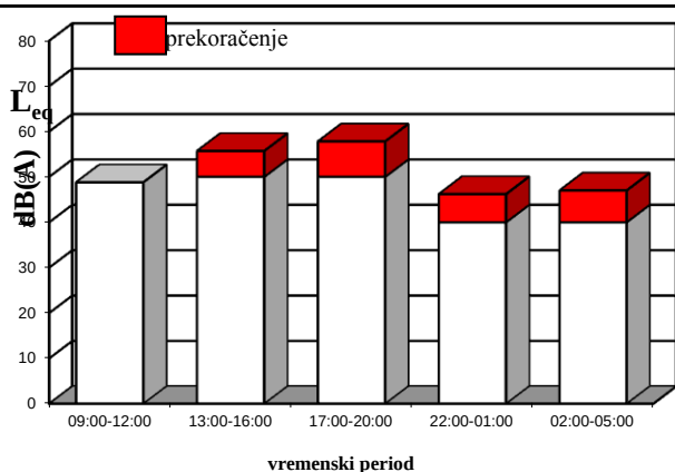
Sl. 4.9 Prekoračenje granične vrednosti - merno mesto 11.2
