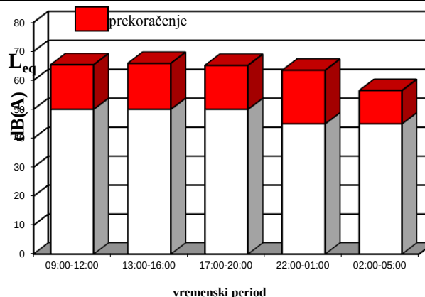
Sl. 4.8 Prekoračenje granične vrednosti - merno mesto 10.2
