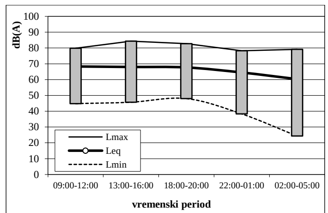
Sl. 3.4 Dinamika izmerenog nivoa buke - merno mesto 6.1
