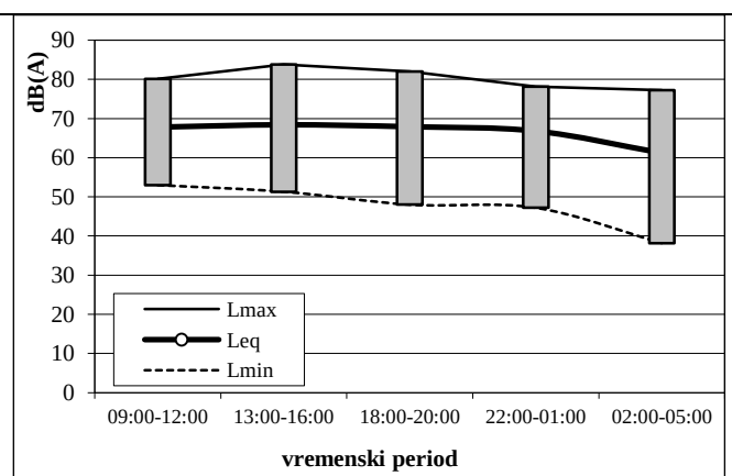
Sl. 3.6 Dinamika izmerenog nivoa buke - merno mesto 8.1
