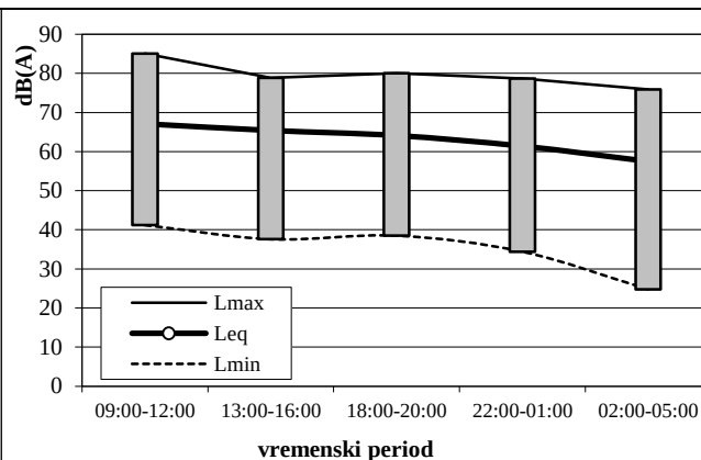
Sl. 3.9 Dinamika izmerenog nivoa buke - merno mesto 11.1
