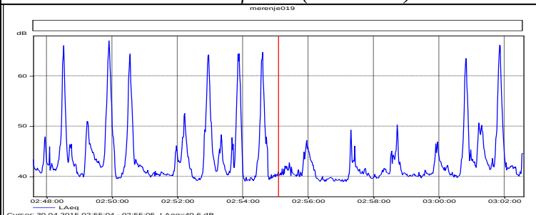
Sl. P.1.5 Profil buke (02:47-03:02)
