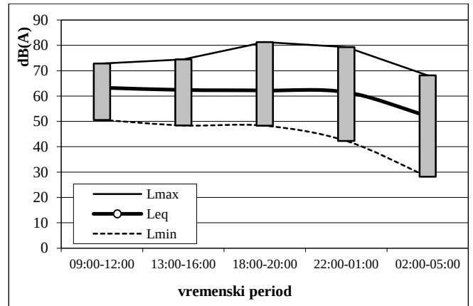
Sl. 3.2 Dinamika izmerenog nivoa buke - merno mesto 4.1
