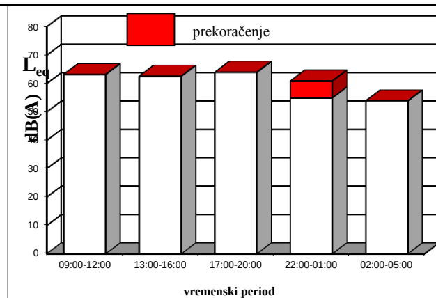
Sl. 4.2 Prekoračenje granične vrednosti - merno mesto 4.1
