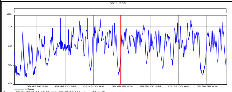
Sl. P.7.1 Profil buke (09:40-09:55)
