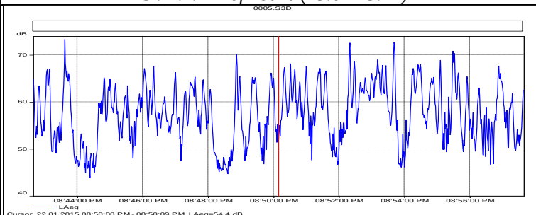
Sl. P.7.3 Profil buke (20:43-20:58)
