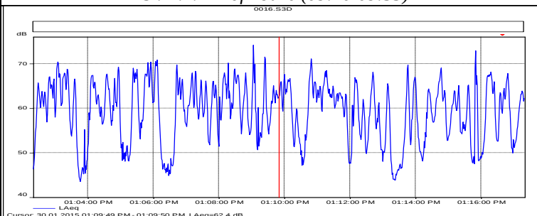
Sl. P.7.2 Profil buke (13:02-13:17)
